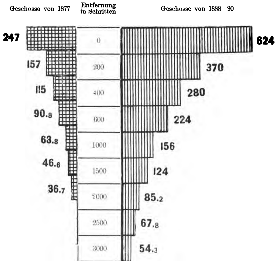
Lebendige Kraft auf den Quadratcentimeter des Geschossumfanges im Augenblick des Schusses in Meter-Kilogrammen.
