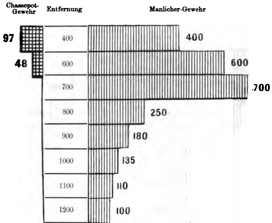
Bestrichener Raum beim Schiessen auf Kavallerie (Höhe 2 Meter 70 Centimeter).
