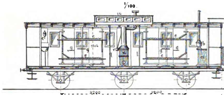
a. Küchenschrank — b. Theemaschine mit beweglicher Röhre — c. Waschtisch — e. Hängebetten — g. Tische — k. Ofen — l. spanische Wand — n. Laterne.
