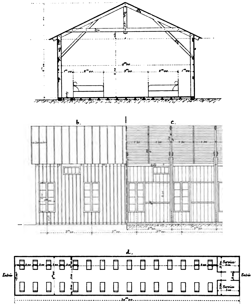
a. Querschnitt — b. Höhe — c. Längsschnitt — d. Plan.
