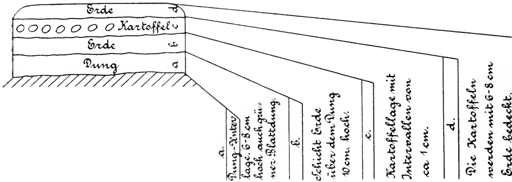
Fig. 2. Querschnitt eines fertigen Beetes.
