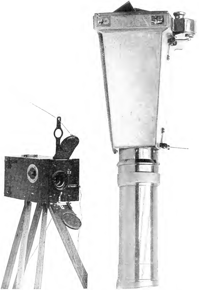
Der von mir anfänglich benutzte Nachtapparat ohne Schließverschluss, der später auf Grund zweier von mir unternommenen Reisen nach Ostafrika verbessert und durch den Goerz = Schilling = Nachtapparat ersetzt wurde und ein Tele = Apparat, wie er in der Goerzischen Optischen Anstalt in Friedenau bei Berlin hergestellt wird.
