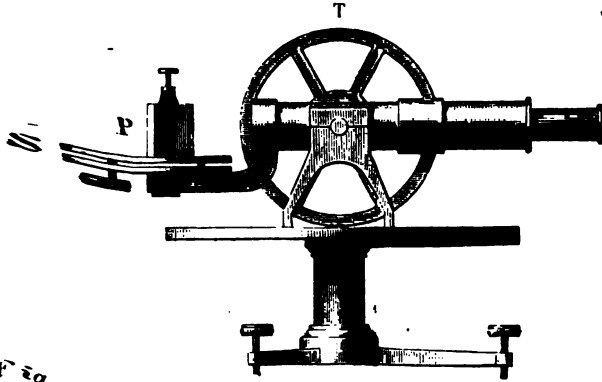
Fig. 2. — Instrument de Fraunhofer, vu de face. T, théodolite. S, disque mobile autour d'un axe vertical et placé devant l'objectif du théodolite. P, prisme en flint-glass.
