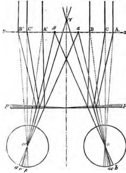
Fig. 19. — Stéréoscope par réfraction de sir D. Brewster : effet pseudo-stéréoscopique (Giraud-Teulon).
