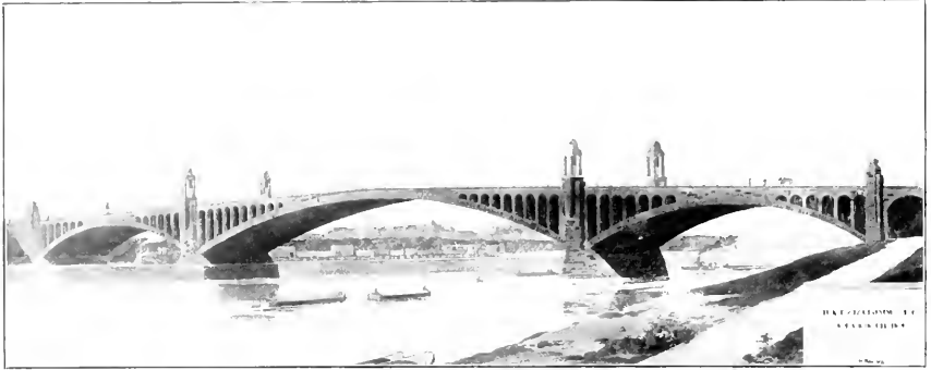
Entwürfe für die II. Neckar-Brücke in Mannheim. Variante.
