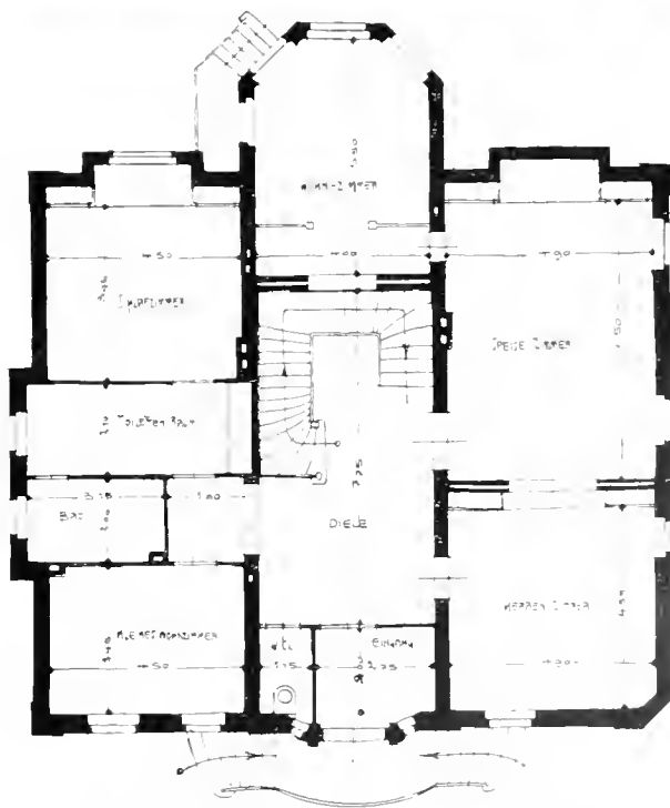
GRUNDRISS DES ERDGESCHOßES DES HAUSES KUNHENN—ESSEN.
