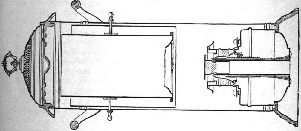
Längsschnitt.
