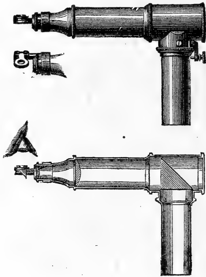
Fig. 87. — Chambre claire d'Oberhaeuser (construite par MM. Bèzu, Hausser et C ie ).
