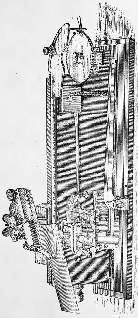
Microtome à levier, de Hansen, construit par M. Em. Deyrolle, à Paris.
