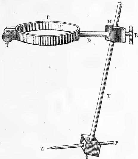
[Fig. 74. — Doigt mécanique.]
