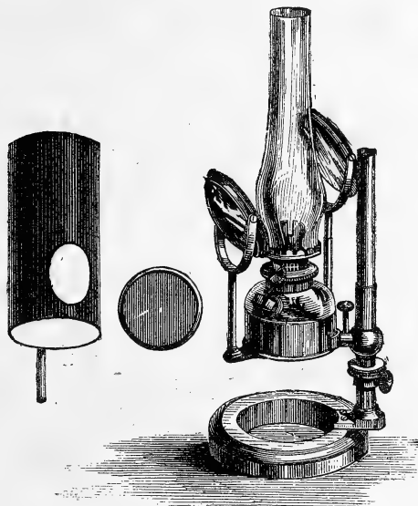
Fig. 89. — Lampe de Swift.
