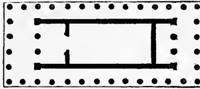
(4) PERIPTEROS.
