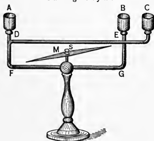
Fig. 265. Ampère's Apparatus.
