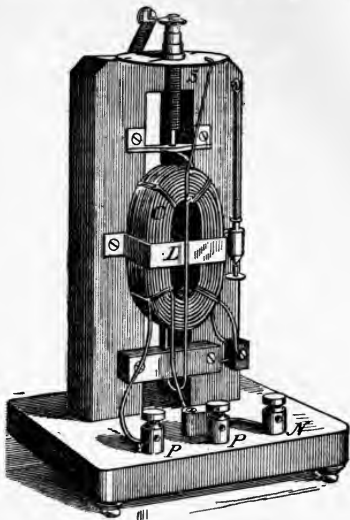
Fig. 224. Siemens' Electro-Dynamometer.
