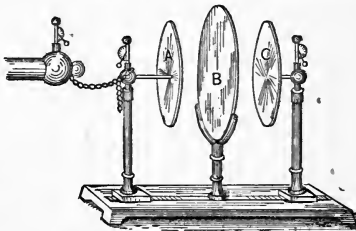
Fig. 167. Aepinus Air Condenser.
