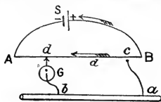
Fig. 451. Potentiometer.
