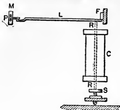
Fig. 383. Bidwell Apparatus.
