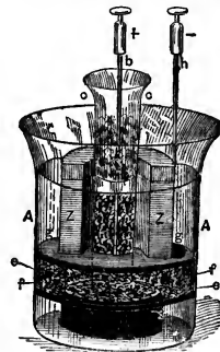
Fig. 113. Siemens-Halske Cell.
