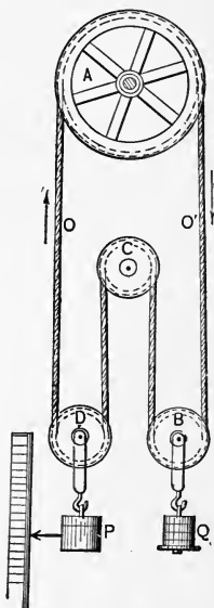
Fig. 223. Parsons' Dynamometer.
