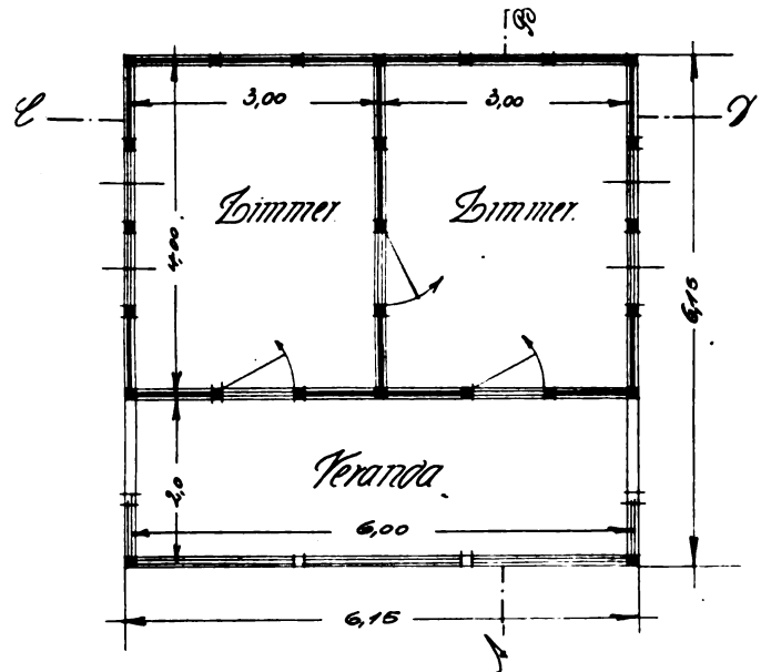
Grundriß zu obenstehendem Gartenhaus.
