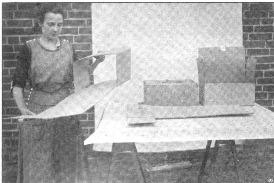
Postkarton postfertig verpackt, daneben leer und offen mit den seitlich eingelegten Verstärkungspappen, davor ein Karton wie er dem Ballen entnommen wird, rechts Veranschaulichung wie er zusammenzufügen ist.
