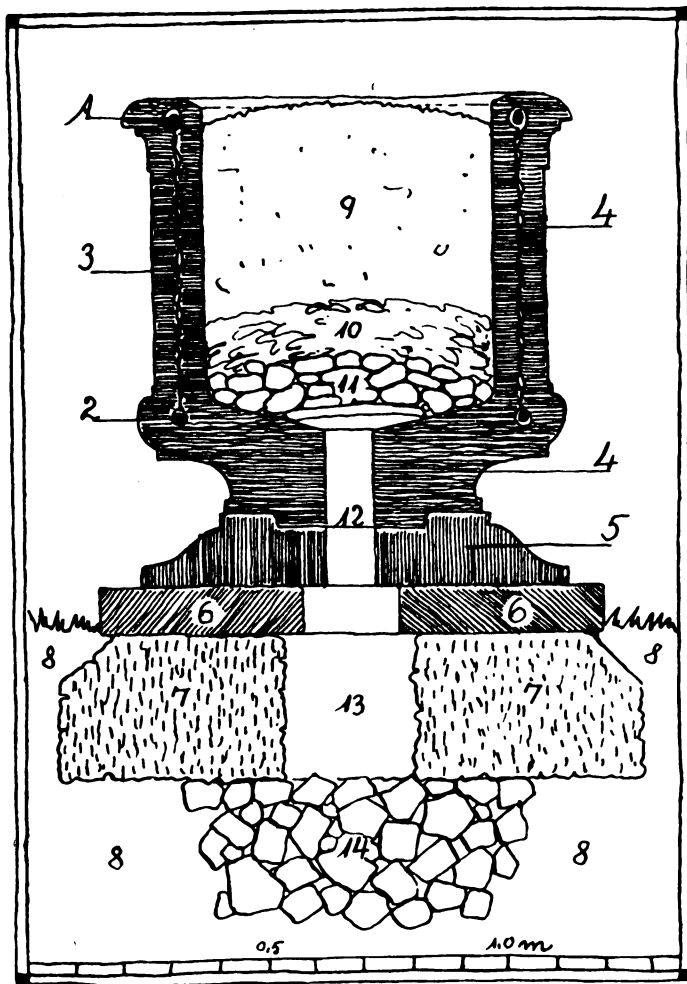
Vasenquerschnitt. 1 oberer Eisenring, 2 unterer Eisenring, 3 Drahtnetzeinlage, 4 Oberteil, 5 Fuß, 6 Sockelstufe, 7 Betonfundament, 8 Erdboden, 9 Erdfüllung, 10 grobe Düngererde, 11 Ziegelbrocken, 12 und 13 Wasserschlacht, 14 Steine (Versickerung).
