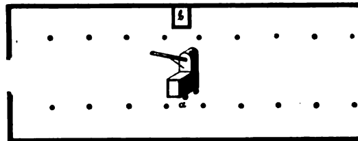
Grundriß zum hölzernen Pomeranzenhaus. a fahrbarer Ofen, b Schornstein.
