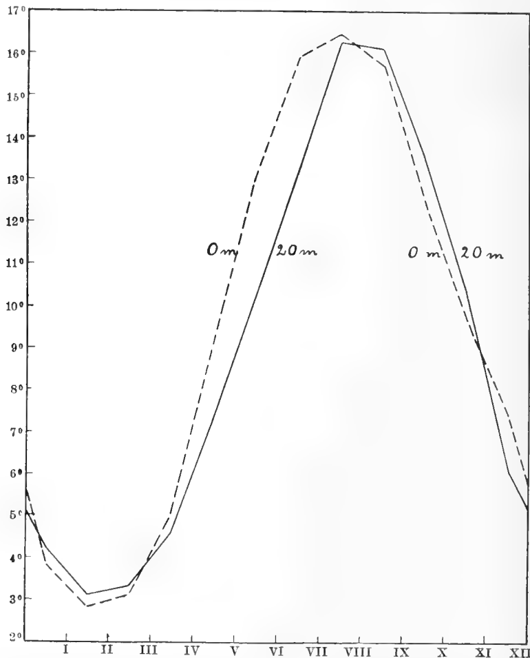
Fig. 11. Durchschnittliche Temperaturen in den einzelnen Monaten an der Oberfläche und in 20 m Tiefe bei Helgoland.
