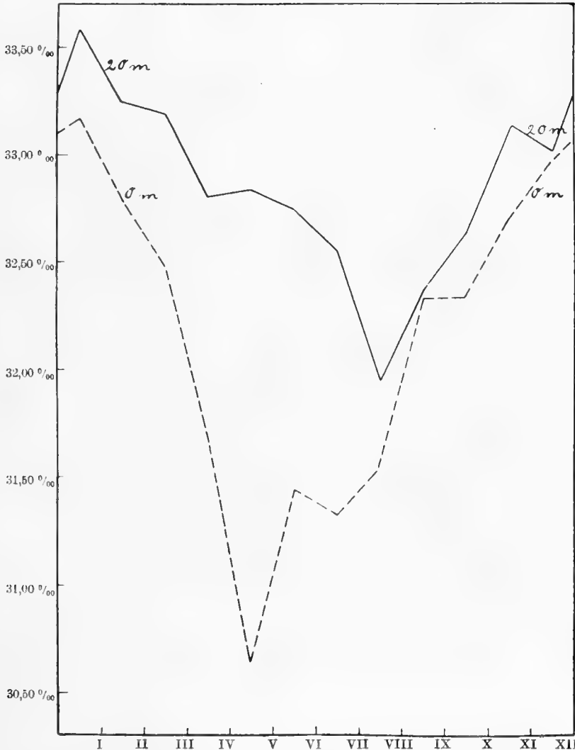
Fig. 10. Durchschnittliche Salzgehalte in den einzelnen Monaten an der Oberfläche und in 20 m Tiefe bei Helgoland.
