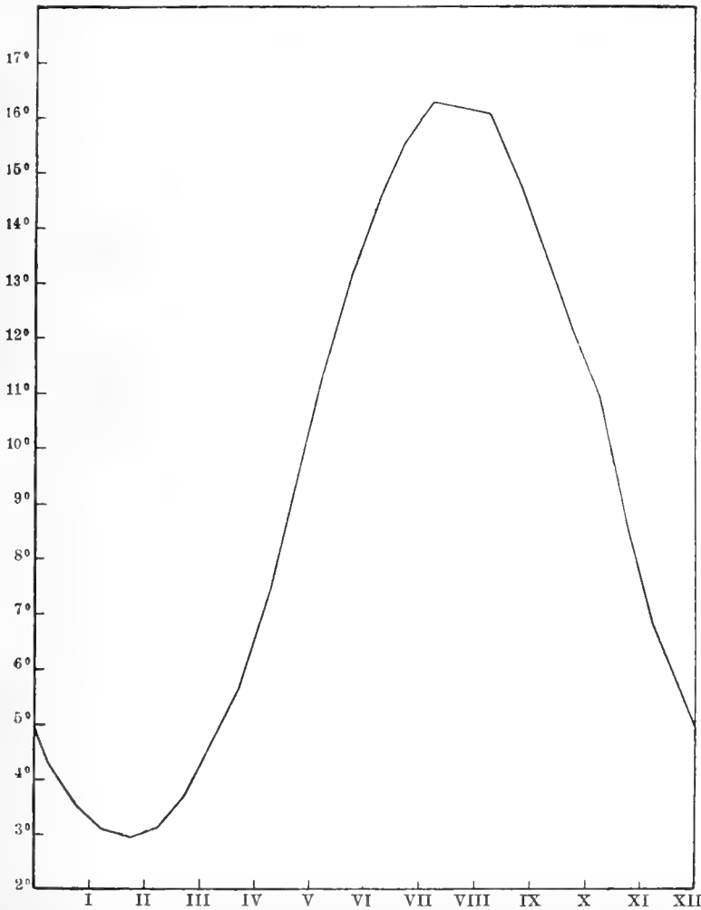
Fig. 12. Temperaturen in 14tägigen Mitteln an der Oberfläche im Strom zwischen Helgoland und Düne nach täglichen Beobachtungen vom 1. Januar 1902 bis 31. März 1907.
