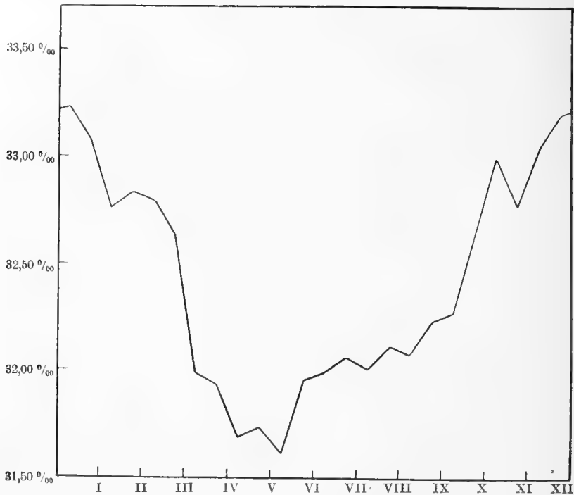
Fig. 13. Salzgehalte in 14tägigen Mitteln an der Oberfläche im Strom zwischen Helgoland und der Düne nach täglichen Beobachtungen vom 1. Januar 1902 bis 31. Dezember 1906.
