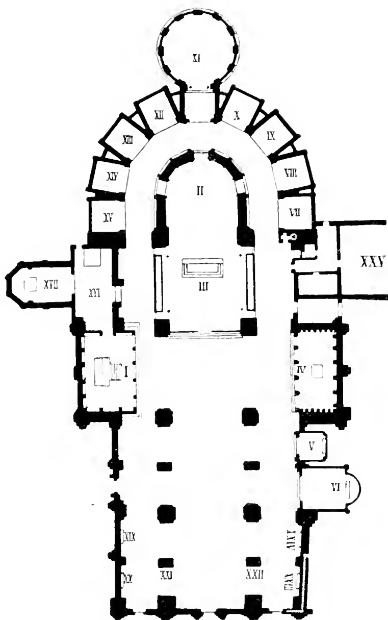
GRUNDRISS DER BASILIKA DEL SANTO IN PADUA
