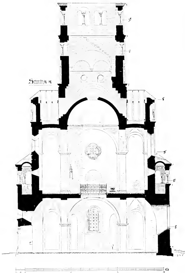
QUERSCHNITT DER KIRCHE IN SCHWARZ-RHEINDORF Mit Genehmigung des Provinzialkonservators der Rheinprovinz
