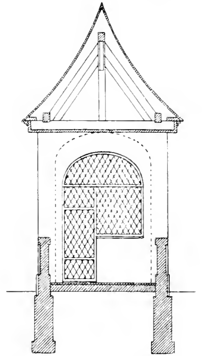
H. Grassel Kapelle, Querschnitt
