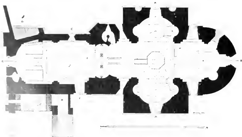
GRUNDRIß DER UNTERKIRCHE ZU SCHWARZ-RHEINDORF Mit Genehmigung des Provinzialkonservators der Rheinprovinz
