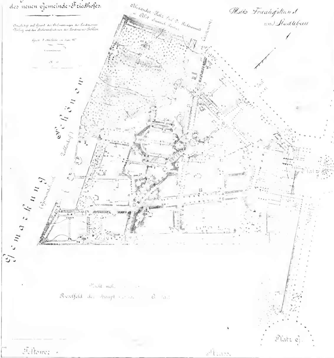
„Friedhofskunst und Stadtbau“. Wettbewerbsentwurf von J. P. Großmann, Leipzig, für den Zentralfriedhof in Groß Lichterfelde. Lageplan (ca. 1:3200).
