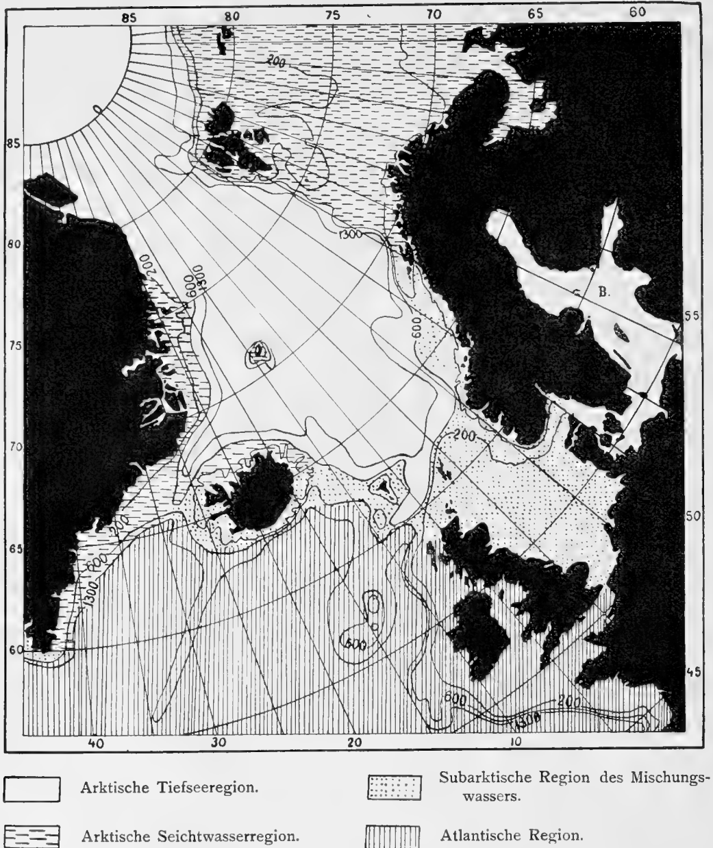
Fig. 46. Die hydrographischen und tiergeographischen Hauptregionen des norwegischen Nordmeeres und der angrenzenden Partien der arktischen Meere.
