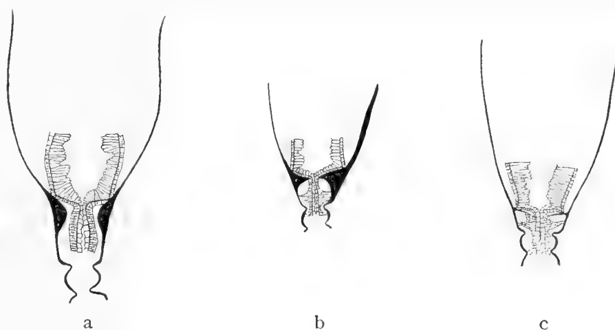
Fig. 38. Mediane Längsschnitte von Campanulariden-Hydrotheken. Vergr. \times 66 (Leitz, Okular 2, Objektiv 3). a Campanularia integra MACGILLIVRAY (von Solsvik bei Bergen). b Laomedea geniculata (LIN.) (von derselben Lokalität). c Laomedea flexuosa HINCKS (von dem Kristianiafjord bei Dröbak).
