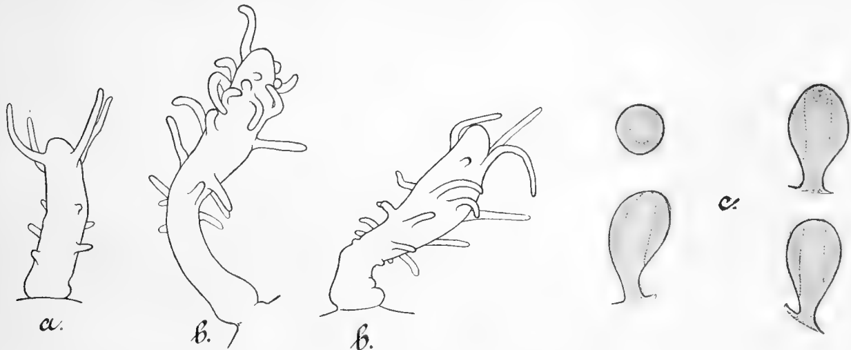
Fig. 1. Rhizogeton nudum n. sp. Vergr. \times 36^{\circ} . a junger Hydranth, b völlig entwickeltes Individuum, c Gonophoren.
