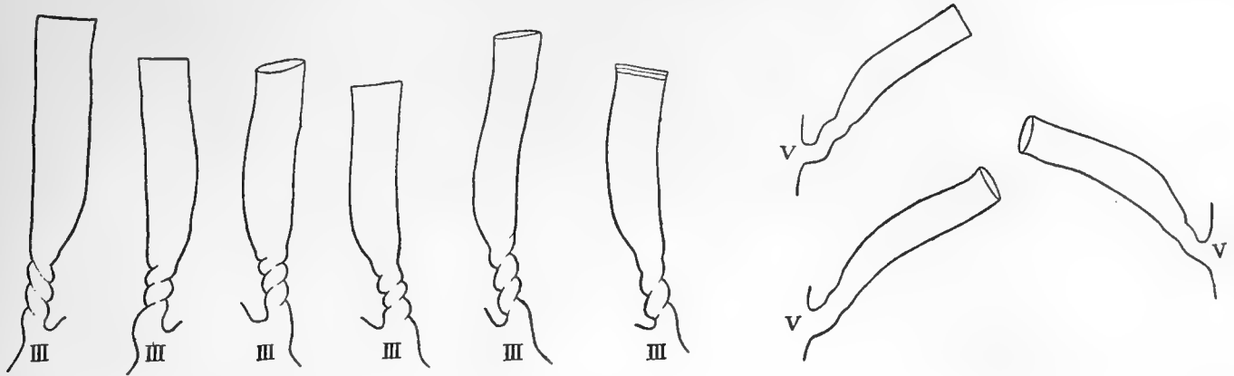
Fig. 17. Lafoëa gracillima (ALDER) forma typica . Vergr. \times 52 . Hydrothekenvariation. III Station 59. V Tisler, an der Mündung des Kristianiafjordes, 20—35 m Tiefe.
