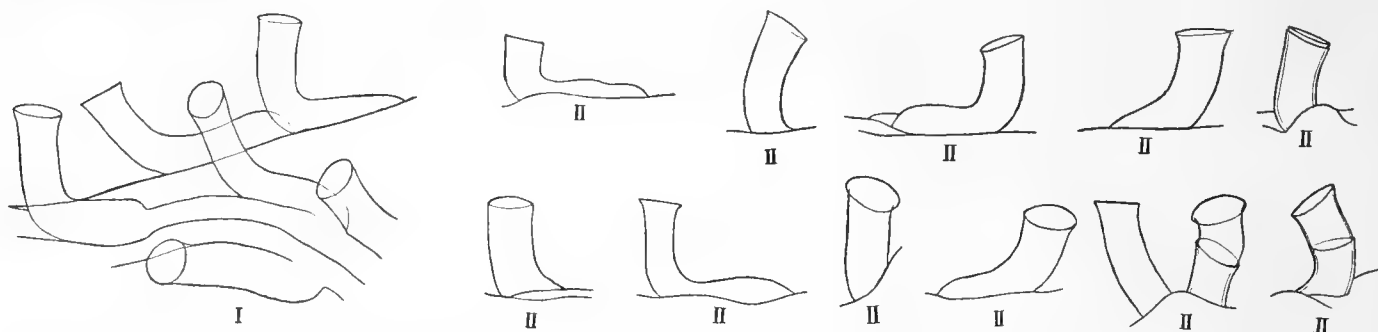
Fig. 21. Filellum serpens (HASSALL). Vergr. \times 52 . I Teil einer Kolonie von Station 56. II Variationen der freien Hydrothekenpartie (Station 59).
