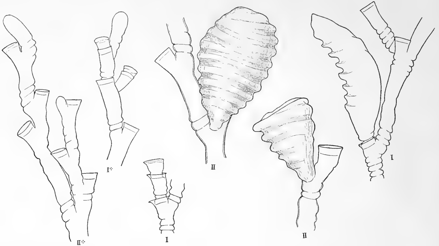
Fig. 12. Halecium ornatum NUTTING. Vergr. \times 25 . (Leitz, Okular 1, Objektiv 2), die übrigen \times 36 . I männliche, II weibliche Kolonie von Station 8.
