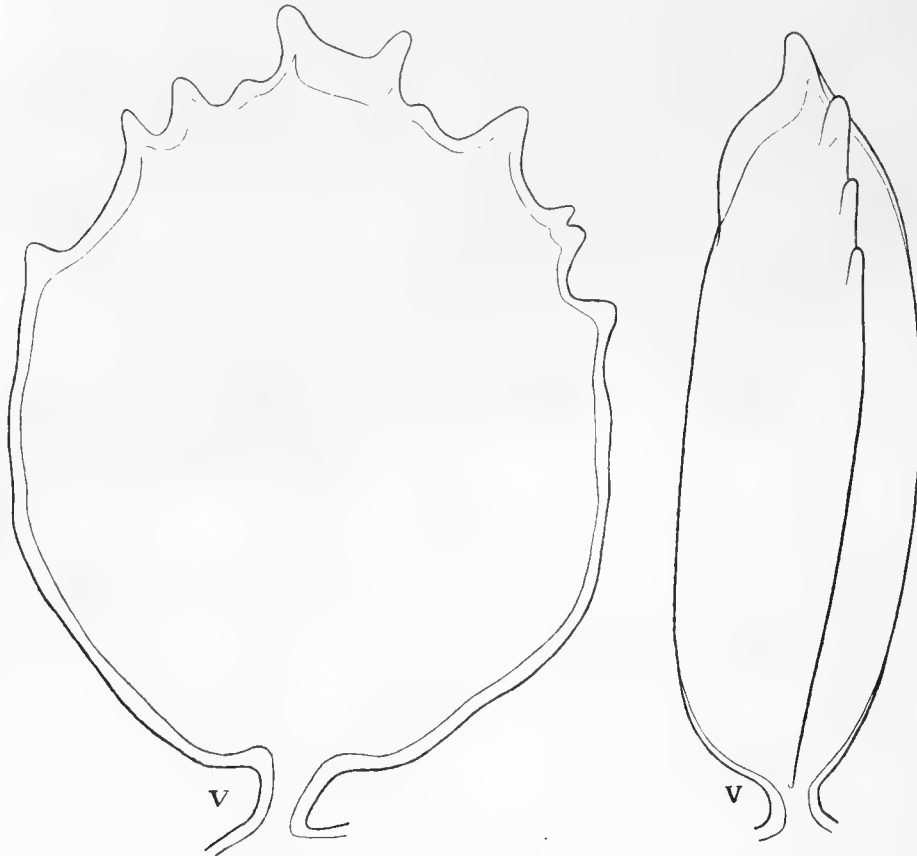
Fig. 15. Halecium minutum BROCH. Vergr. \times 36 . Weibliche Gonangien der Originalexemplare aus dem Nordmeere ( 64^{\circ} 17'5'' n. Br., 14^{\circ} 44' w. L., 75 m Tiefe).
