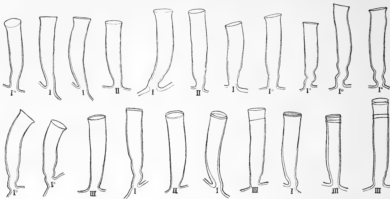
Fig. 16. Lafoëa dumosa (FLEMING). Vergr. \times 36 . Hydrothekenvariation (* auf kriechenden Stolonen). I Station 56. II Mittlere Nordsee ( 61^{\circ} 12' n. Br., 0^{\circ} 91' w. L., 160 m Tiefe). III Hvaler, an der Mündung des Kristianiafjords, 20—35 m Tiefe.
