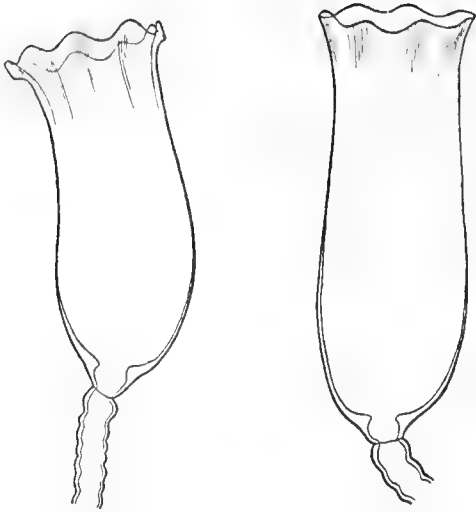
Fig. 42. Campanularia speciosa CLARK von Station 32. Vergr. 36.
