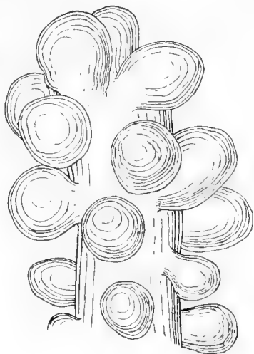
Fig. 2. Lampra spitzbergense n. sp. Vergr. \times 36 . a natürliche Größe, b Blastostyl.
