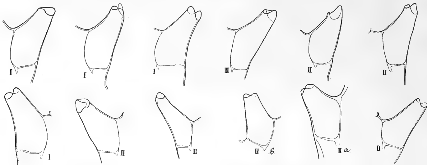
Fig. 27. Sertularia tenera G. O. SARS. Vergr. \times 52 . Hydrothekenvariation. I Station 46, ♀. II Station 47, ♂ (a an einem Hauptstamme, b von einer Zweigecke).
