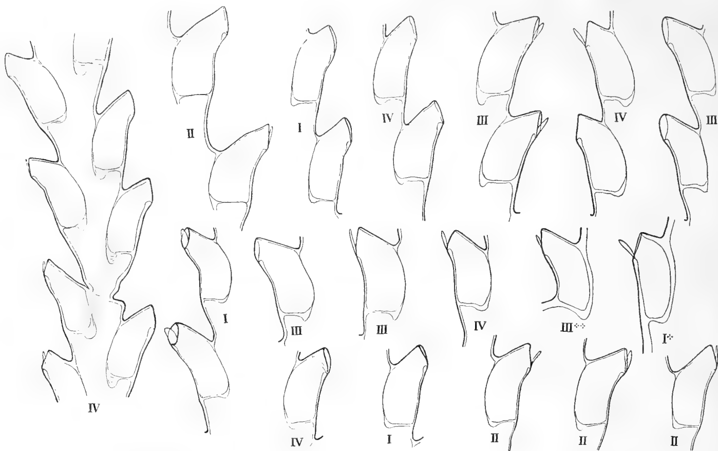
Fig. 32. Thuiaria carica LEVINSEN. Vergr. \times 36 . Hydrothekenvariation. I Station 8. II Station 24. III Station 37. IV Station 47. (* am Hauptstamme, ** von einer Zweigecke.)
