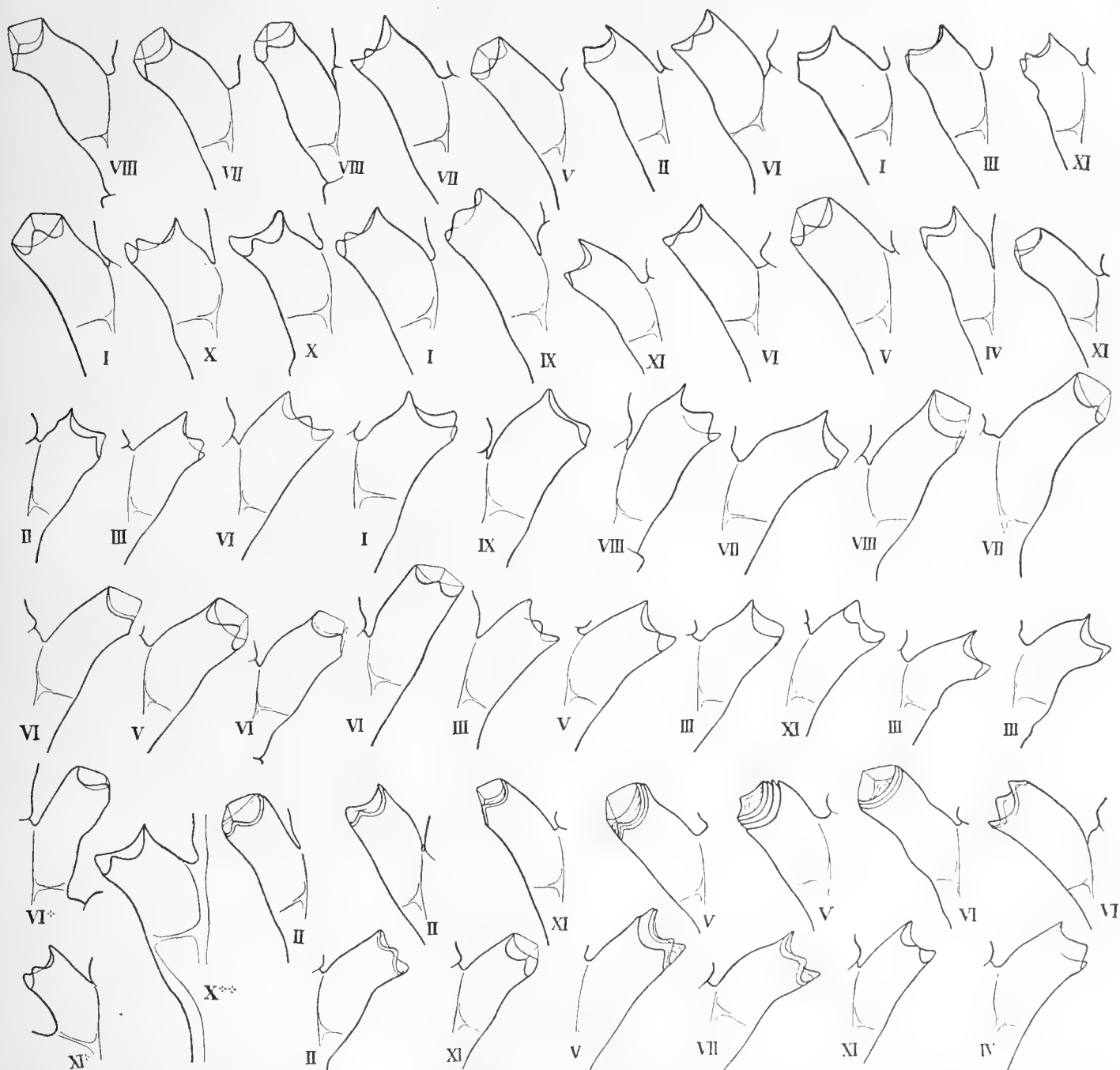
Fig. 25. Sertularella tricuspidata (ALDER). Vergr. \times 36 . Hydrothekenvariation. I Station 8. II Station 15. III Station 25. IV Station 29. V Station 30. VI Station 32. VII Station 32. VIII Station 45. IX Station 56. X Station 56. XI Station 59. (* in einer Zweigecke, ** an einem ausgeprägten Hauptstamme.)
