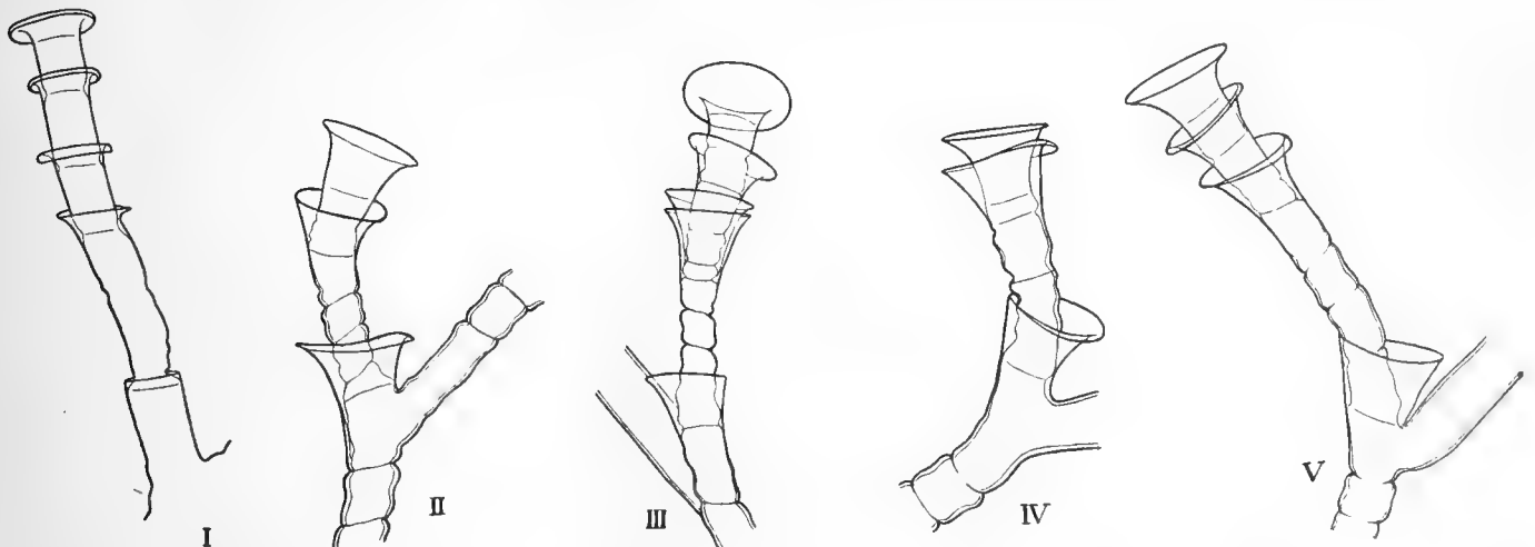
Fig. 14. Halecium sp. ( minutum BROCH aff.). Vergr. \times 52 . Hydrothekenverhältnisse. I Station 37. II Station 56. III Station 59. IV Original exemplar von 62^{\circ} 16' n. Br., 6^{\circ} 6' w. L., 110 m Tiefe. V Original exemplar, ♀, von 64^{\circ} 17' n. Br., 14^{\circ} 44' w. L., 75 m Tiefe.
