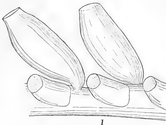
Fig. 33. Thuiaria carica LEVINSEN. Vergr. \times 36 . Männliche Gonotheken von Station 8.
