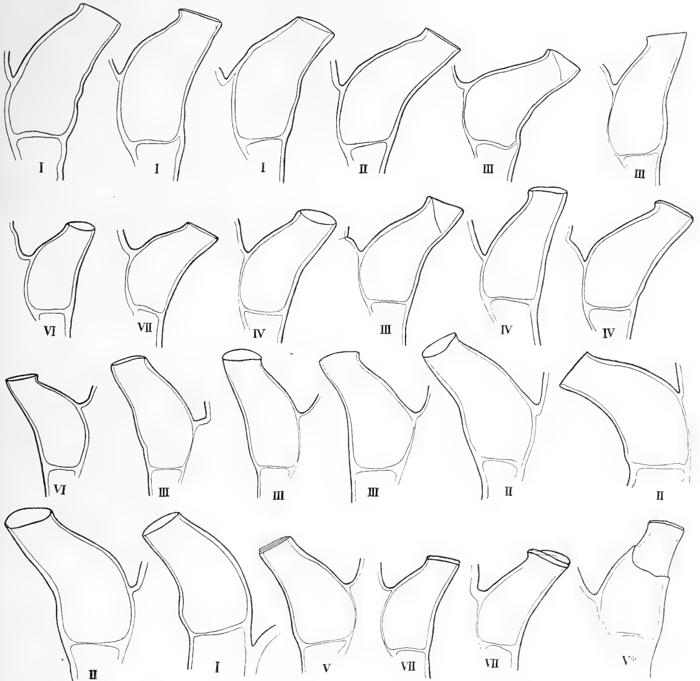
Fig. 35. Diphasia abietina (LIN.) forma typica . Vergr. \times 36 . Hydrothekenvariation (* Primärhydrothek verletzt). I Station 32. II Station 32. III Station 56. IV Station 56. V Station 56. VI Oestliche Nordsee ( 56^{\circ} 4' n. Br., 6^{\circ} 45' ö. L., 41 m Tiefe). VII Tisler (an der Mündung des Kristianiafjordes), 20–30 m Tiefe.
