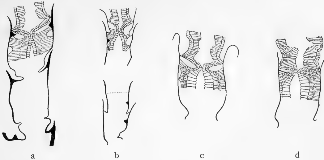
Fig. 3. Mediane Längsschnitte von Halecium -Hydrotheken. Vergr. \times 90 (Leitz, Okular 4, Objektiv 3). a Halecium halecinum (LIN.) (Station 45). b Halecium muricatum (ELL. et SOL.) (Station 51). c Halecium labrosum ALDER (Station 32). d Halecium ornatum NUTTING (Station 8).
