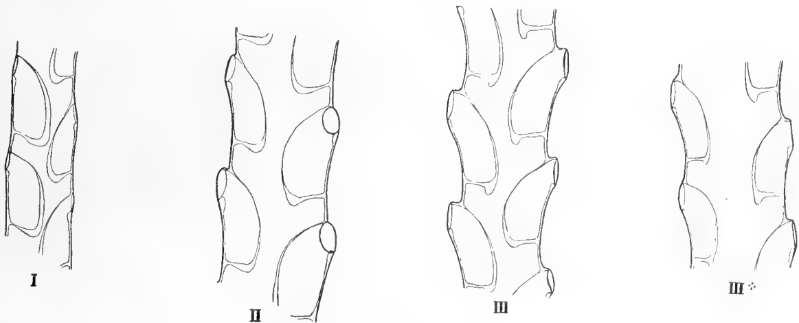
Fig. 31. Thuiaria laxa ALLMAN. Vergr. \times 36 . Zweigteile. I Station 9. II Station 47. III Originalexemplar von der Thuiaria Hjorti BROCH (28) von 61^{\circ} 21' n. Br., 5^{\circ} 12' w. L., 375 m Tiefe. (* Basalstück eines Zweiges.)
