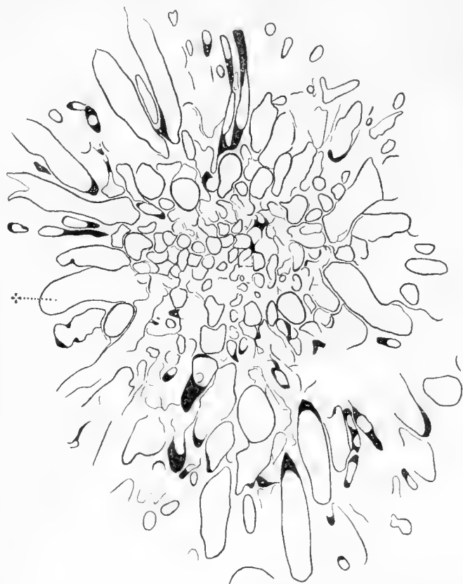
Fig. 23. Querschnitt von einer Kolonie der Lafoëina maxima LEVINSEN von Station 5. Vergr. \times 25 . (Nur die chitinigen Teile sind eingezeichnet worden.) Bei dem * ist ein Gonangium getroffen.
