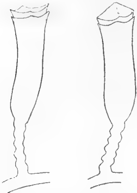
Fig. 24. Lovenella quadridentata (HINCKS) von Station 15. Vergr. \times 52 .
