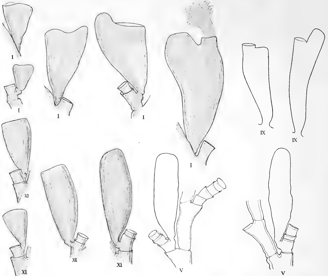
Fig. 5. Halecium halecinum (LIN.). Vergr. \times 36 . Gonangien. I Entwicklung der weiblichen Gonotheke (Station 9). XI Entwicklung der männlichen Gonotheke (Station 9). V Völlig entwickelte männliche Gonotheke (Station 25). IV Völlig entwickelte weibliche Gonotheke aus der südöstlichen Nordsee.
