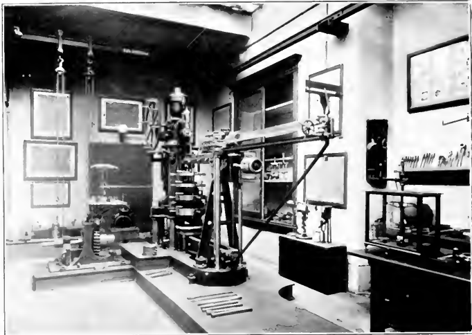
Mechanisch-technisches Laboratorium.
