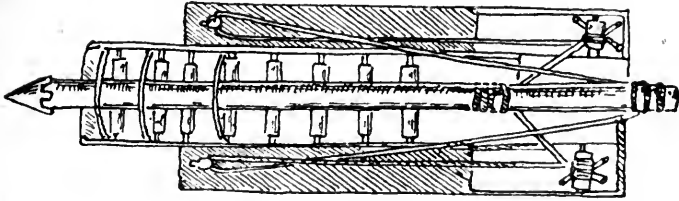
54. I Römischer Mauerbohrer (terebra), nach Wefcher.
