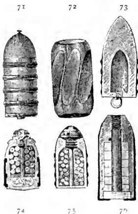
74. Shrapnel für österreichische gezogene Geschütze.
