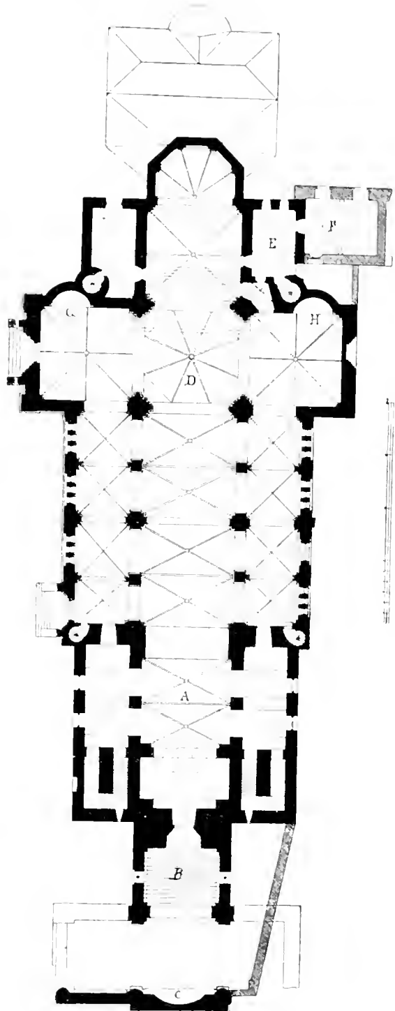
Fig. 39. Werden. Grundriss der Abteikirche.
