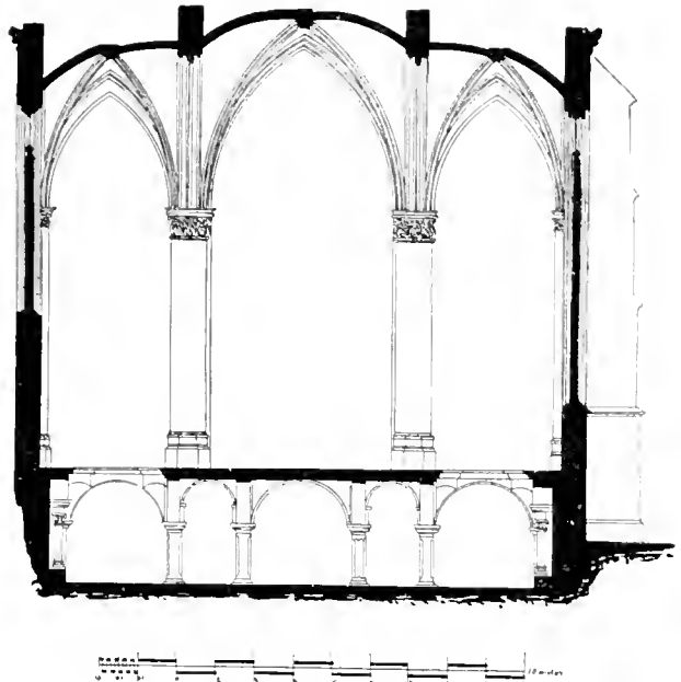
Fig. 8. Essen. Querschnitt durch den Hochchor der Munsterkirche
