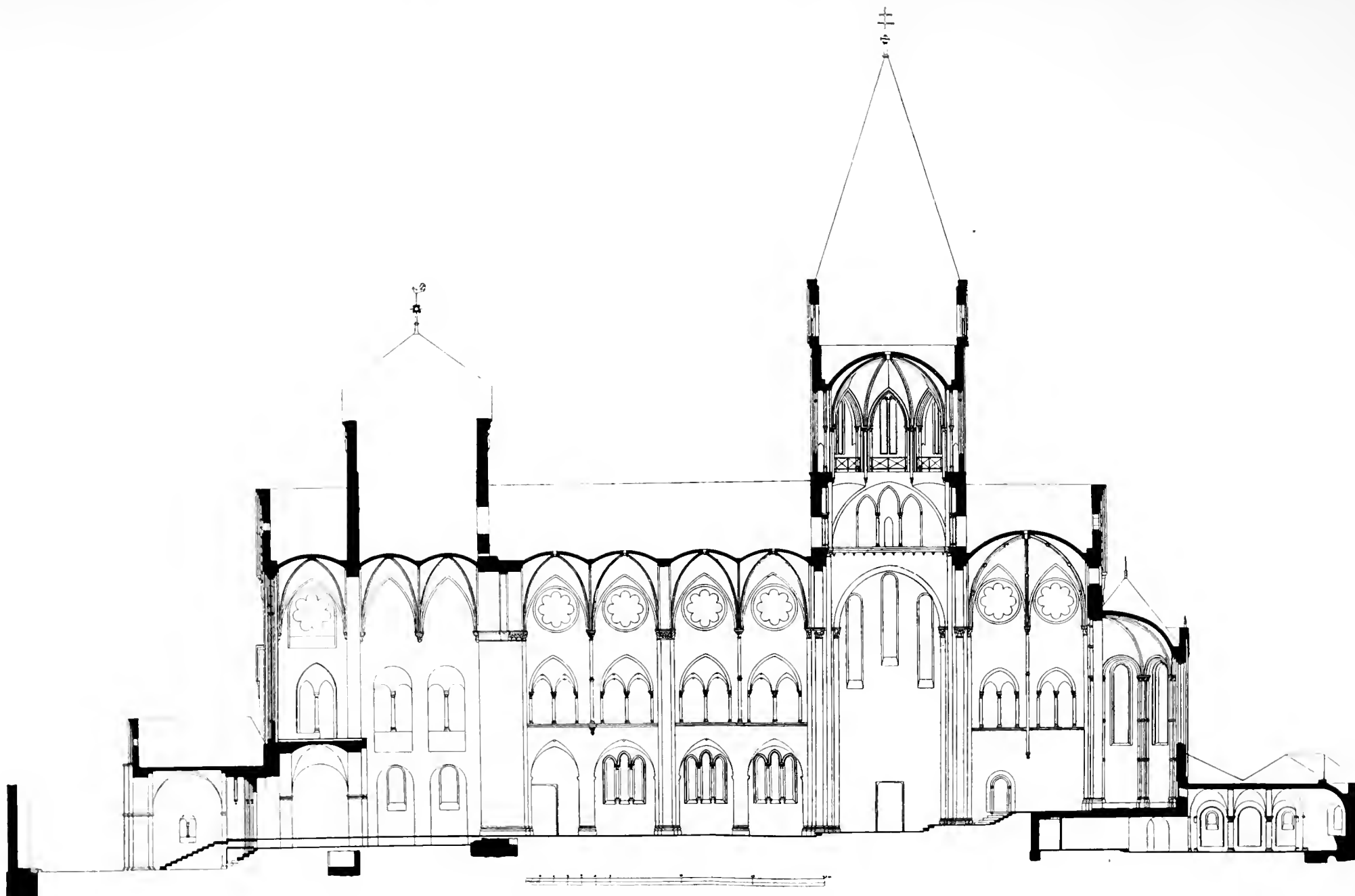
Werden. Längsschnitt durch die Abteikirche.
