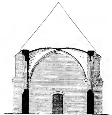
Querschnitt der Kirche.
