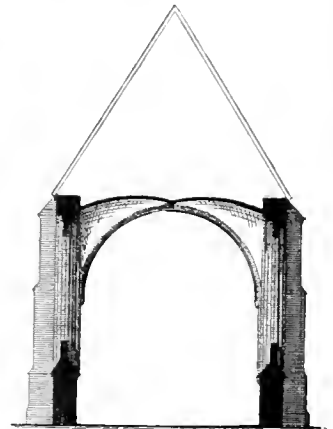
Querschnitt der Kirche.
