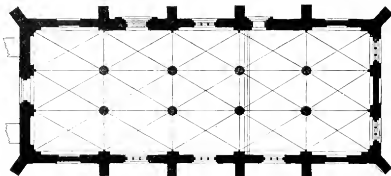
Grundriss der Kirche.
