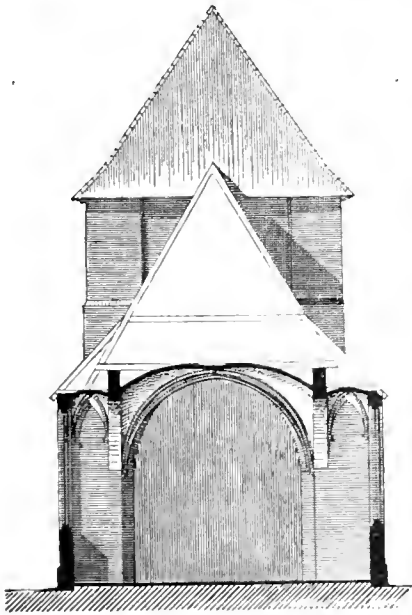
Querschnitt.
