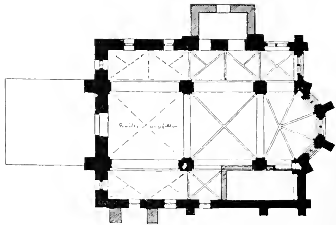
Grundriss der Kirche zu Gross-Salitz.
