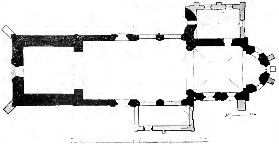
Grundriss der Kirche.
