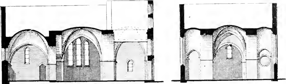
Längsschnitt
