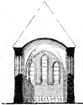
Querschnitt des Chors.
