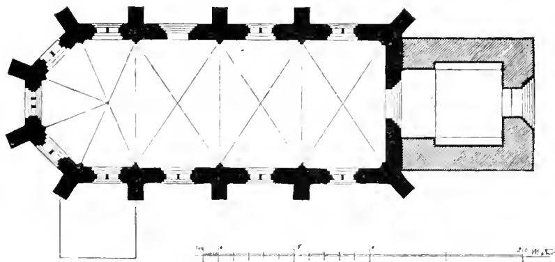
Grundriss der Kirche.
