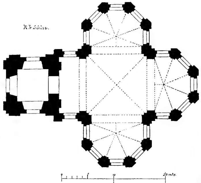
Grundriss der Schelfkirche.
