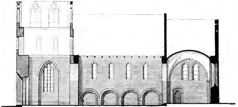
Längsschnitt der Kirche zu Neuburg.
