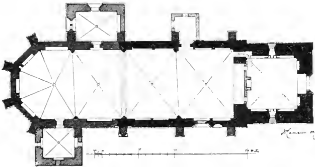
Grundriss der Kirche.
