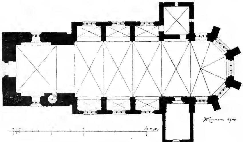
Grundriss der Kirche.
