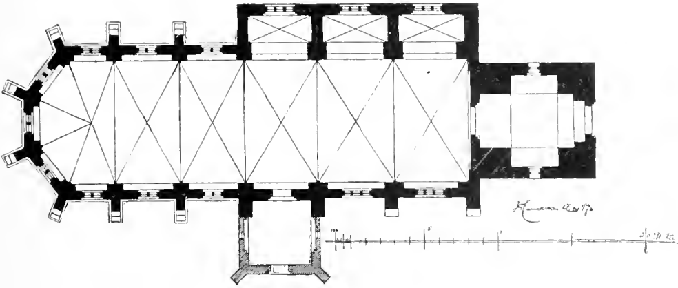
Grundriss der Kirche zu Gressow.
