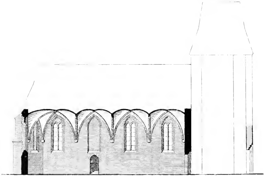
Längsschnitt der Kirche zu Hornstorf.
