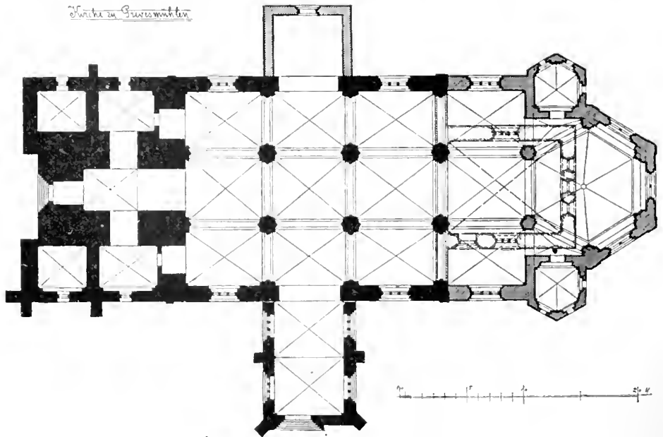
Grundriss der Kirche zu Grevesmühlen.
