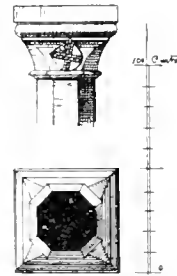
Pfeiler mit Grundriss.
