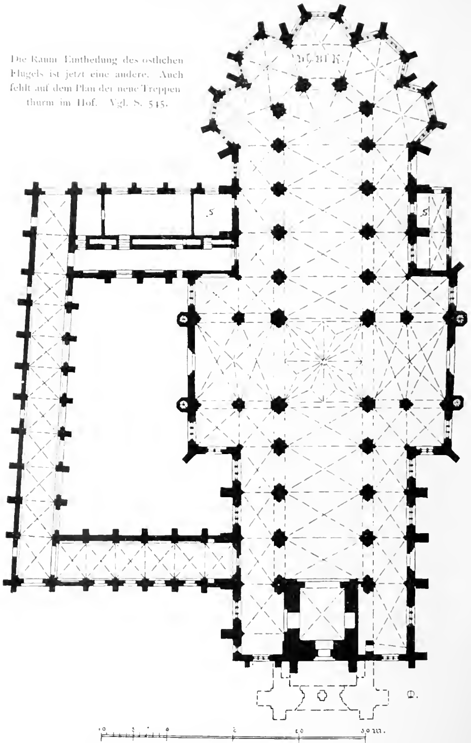
Grundriss des Domes zu Schwerin.
