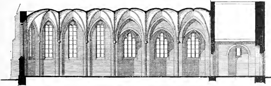
Längsschnitt der Kirche.
