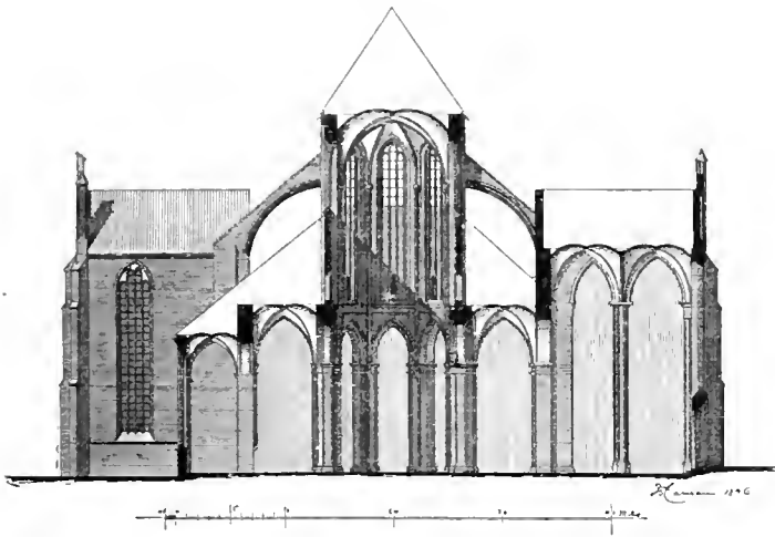
Querschnitt der Marien-Kirche.
