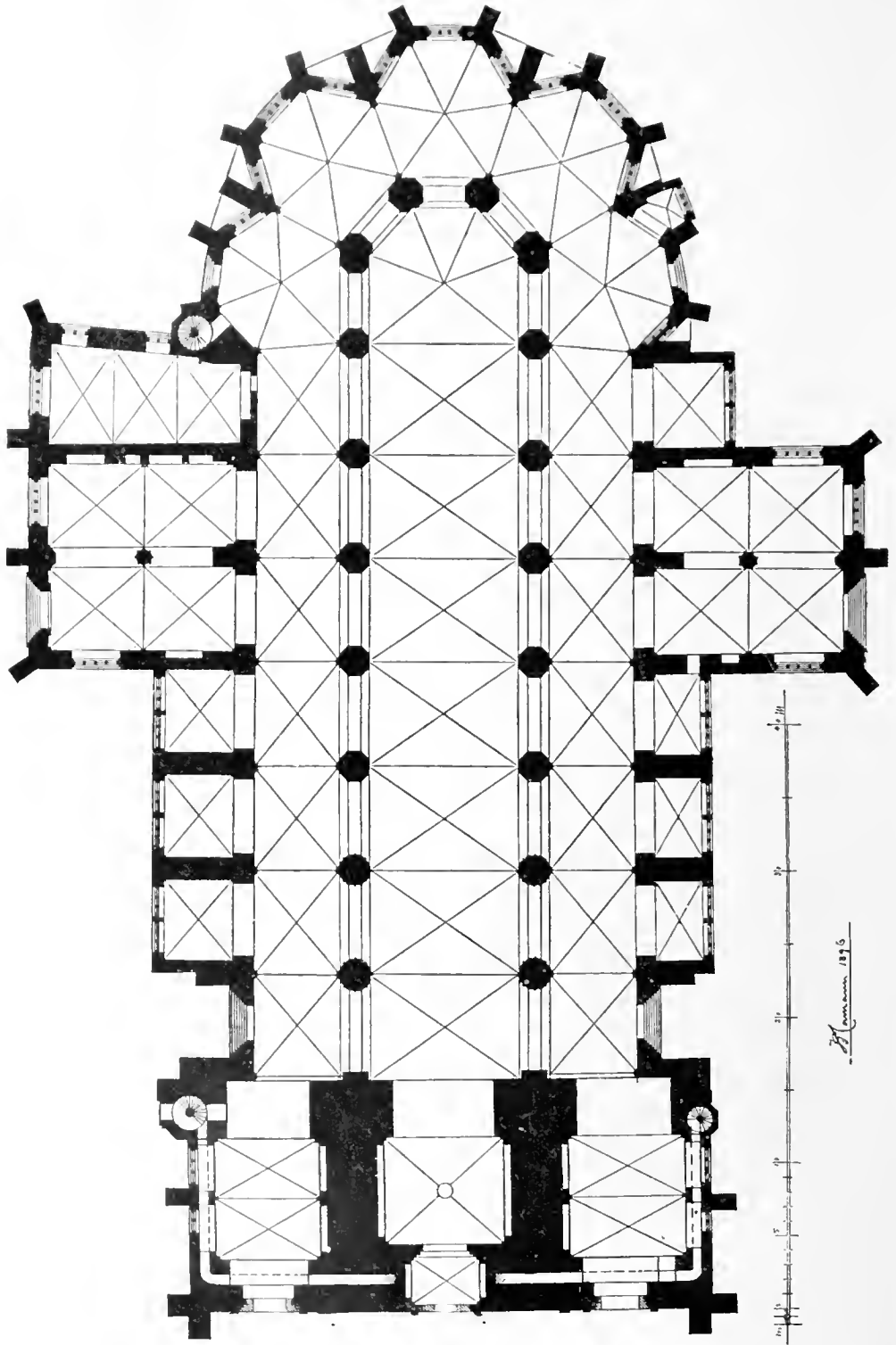
Grundriss der Marien-Kirche.
