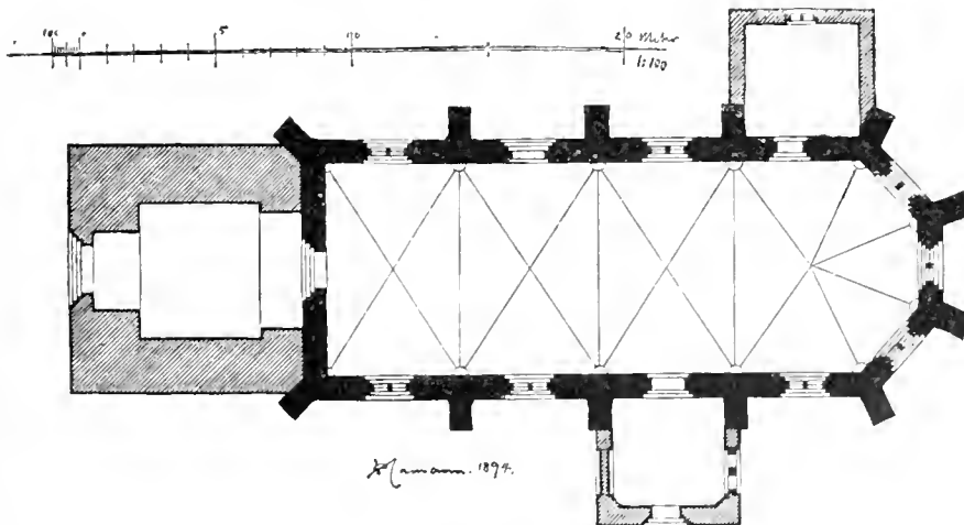
Grundriss der Kirche.
