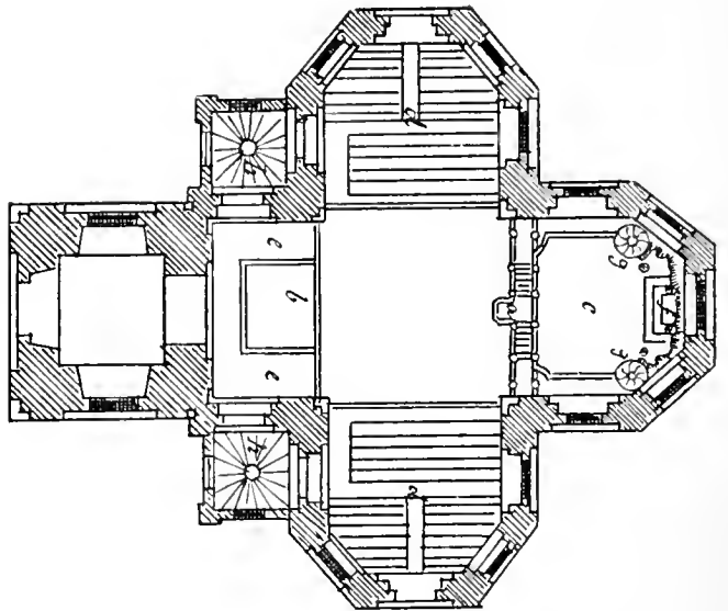
Innere Einrichtung der Kirche nach dem Vorschlag von Sturm.
