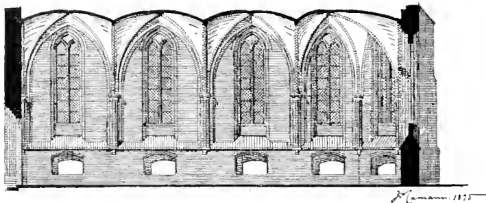
Längsschnitt des Schiffes der Kirche zu Zurow.
