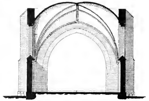
Querschnitt des Chores.
