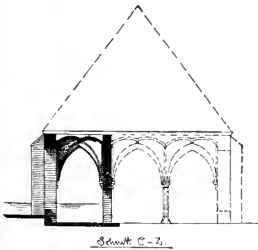
Querschnitte.
