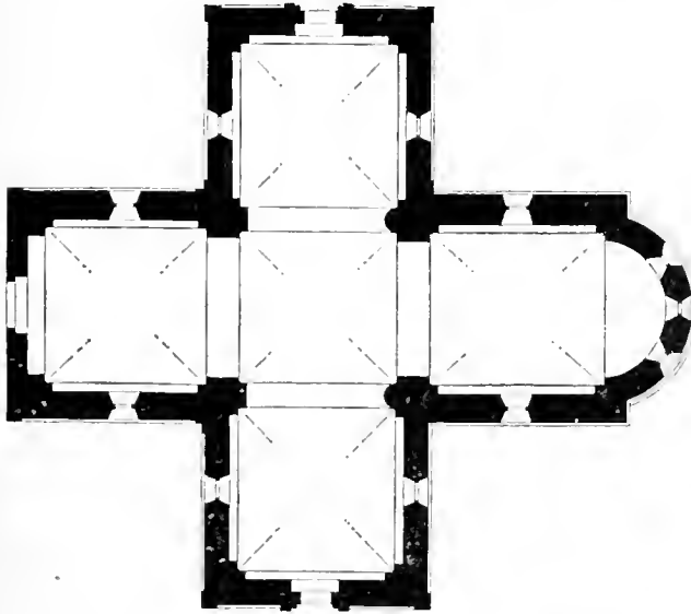
Grundriß der Kirche zu Vietlütbe.
