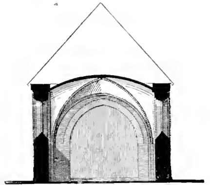
Querschnitt des Chors.
