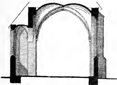
Querschnitt des Chores.
