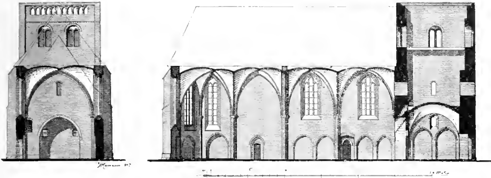
Querschnitt und Längsschnitt der Kirche zu Kirchdorf auf Poel.
