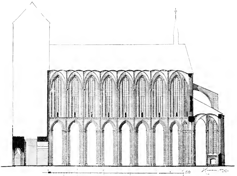
Querschnitt und Längsschnitt der St. Nikolai-Kirche.
