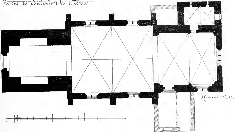
Grundriss der Kirche zu Beidendorf.
