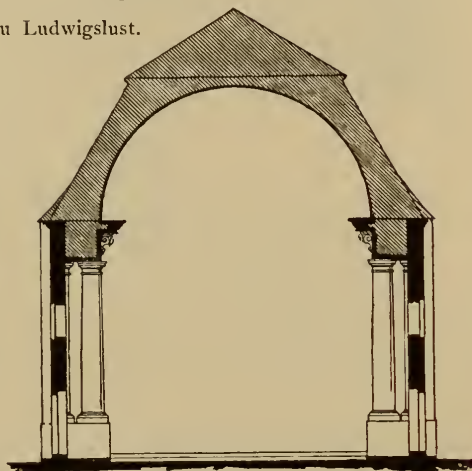
Querschnitt der Stadtkirche.
