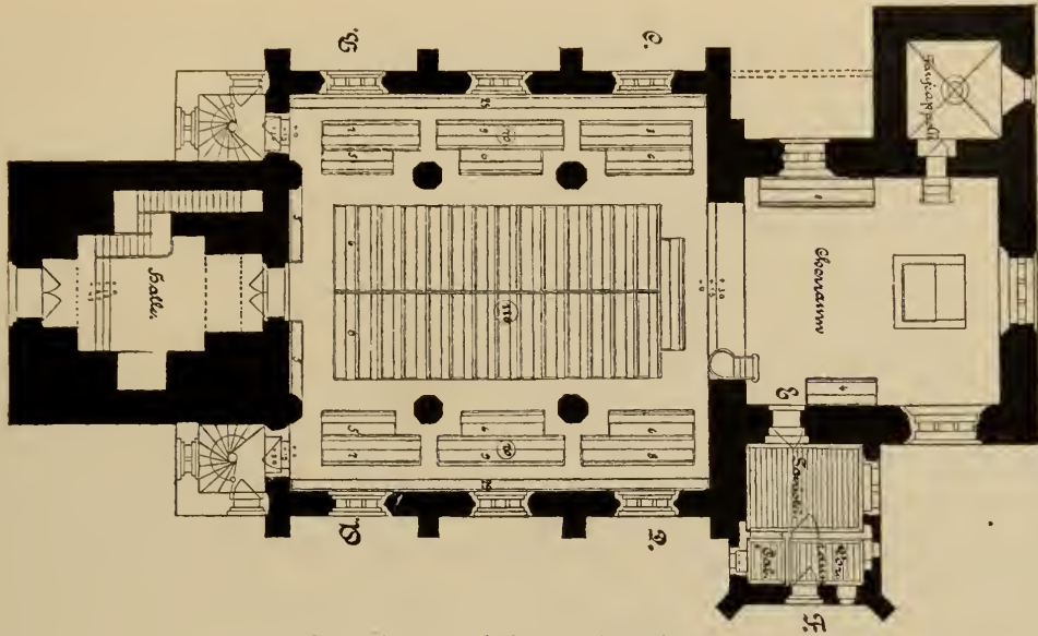
Grundriss der Kirche zu Lichtenhagen.
