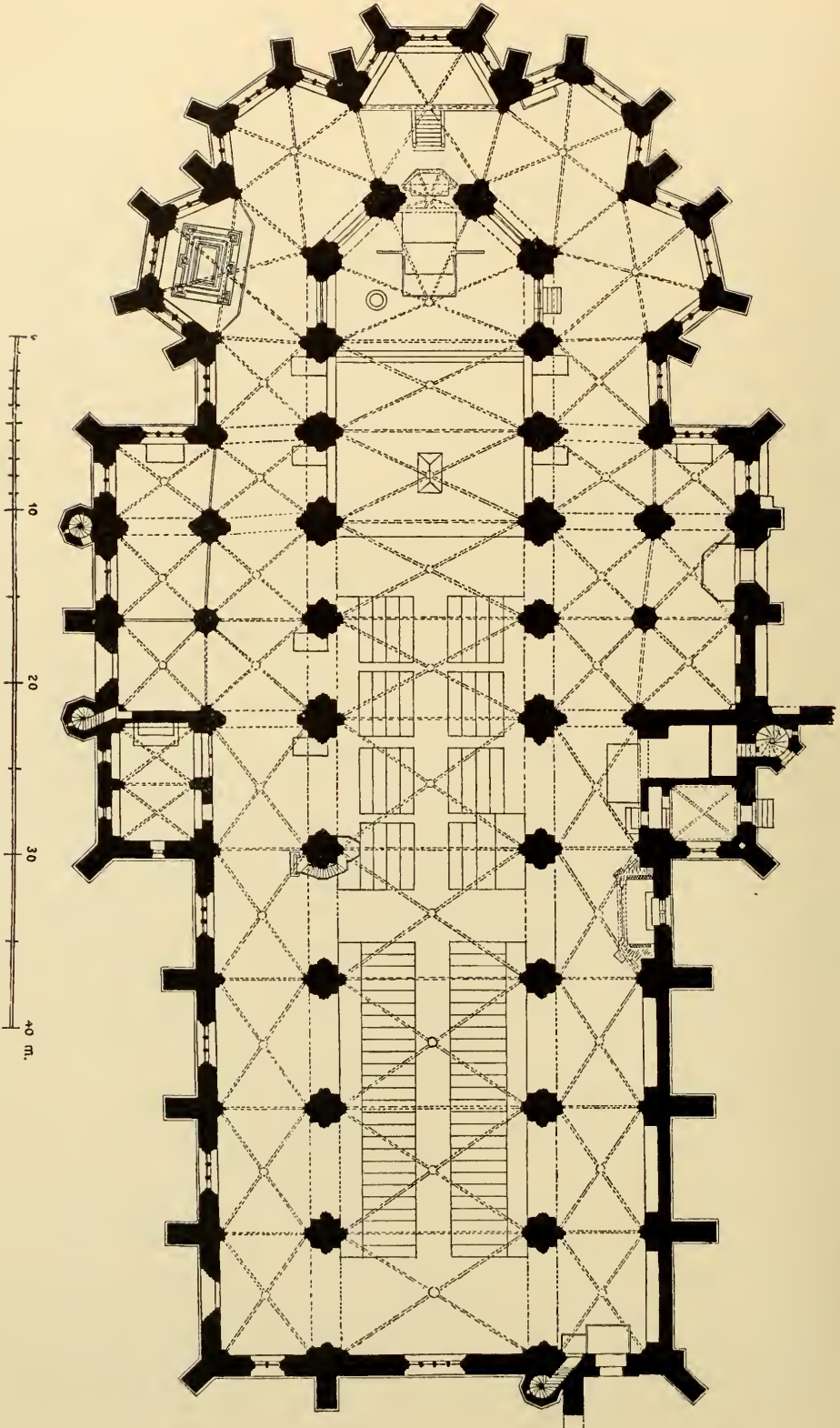
Grundriss der Kirche zu Doberan. (Nach Mückel)
