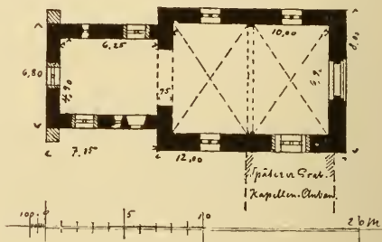
Grundriss der Kirche.
