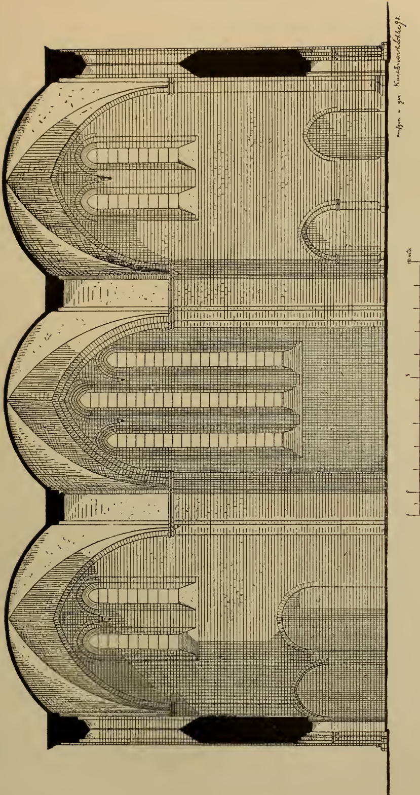
Querschnitt der Kirche zu Neukloster.
