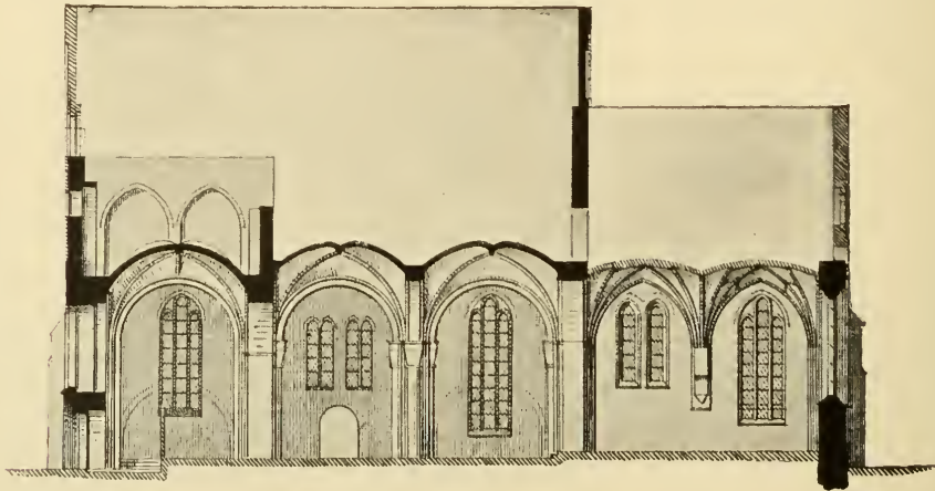
Längsschnitt der Kirche.
