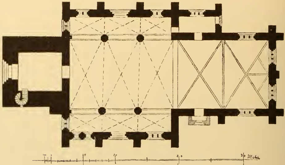
Grundriss der Kirche zu Grabow. (Hamann.)
