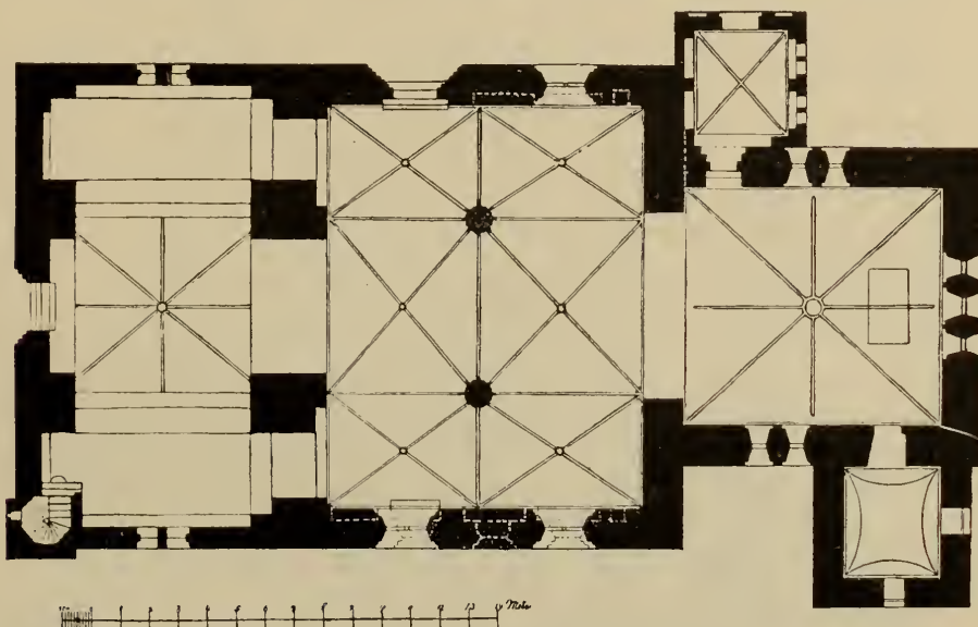
Grundriss der Kirche zu Parkentin.
