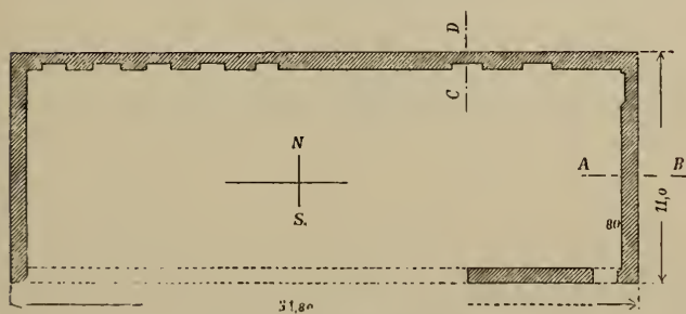
Grundriss der »Wolfsscheune«.
