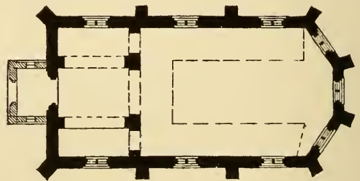
Grundriss der Kirche.
