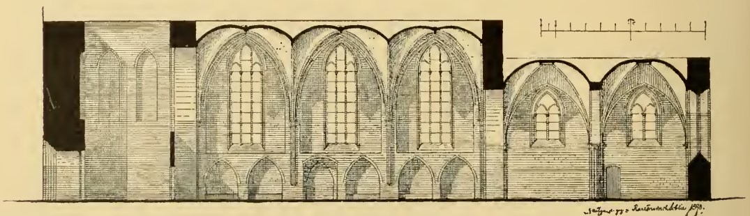
Längsschnitt der Kirche.
