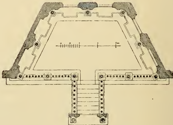
Grundriss der Grabkapelle Herzog Adolf Friedrich's. Nach Scheffers.
