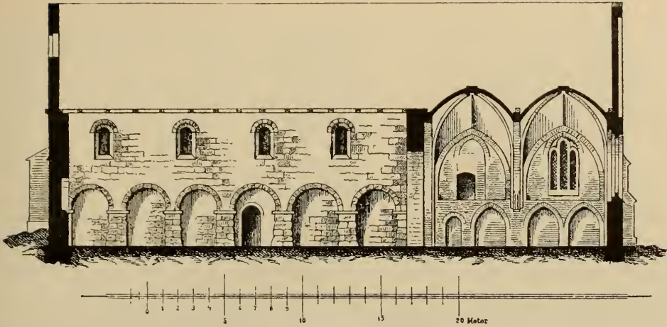
Längsschnitt der ehemaligen Kirche zu Vellahn.
