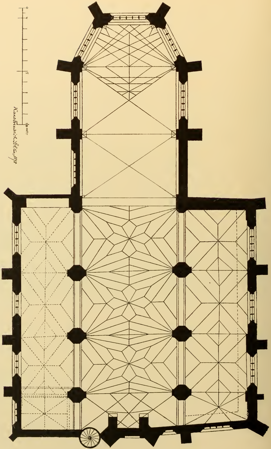
Grundriss der Kirche zu Tempzin.
