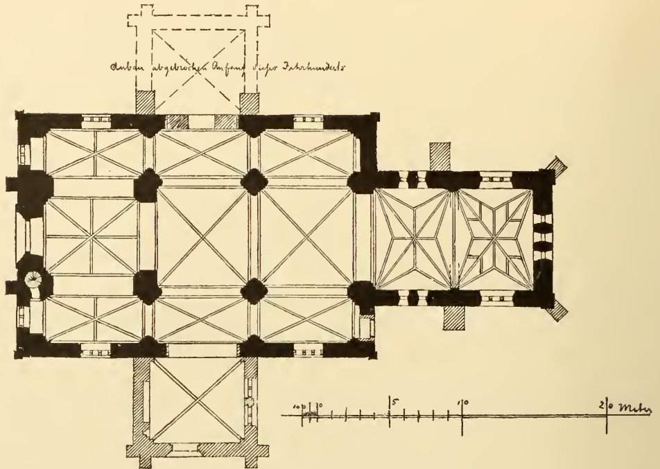
Grundriss der Kirche zu Wittenburg.
