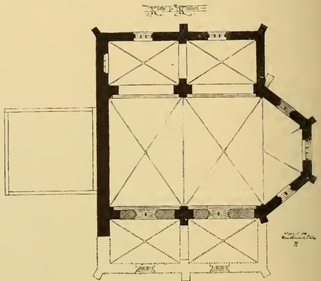
Grundriss der Kirche.
