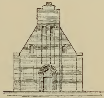
Aufriss der Westseite der Kirche.
