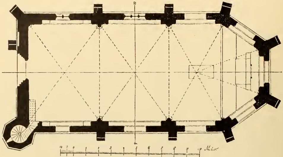
Grundriss der Kapelle zu Althof.
