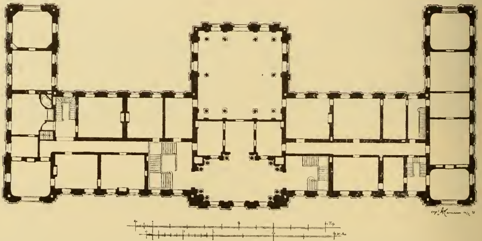
Grundriss des Untergeschosses des Schlosses.
