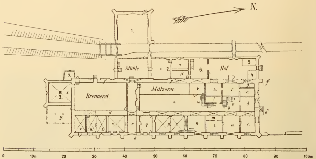
Grundplan des Wirtschaftshofes (Brauerei mit Mühle). Nach Möckel.
