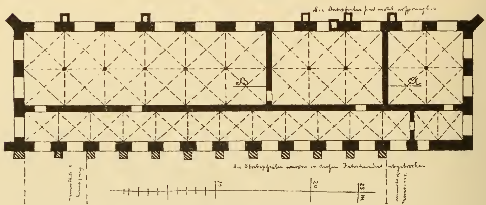
Grundriss des Klosterhauses.
