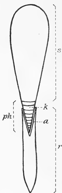
Fig. XI. Schema eines Belemniten.
