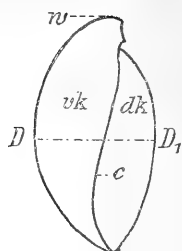
Fig. IV b. Seitenansicht.
