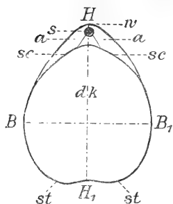
Fig. IV a. Rückenansicht.
