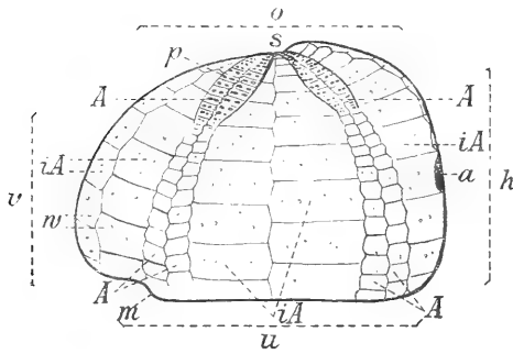
Fig. II. Irregulärer Seeigel.
