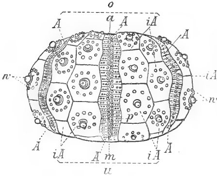
Fig. I. Regulärer Seeigel.
