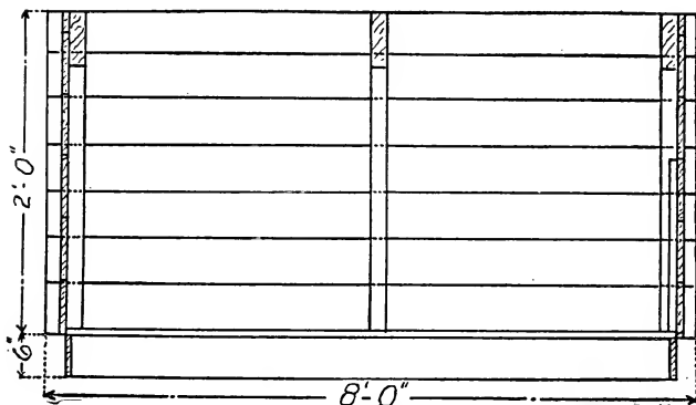
FIG. 15—LONGITUDINAL SECTION
