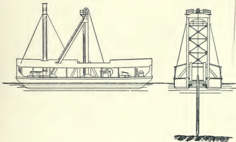
FIG. 4.—Lobnitz Rockcutter.
