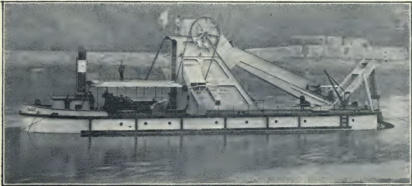
FIG. 18.—Dredge "Cadiz."
