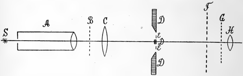
Схема расположенія опыта, если смотрѣть сверху.
