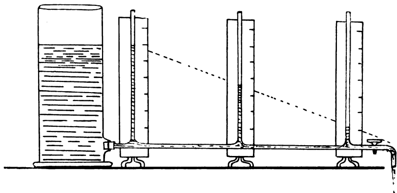
Fig. 2. Hydraulisches Abbild des elektrischen Stromes.
