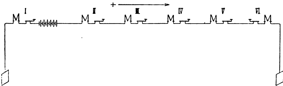
Fig. 204. Ruhestromschaltung.
