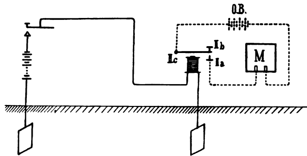
Fig. 178. Relaisprinzip.
