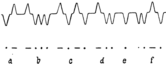
Fig. 217. Wellenförmige Morseschrift des Schnelltelegraphen.
