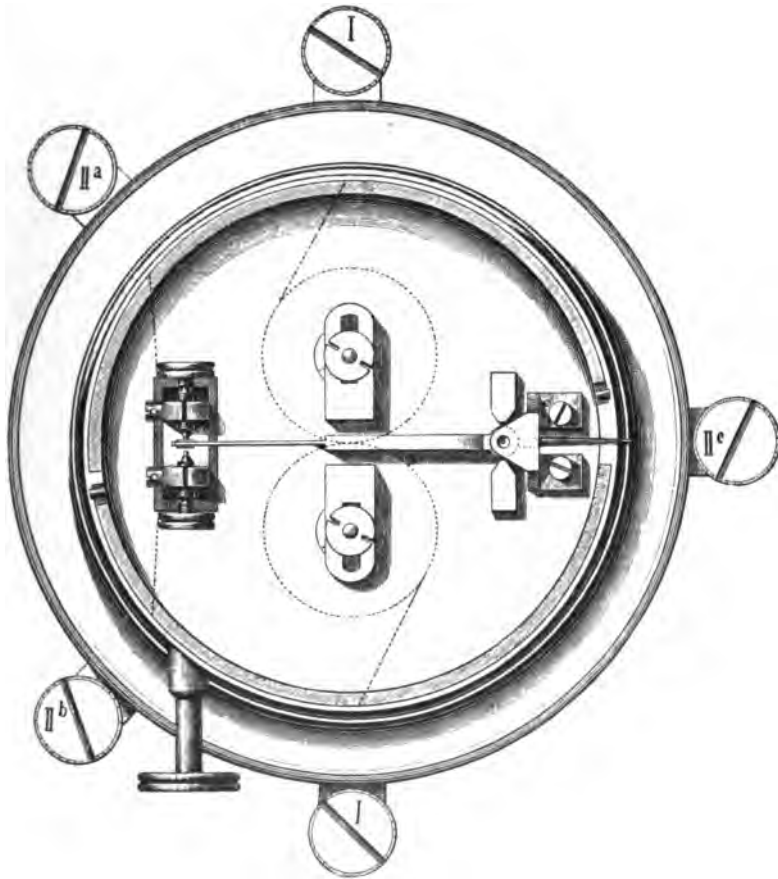
Fig. 184. Siemssches Polarisirtes Relais von oben.
