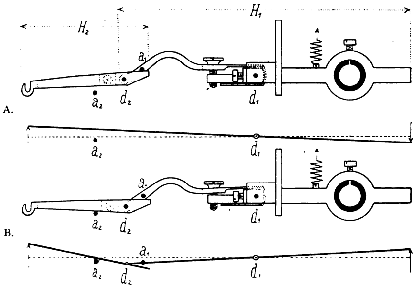
Fig. 150. Schriebhebel.
