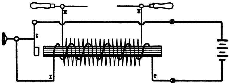
Fig. 52. Schema eines Funkeninduktors. Strom geschlossen.
