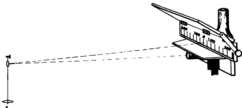
Fig. 269. Kabelgalvanometer. Spiegel, Skala, Beleuchtung.
