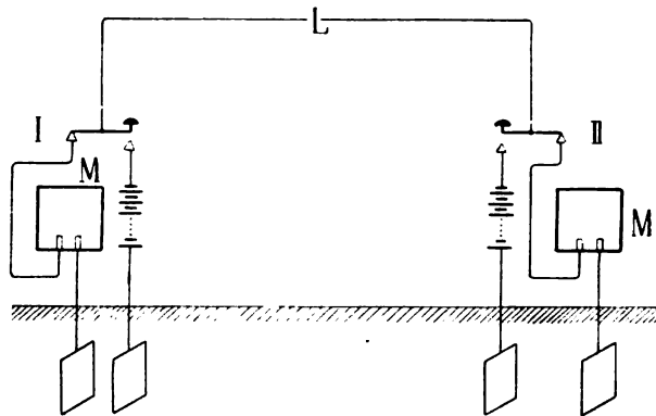
Fig. 203. Arbeitsstromschaltung.
