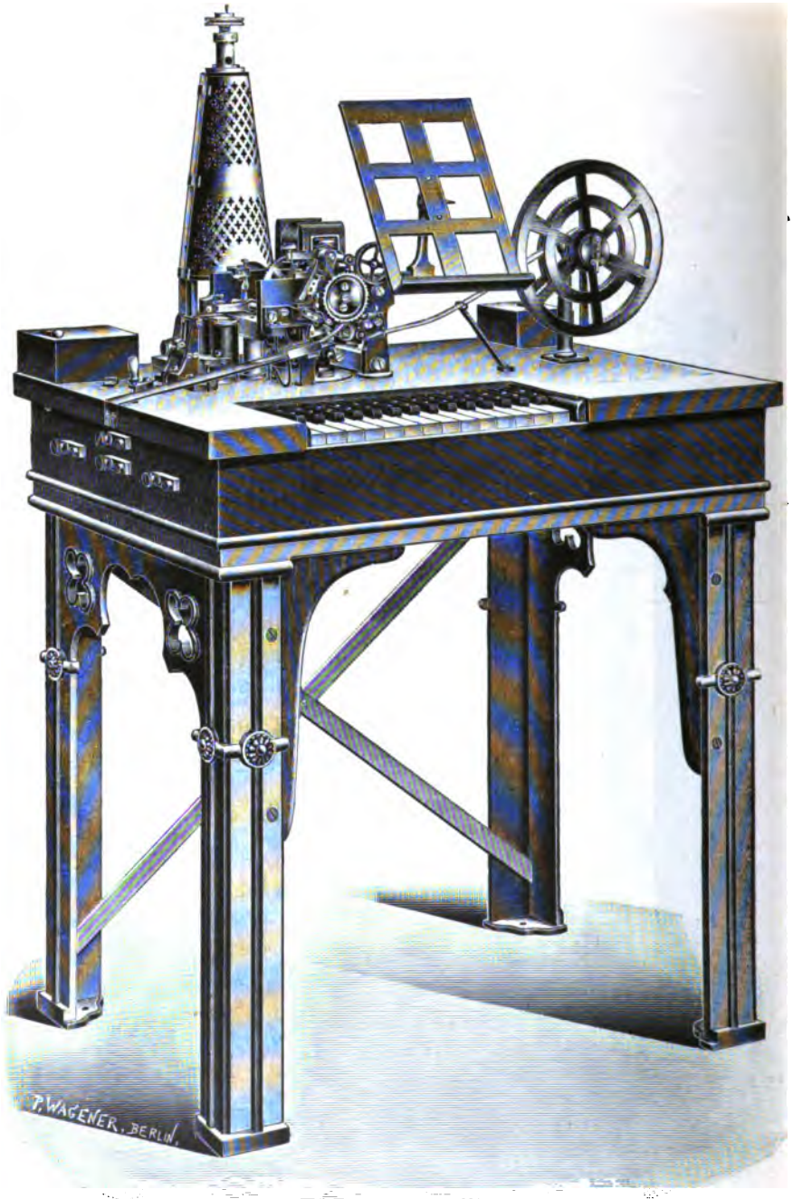
Fig. 221. Heutiger Hughes-Apparat.
