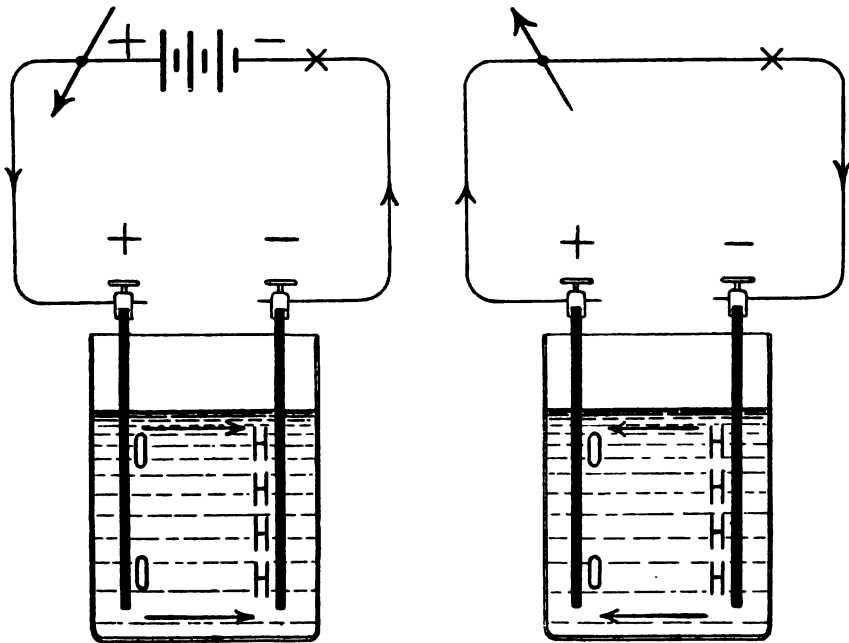
Fig 103. Platinbleche in verdünnter Schwefelsäure.
