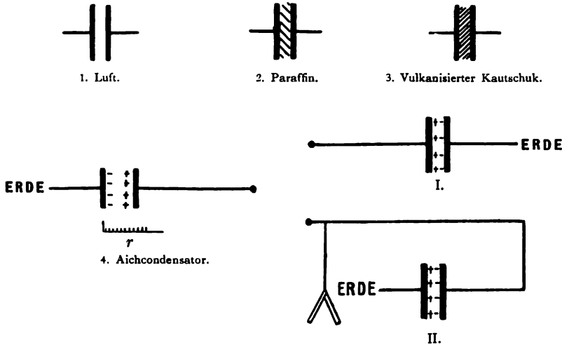
Fig. 69. Bestimmung der Dielektricitätsconstante.
