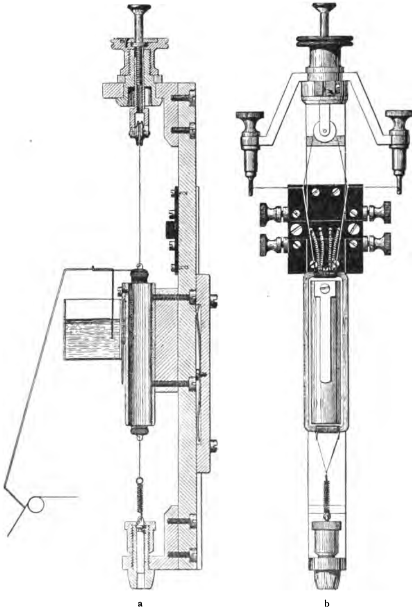
Fig. 271. Heberschreiber. Nach Montillot.
