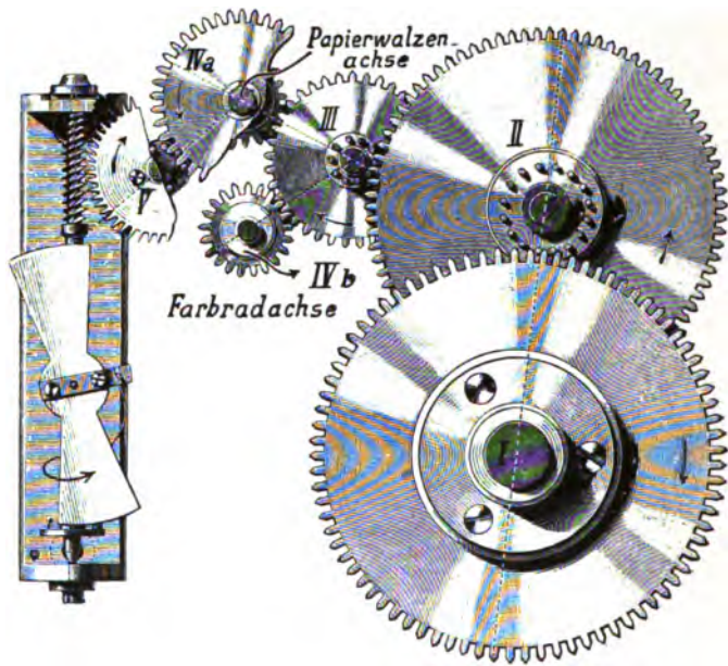
Fig. 151. Uhrwerk.
