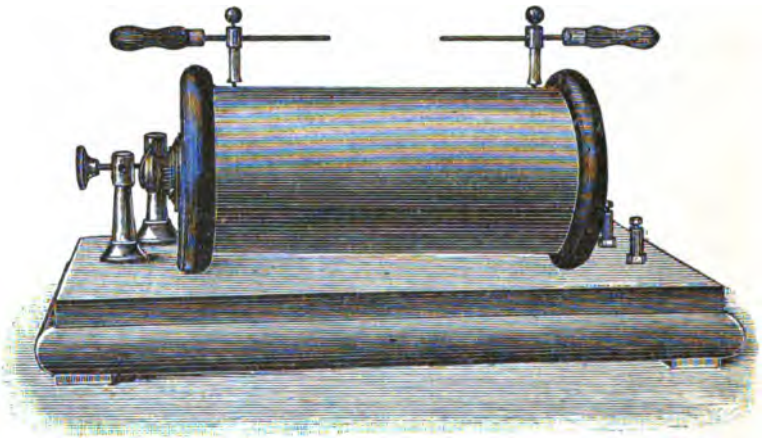
Fig. 50. Funkeninduktor. Etwa \frac{1}{4} .
