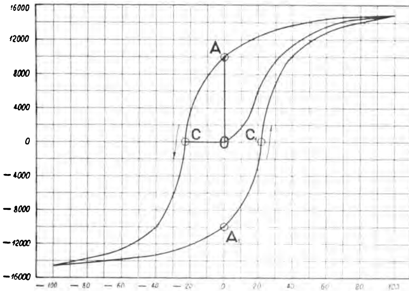
Fig. 44. Hysteresiskurve.
