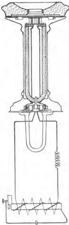
Fig. 285. Telephon mit Hufeisenmagnet, vom Induktorium gespeist.
