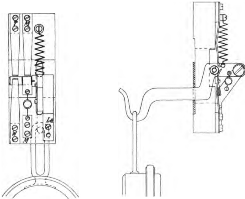
Fig. 322. Älterer Hakenumschalter.
