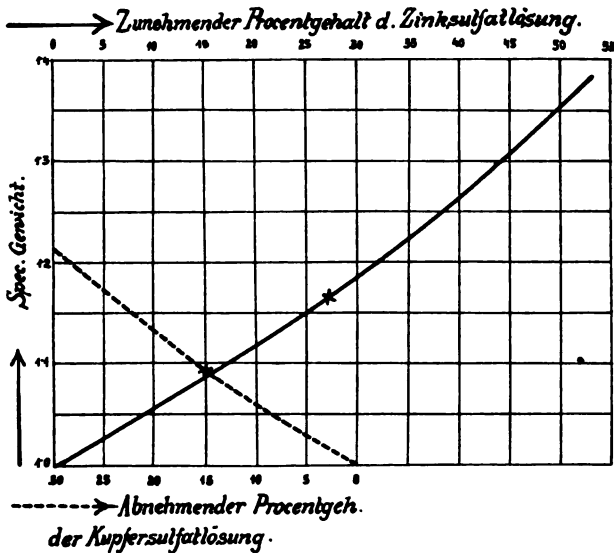
Fig. 87. Die Elektrolyte im arbeitenden Callaudschen Element.
