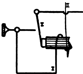
Fig. 52. Schema eines Funkeninduktors. Strom geschlossen.
