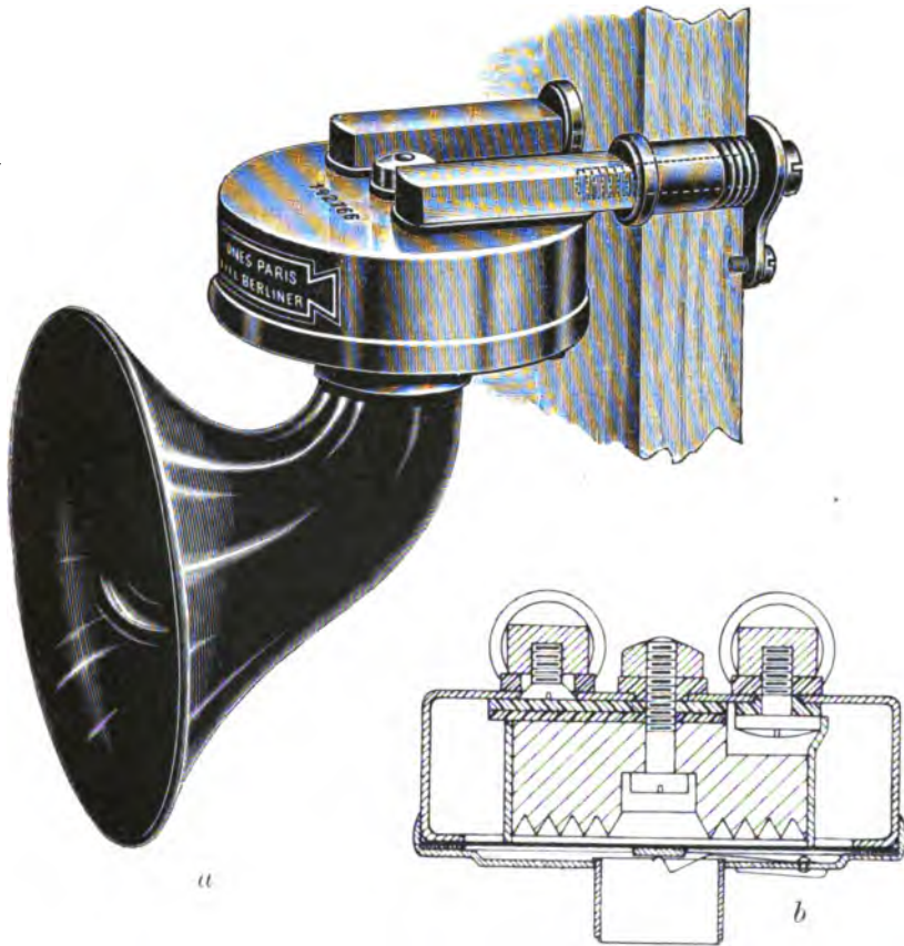
Fig. 314. Berlinersches Mikrophon.
