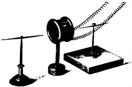
Fig. 37. Magnetische Wirkung einer Strom-durchflossenen Spule.
