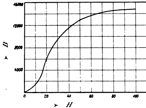
Fig. 43. Jungfräuliche Magnetisierungskurve.
