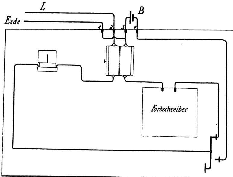
Fig. 210. Einfachste Arbeitsstromschaltung.
