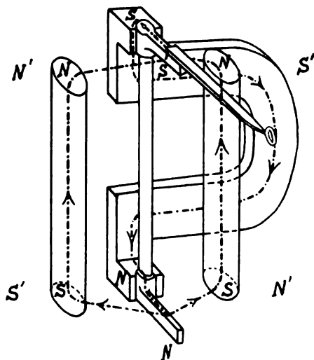
Fig. 187. Kraftlinienverlauf im Relais mit drehbaren Kernen.
