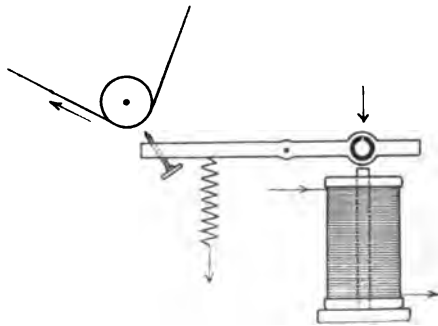
Fig 139. Schema des Morseempfängers.
