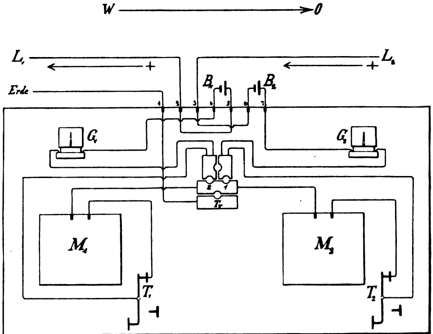
Fig. 216. Ruhestrom-Trennstelle.
