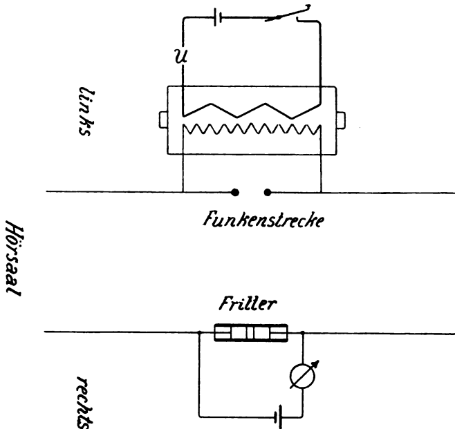
Fig. 338. Nachweis freier elektrischer Wellen.
