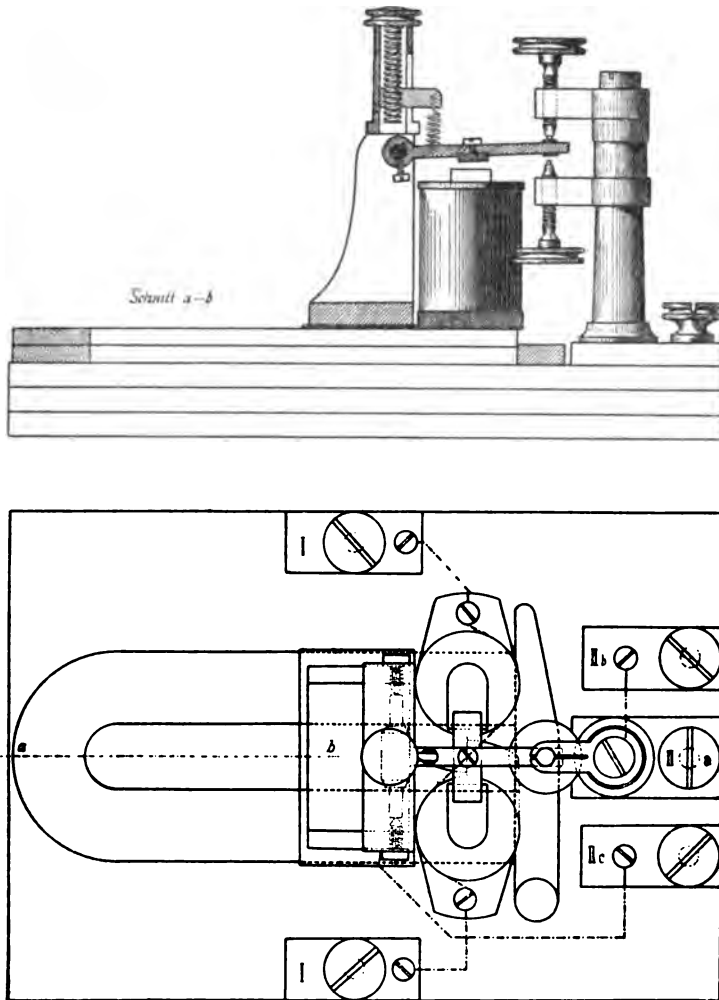
Fig. 180. Hughes-Relais.
