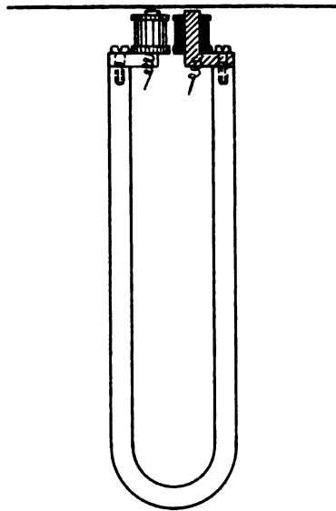
Fig 42. Polarisierter Elektromagnet des alten Siemensschen Telephons.
