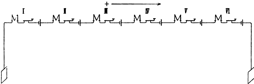
Fig. 205. Ruhestromschaltung. Batterie auf die ganze Ämterreihe verteilt.
