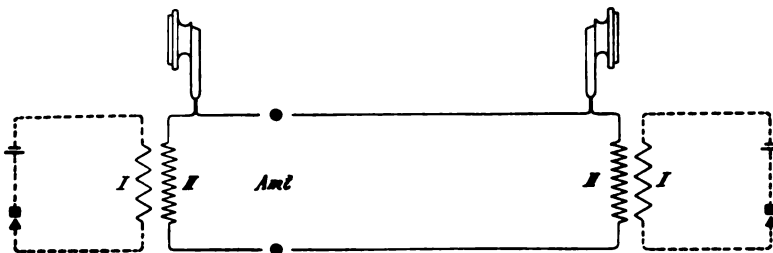
Fig. 297. Prinzipielle Fernsprechschtung.
