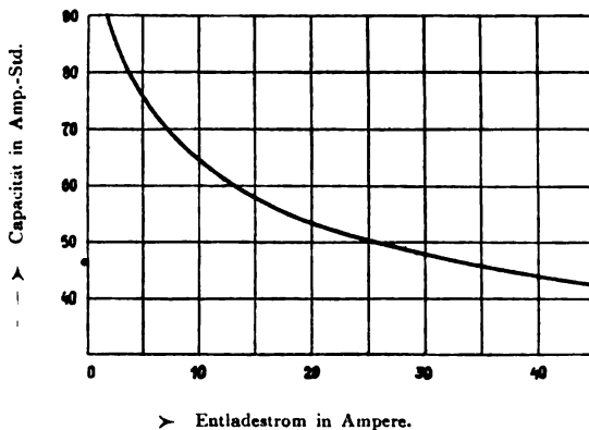
Fig. 111. Abhängigkeit der Capacität vom Entladestrom. Nach Liebenow.
