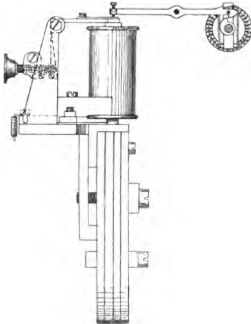
Fig. 235. Elektromagnet und Auslösung der Druckachse.
