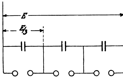
Fig 348. Unterteilte Funkenstrecke.
