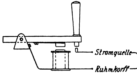
Fig. 353. Funkentelegraphische Taste.
