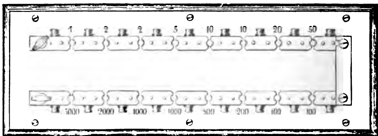
Fig. 278. Widerstandskasten von oben. Alle Stöpsel gezogen.
