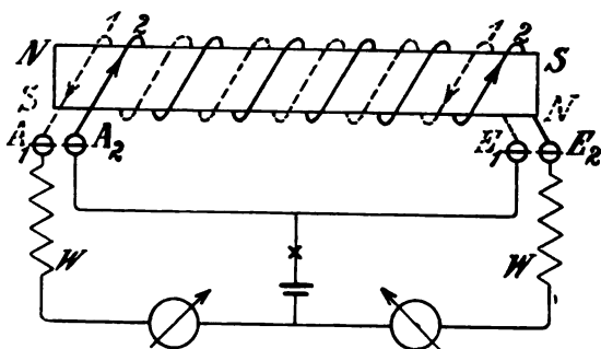
Fig. 276. Prinzip des Differentialrelais.
