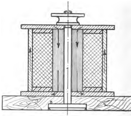
Fig. 262. Ältere Induktanzrolle.
