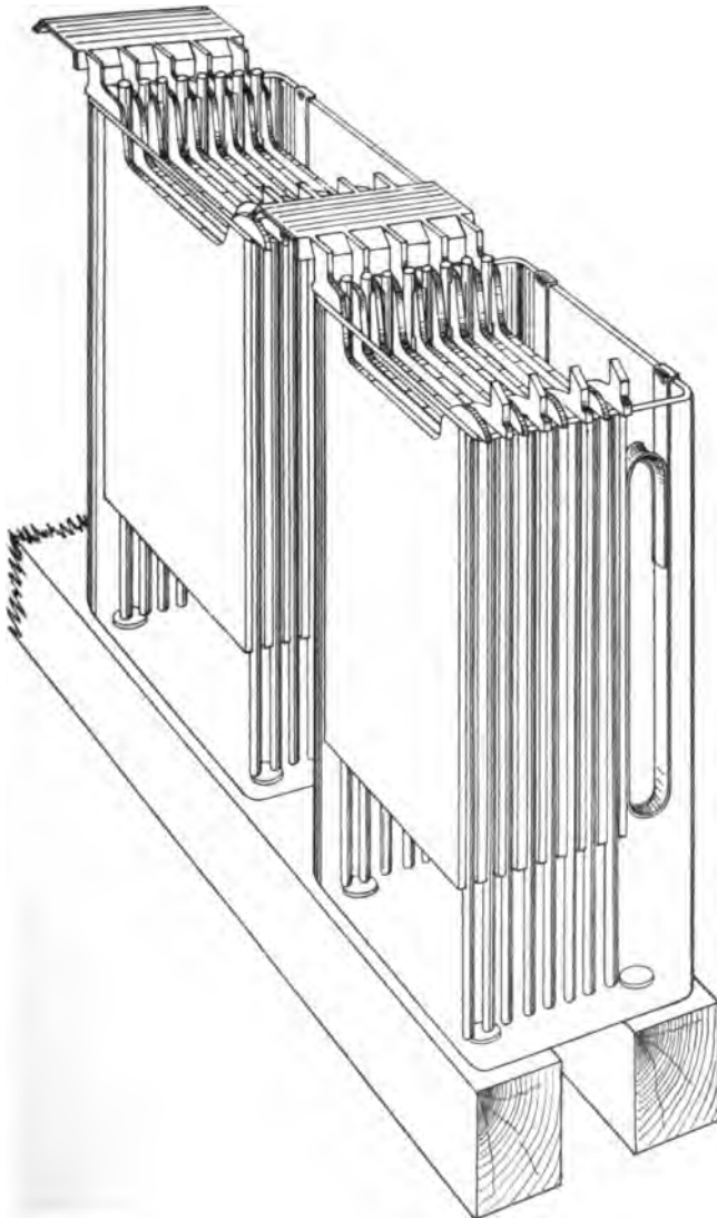
Fig. 118. Zwei hinter einander geschaltete grössere Hagener Zellen.
