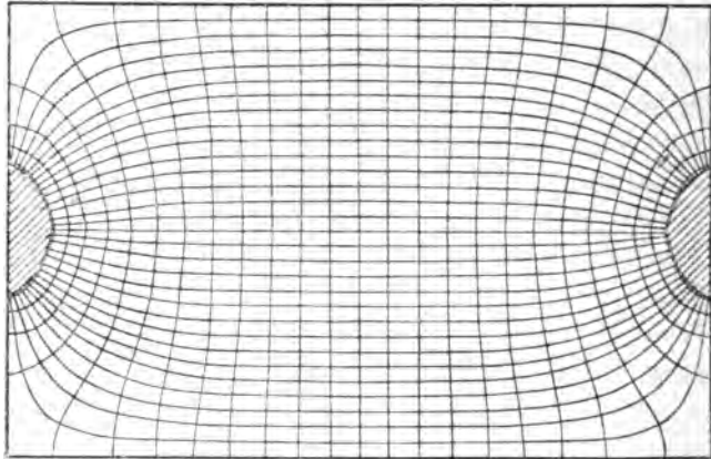
Fig. 287. Strom- und Spannungslinien eines durchflossenen Bleches.
