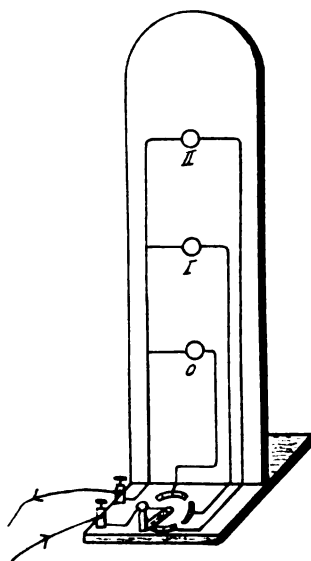
Fig. 4. Modell zur Demonstration des Ohmschen Gesetzes.
