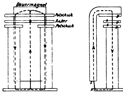
Fig. 317. Wechselstromwecker. Kraftlinienverlauf.
