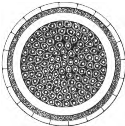
Fig. 300. Papierkabel (Querschnitt).
