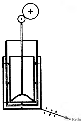
Fig. 64. Ladung der Leydener Flasche.
