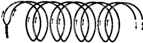
Fig. 49. Schema der bifilaren Wicklung.
