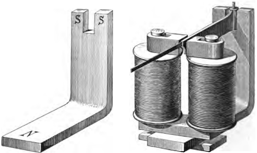
Siemenssches Polarisiertes Relais.
