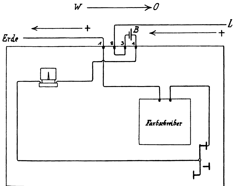
Fig. 215. Ruhestrom-Endstelle.
