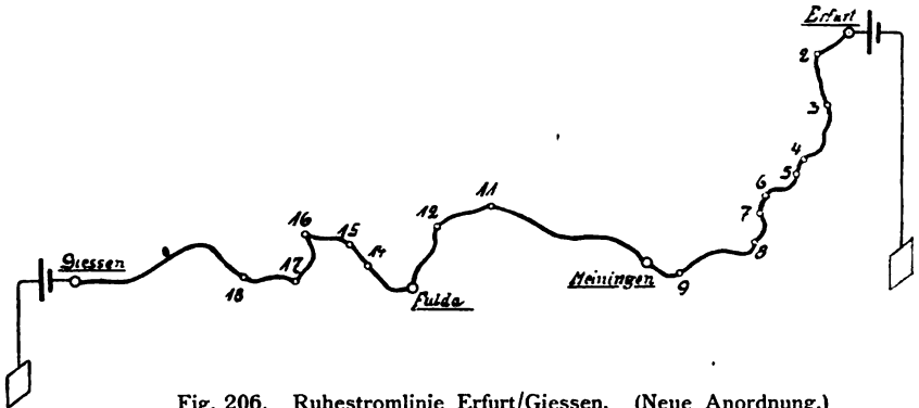
Fig. 206. Ruhestromlinie Erfurt/Giessen. (Neue Anordnung.)
