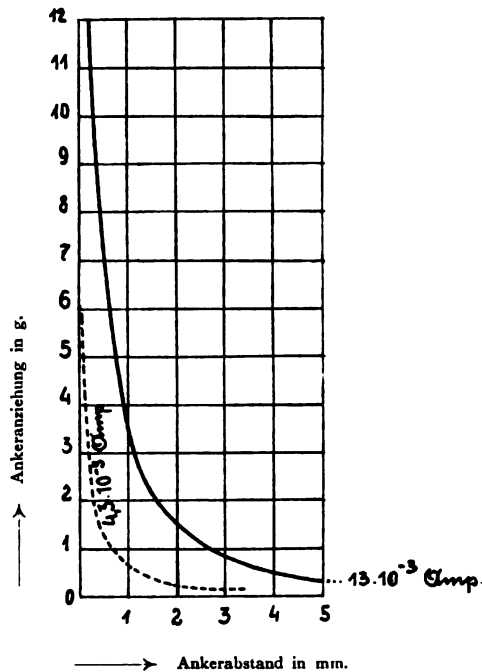
Fig. 145. Ankeranziehung und -abstand.
