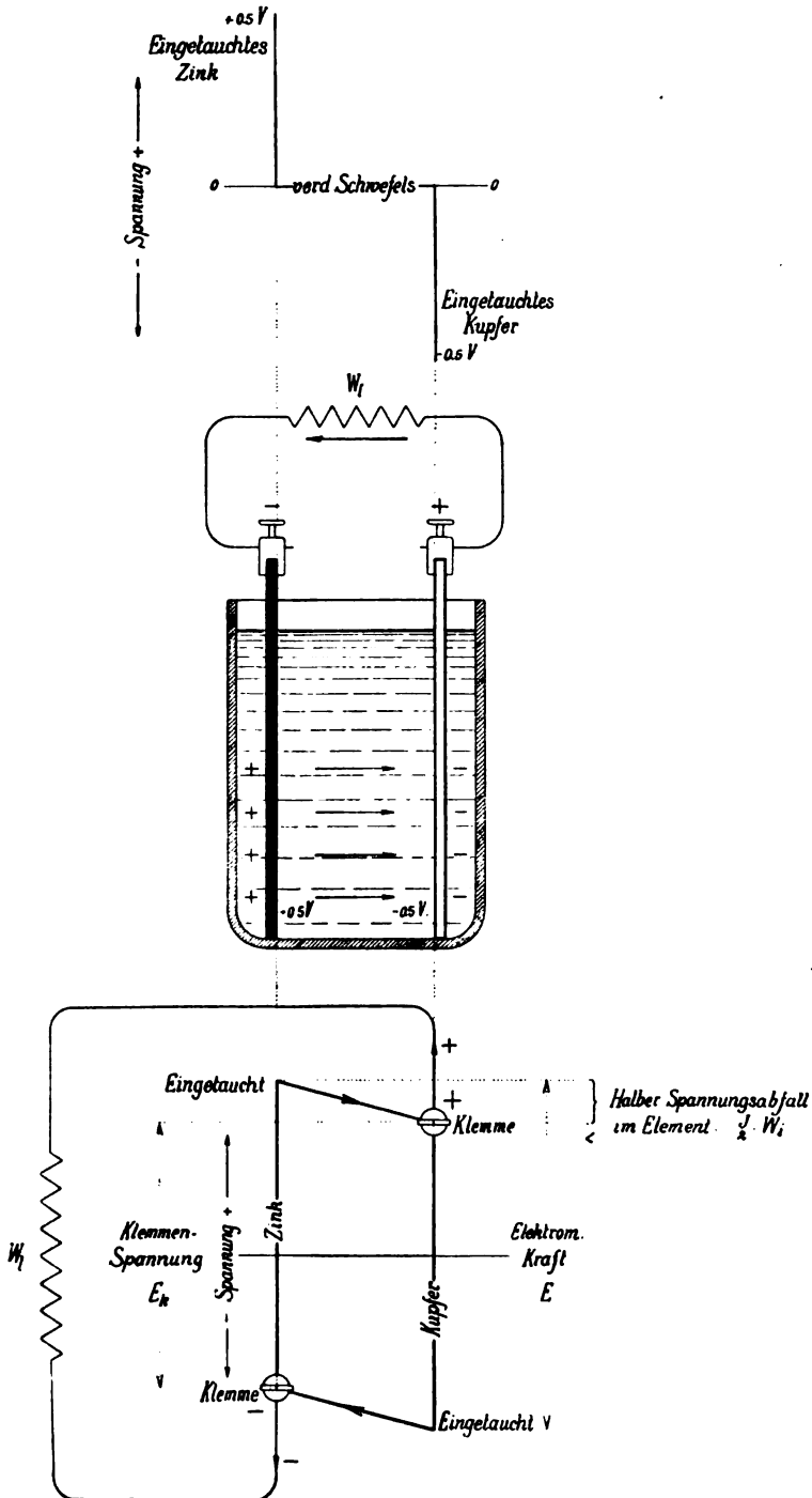
Fig. 83 a, b, c. Spannungssprünge, Stromrichtungen, Klemmenspannungen eines einfachen galvanischen Elementes.
