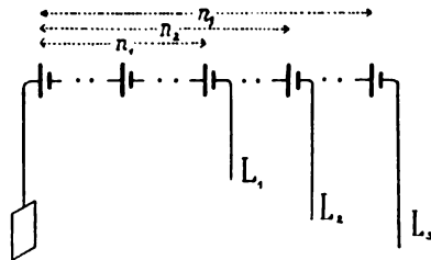
Fig. 194. Mehrere Leitungen verschiedener Länge an einer Batterie.
