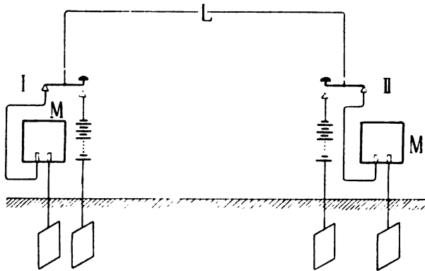
Fig. 166. Einfachste Arbeitsstromschaltung.
