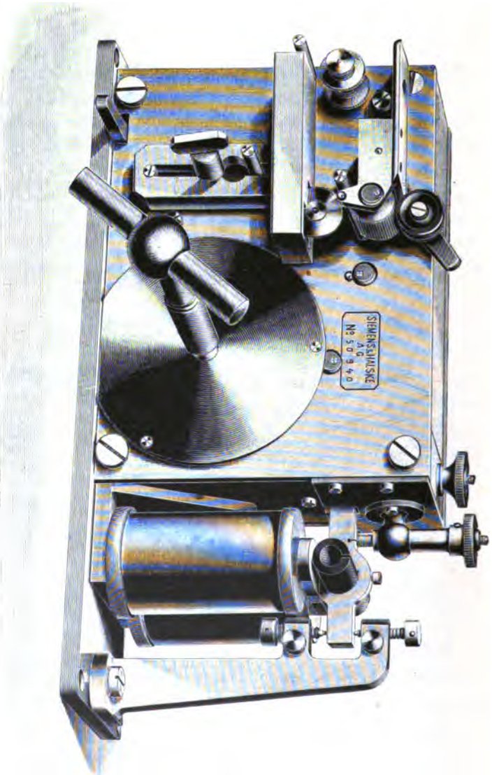
Fig. 141. Deutscher Farbschreiber. ( \frac{1}{2} natürliche GröÙe. Federtrommel im Gehäuse.)
