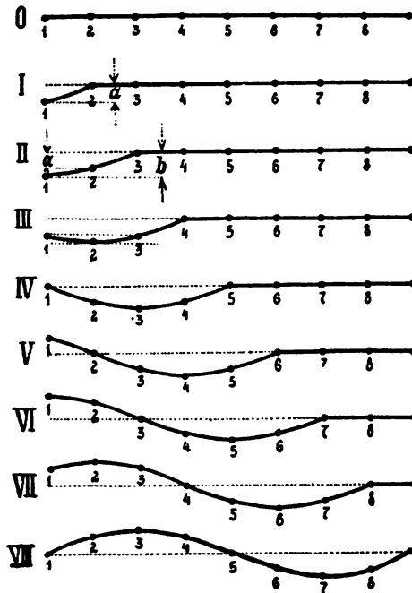
Fig. 121. Zustandekommen einer Seilwelle.
