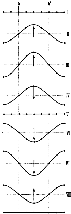
Fig. 127. Stehende Seilwelle.
