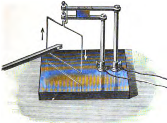
Fig. 27. Umkehrung des Oersted'schen Versuches.
