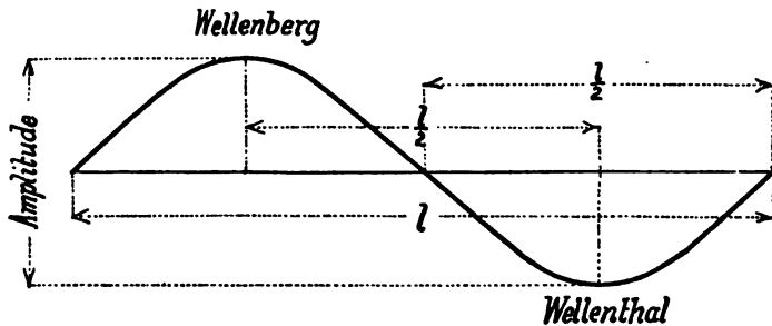
Fig. 122. Wellenlänge l , Wellenthal, Amplitude.
