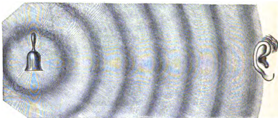
Fig. 131. Verdichtungen und Verdünnungen tönender Luft, schematisch.
