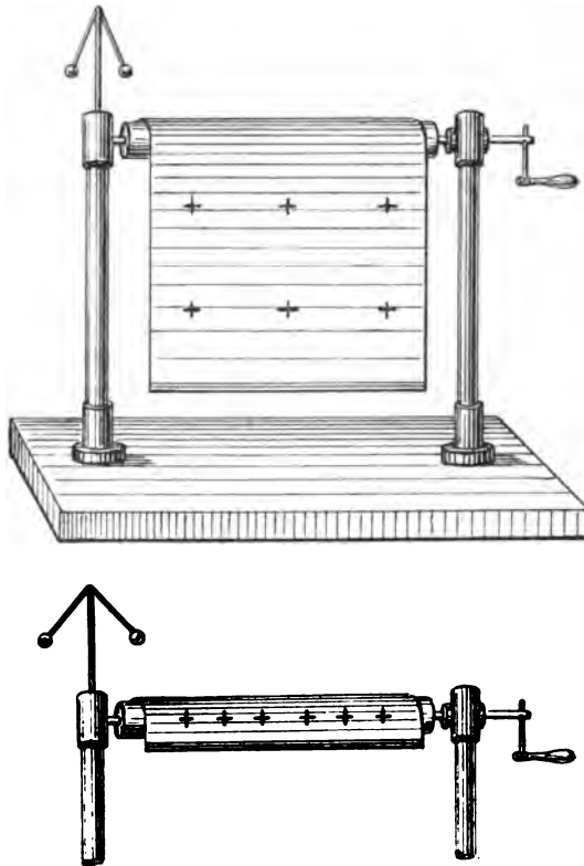
Fig. 60. Faradaysches Rouleau.
