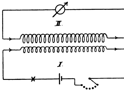
Fig. 46. Voltainduktion.
