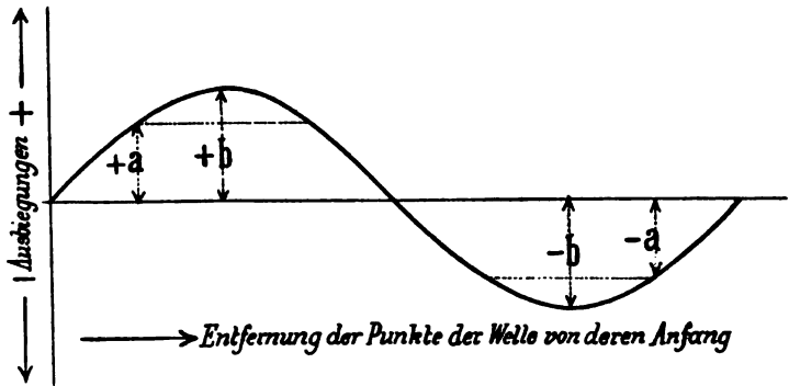
Fig. 123. Welle.
