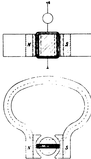
Fig. 270. Drehspulinstrument.
