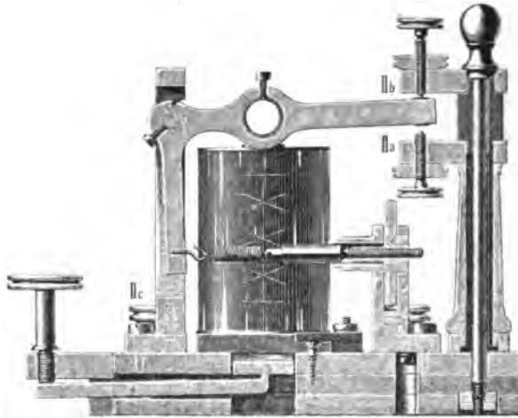
Fig. 179. Weicheisen-Relais.
