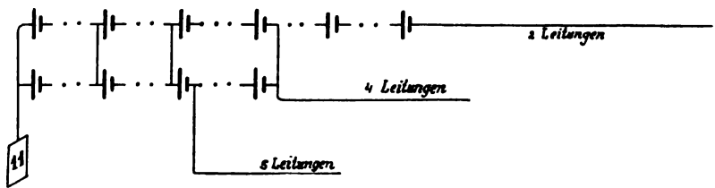
Fig. 197. Verwendung paralleler Zellen in einer Batterie.
