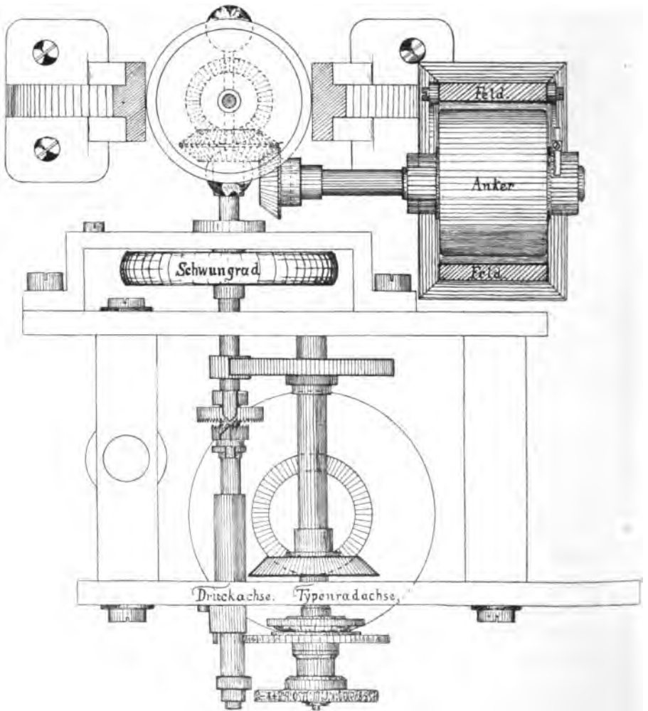
Fig. 238. Wichtigste Teile des Triebwerks.
