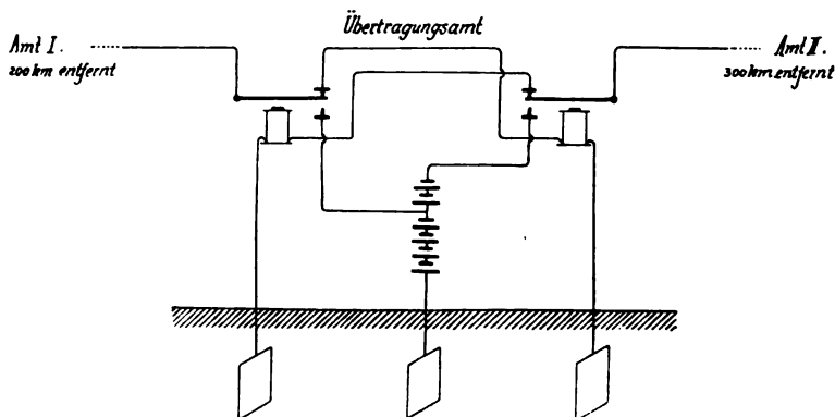
Fig. 189. Übertragung mit zwei Relais.
