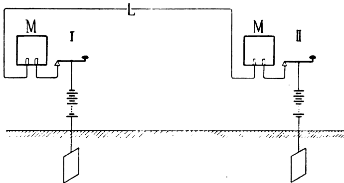
Fig. 167. Einfachste Ruhestromschaltung (nicht verwandt).
