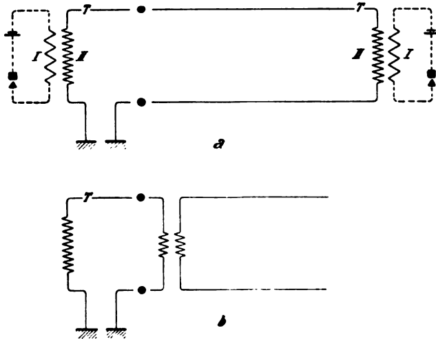
Fig. 298. Verbindung von Doppel- und Einzelleitung. a. direkt. b. durch Übertrager.
