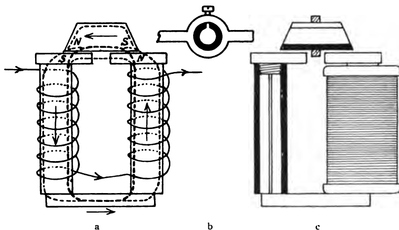
Fig. 143. Farbschreibermagnet.
