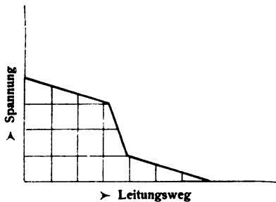
Fig. 6. Spannungsabfall in einer Glühlampe und ihren Zuleitungen.
