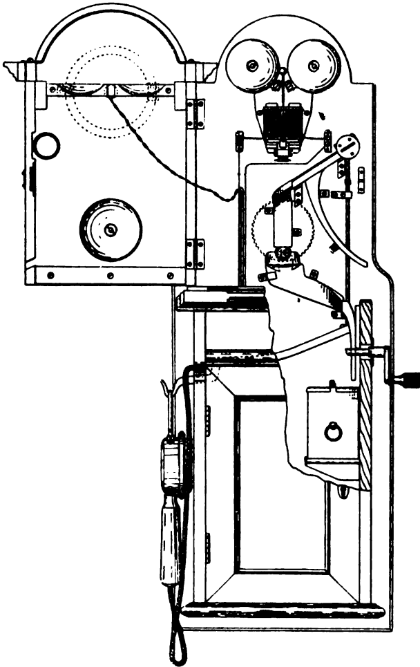
Fig. 334. Fernsprechautomat.
