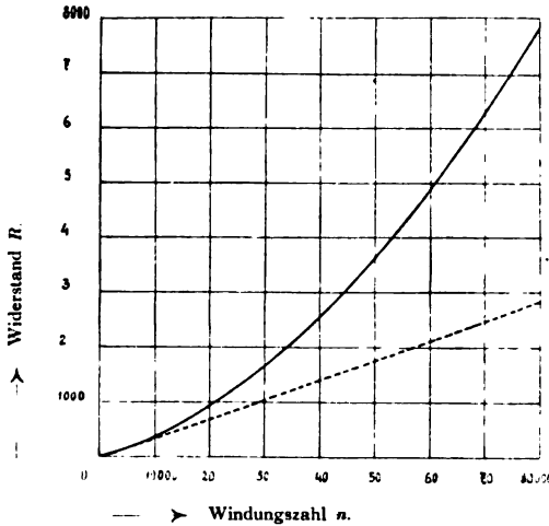
Fig. 146. Widerstand und Windungszahl der Farbschreiberspulen.
