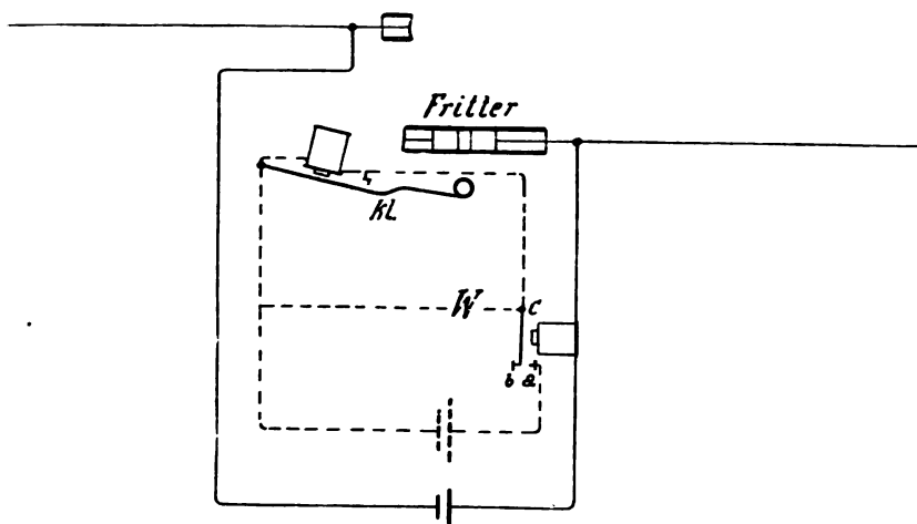
Fig. 341. Entfrittung.
