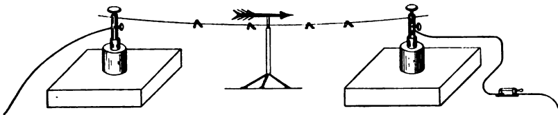
Fig. 1. Demonstration der Wärmewirkung eines elektrischen Stromes.
