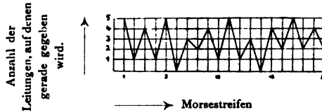
Fig 195. Schwankende Beanspruchung einer Batterie durch gemeinsame Leitungen.
