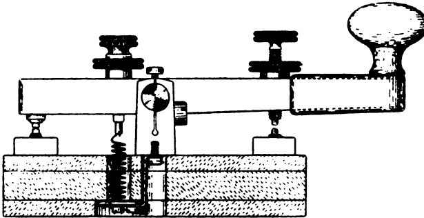
Fig. 158. Taste.
