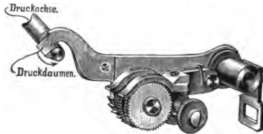
Fig. 242. Druckhebel.
