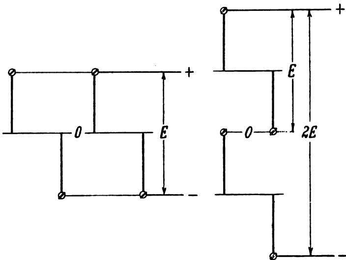
Fig. 100. Diagramm der Elektromotorischen Kraft zweier Elemente.
