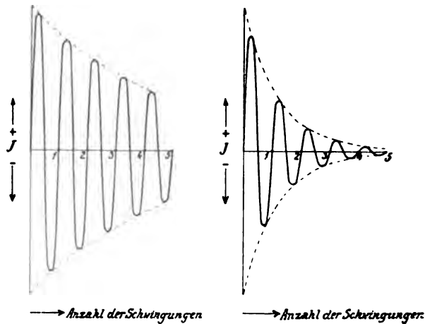
Fig. 346. Dämpfungskurven. Nach Zenneck.
