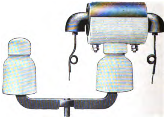
Fig. 305. Pupinspule für Oberleitung. Nach Dolezalek und Ebeling.
