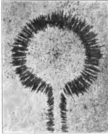
Fig. 35. Kraftlinienbild einer Windung auf einer zu ihr parallelen Ebene.
