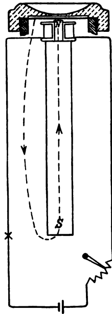
Fig. 284. Telephon mit Stabmagnet.
