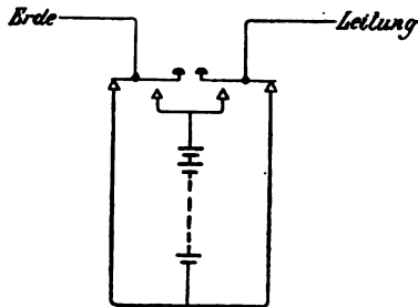
Fig. 266. Prinzip der Doppeltaste.
