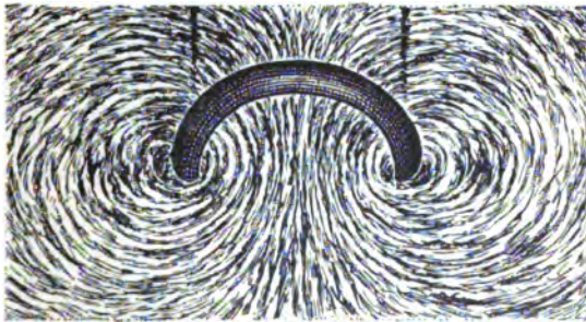
Fig. 34. Kraftlinienbild auf einer eine Windung schneidenden Ebene.
