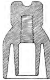
Fig. 202. Porzellandoppelglocke.
