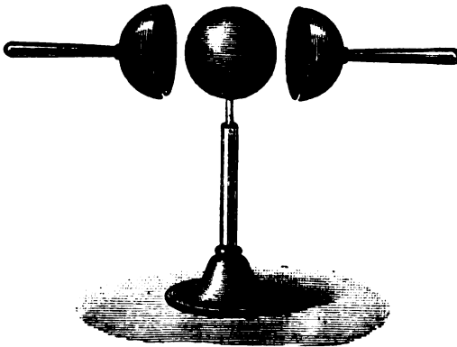
Fig. 61. Zweiter Versuch zum Beweise, dass die statische Elektrizität auf der Leiteroberfläche sitzt.
