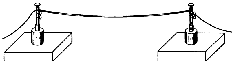
Fig. 12. Platin-Silber-Kette zum Beweise der Abhängigkeit der Wärmeentwicklung vom Widerstande.
