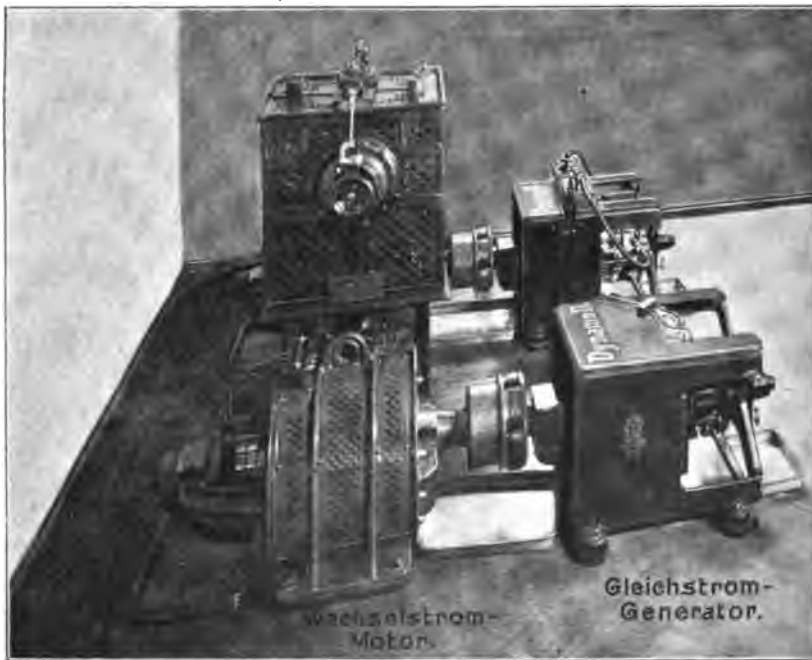
Fig. 201. Motorgeneratoren zur Akkumulatoren-Ladung.
