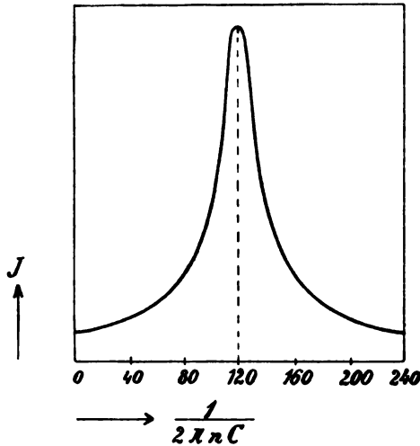
Fig. 349. Resonanzkurve.
