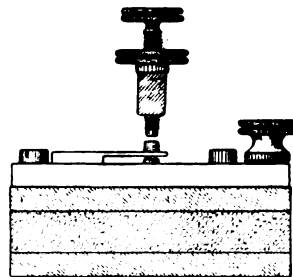
Fig. 159. Federnder Arbeitskontakt.
