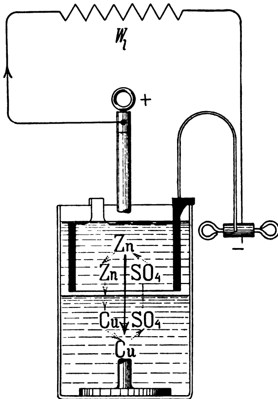
Fig. 91. Arbeitendes Telegraphenelement.
