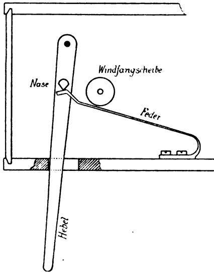
Fig. 153. Auslösung.
