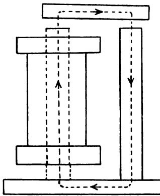
Fig. 41. Schema eines hinkenden Elektromagneten.
