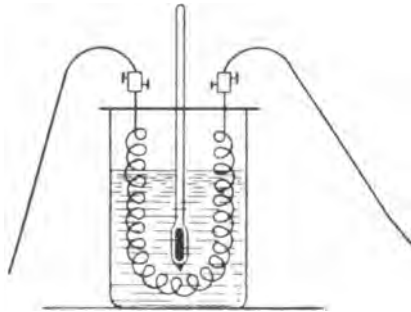
Fig. 11. Versuch zur Bestimmung des elektrischen Wärmeäquivalentes.
