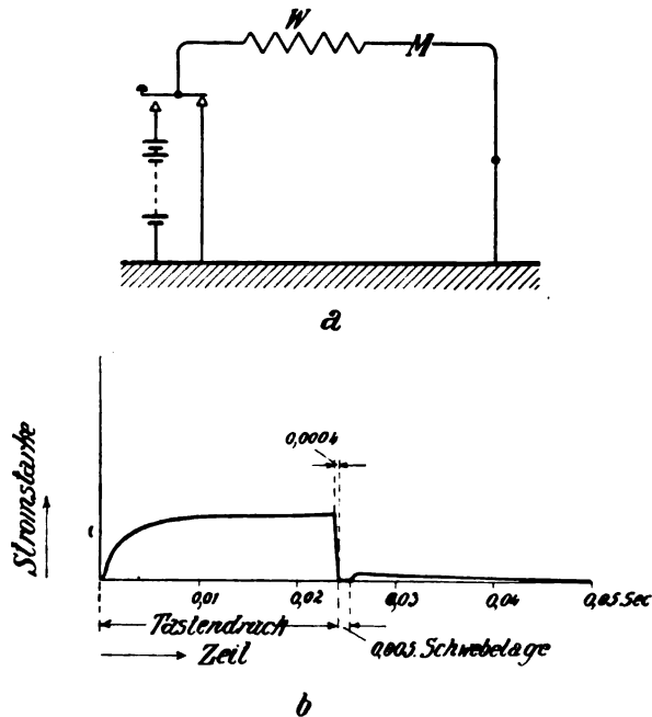
Fig. 249. Zeitlicher Verlauf eines Telegraphierstromes.
