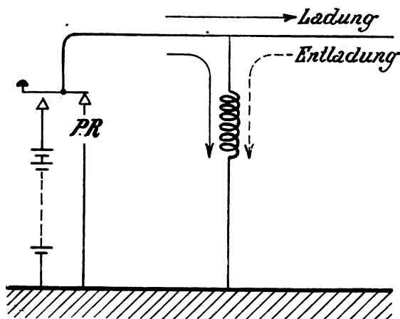
Fig. 261. Wirkung einer Induktanzrolle.
