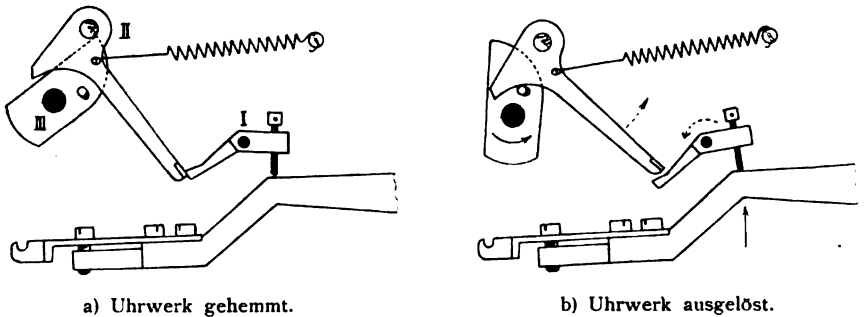
Fig. 154. Selbstthätige Auslösung.
