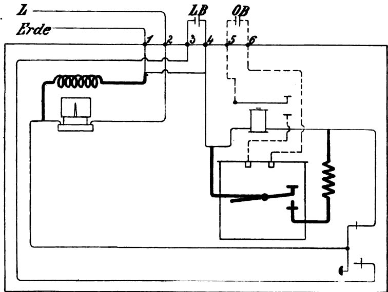
Fig. 260. Endstelle mit Induktanzrolle und unmittelbarer Erdung.
