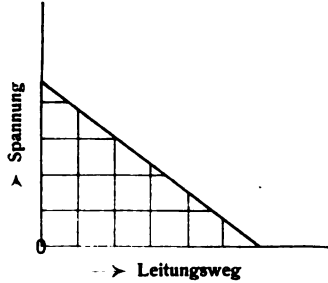
Fig. 5. Spannungsabfall in einem Leiter von gleichmäßigem Widerstande.
