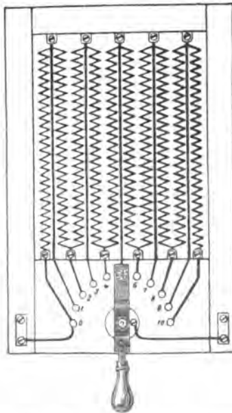
Fig. 26. Regulierwiderstand.
