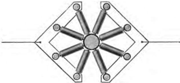
Fig. 312. Englischs Walzenmikrophon. Nach Crotch.
