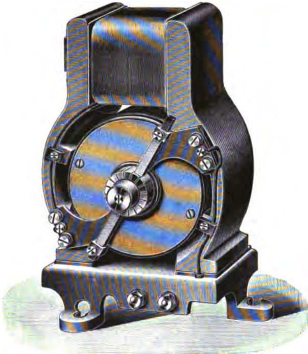
Fig. 236. Gleichstrommotor.
