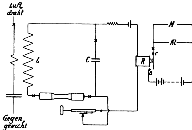
Fig. 358. Empfangsschaltung.
