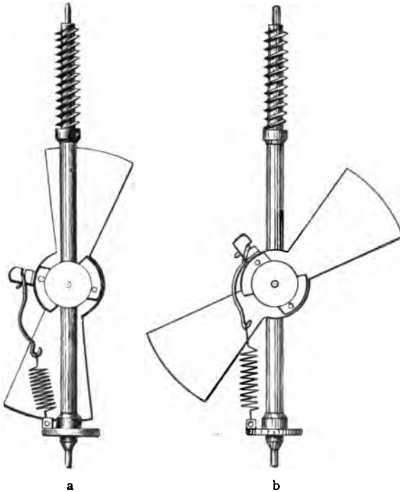
Fig. 152. Windfang. Natürliche Grösse.
