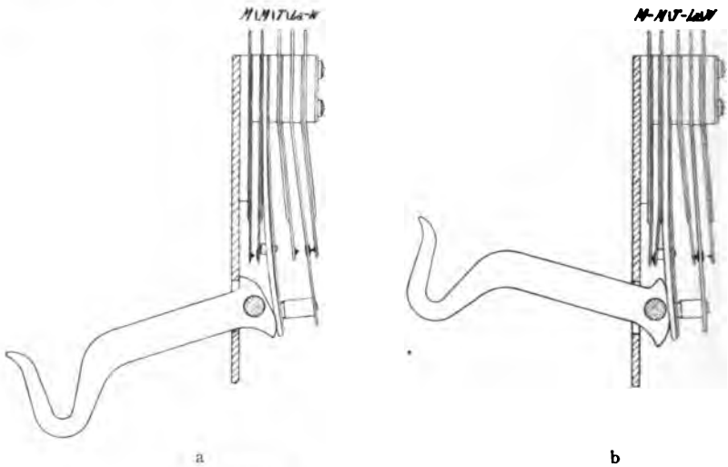
Fig. 323. Neuer Umschalter.
