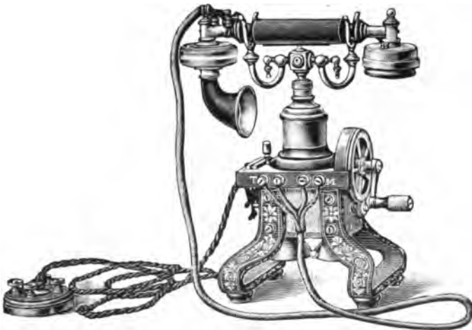
Fig. 330. Schwedisches Tischgehäuse. Von Ericsson.
