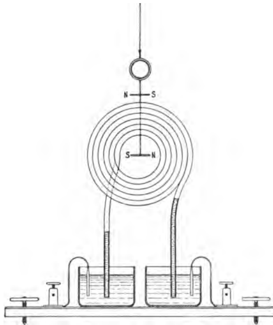
Fig. 80. Elektrolytisches Galvanometer.
