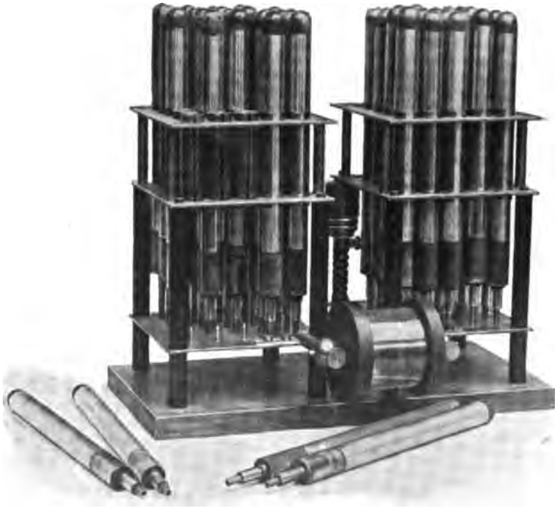
Fig. 354. Leydener Flaschen.
