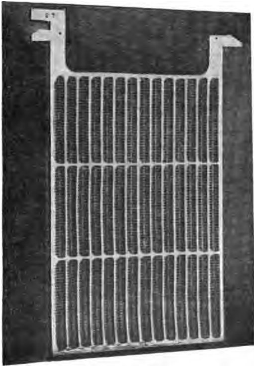
Fig. 105. Gitter der Kölner Akkumulatorenwerke.
