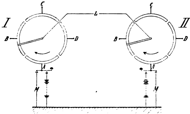
Fig. 274. Baudotprinzip.
