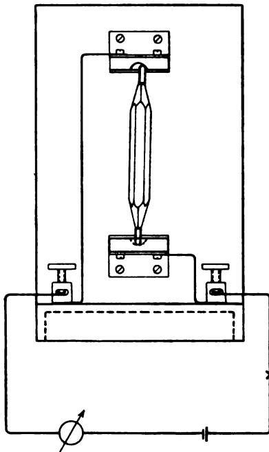
Fig. 286. Mikrophonmodell.
