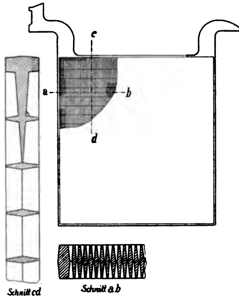
Fig. 108. Positive Hager Plate. (Platte \frac{1}{4} , Schnitte annähernd \frac{1}{1} .)
