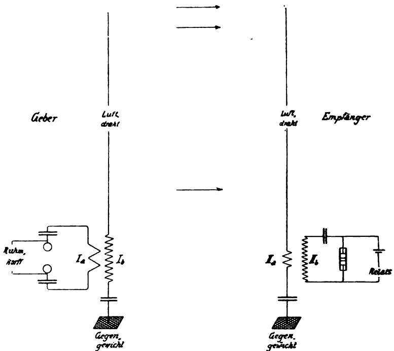
Fig. 351. Prinzipielle Schaltung.
