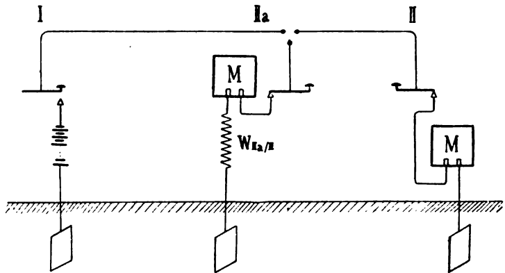
Fig. 172. Anwendung eines Ausgleichswiderstandes.
