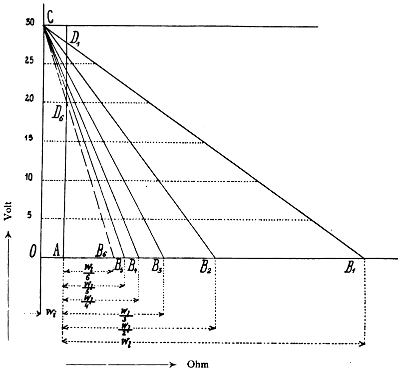
Fig. 196. Abnahme der Klemmenspannung einer Batterie durch Speisung mehrerer paralleler Leitungen vom gleichen Widerstande w_l .
