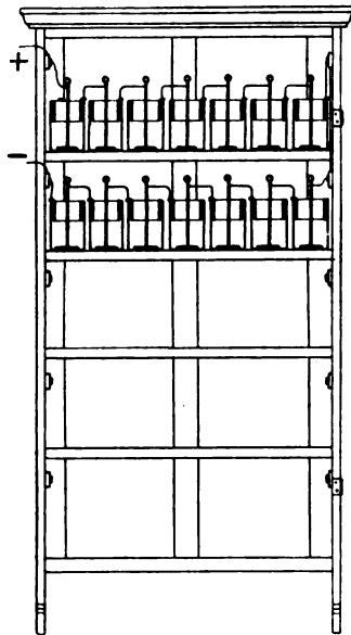
Fig. 192. Elementenschrank.
