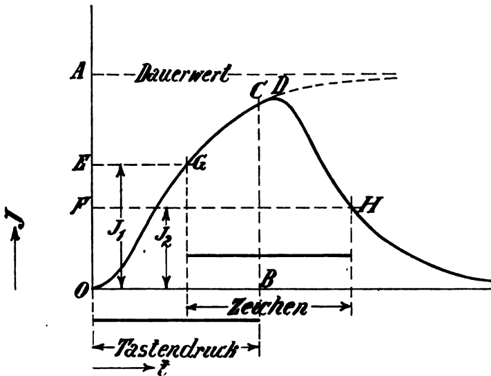
Fig. 256. Telegraphierstrom am Leitungsende. Schematisch. Nach Thomas.
