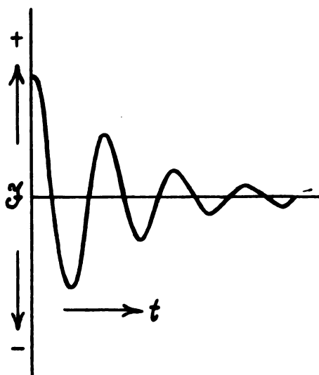
Fig. 59. Diagramm des Funkens.
