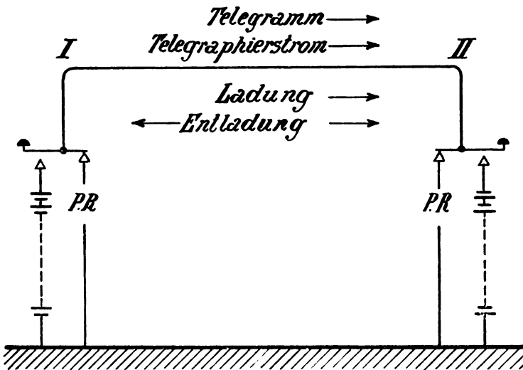
Fig. 259. Entgegengesetzte Klemmenschalung.
