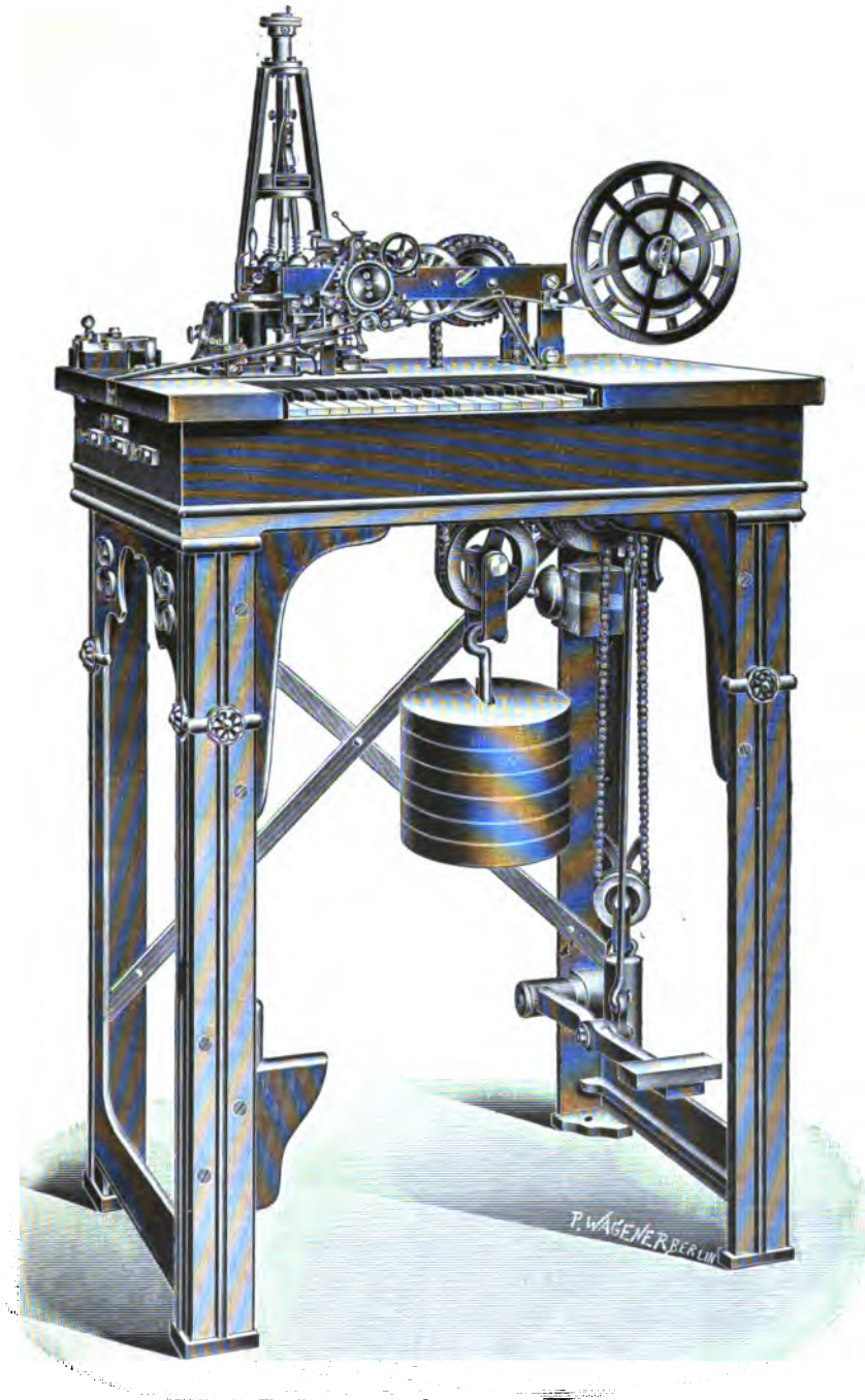
Fig. 220. Hughes-Apparat mit Gewichts- und elektrischem Antrieb.
