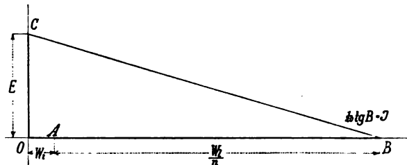
Fig. 102. Stromlieferung n hintereinander geschalteter Elemente.
