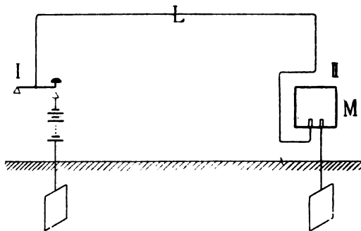
Fig. 165. Einfachste Morseschaltung (nicht verwandt).
