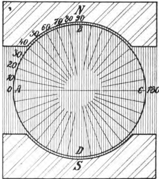
Fig. 318. Drahtwindung im Magnetfelde.
