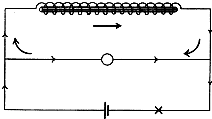
Fig. 48. Selbstinduktion einer Eisen-erfüllten Spule.
