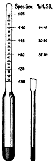
Fig. 112 Akkumulatoren- Aräometer.
