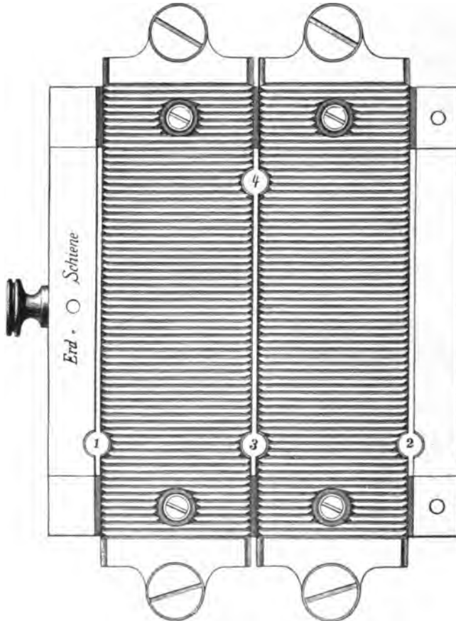
Fig. 175. Tischblitzableiter, Deckelplatte abgehoben.
