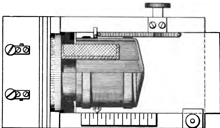
Fig. 263. Induktanzrolle mit verschiebbarem Eisenpilz.
