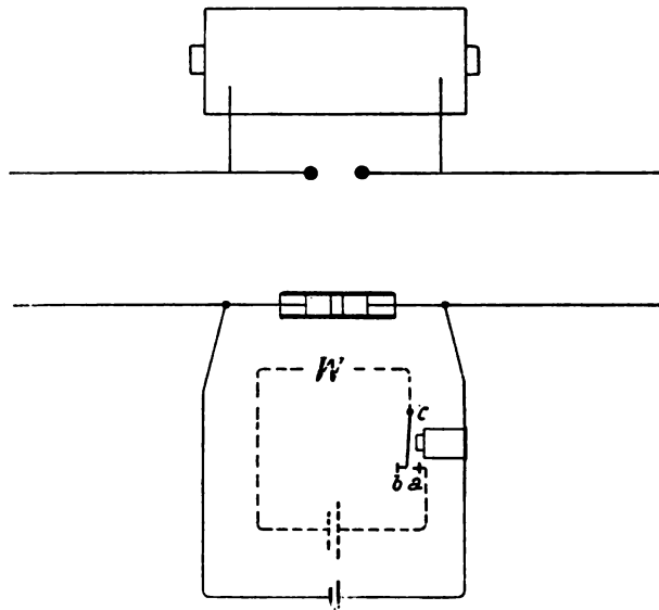
Fig. 339. Empfang elektrischer Wellen mit Fritter und Relais.
