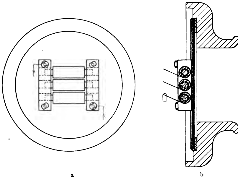
Fig. 289. Walzenmikrophon.
