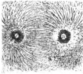
Fig. 39. Kraftlinienbild benachbarter ungleichnamiger Magnetpole.
