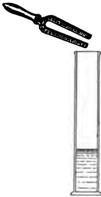
Fig. 136. Resonanz einer Luftsäule bestimmter Länge auf eine Stimmgabel.
