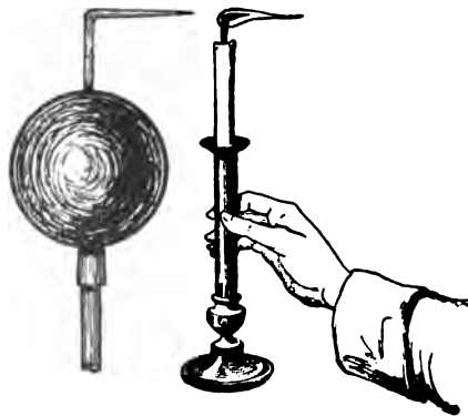
Fig. 62. Spitzenwirkung.
