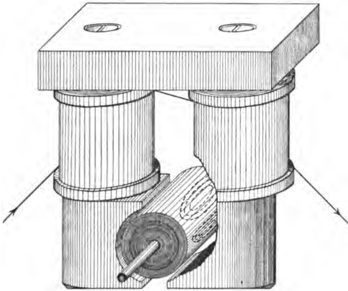
Fig. 47. Induktion von Wirbelströmen.
