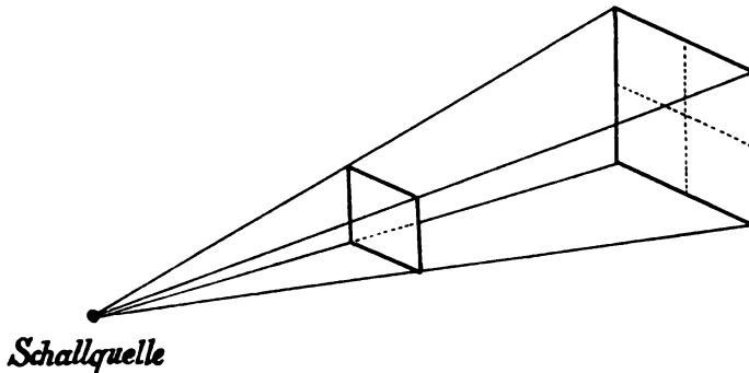
Fig. 133. Die Schallintensitäten verhalten sich umgekehrt wie die Quadrate der Entfernungen von der Schallquelle.
