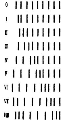
Fig. 130. Längswelle.
