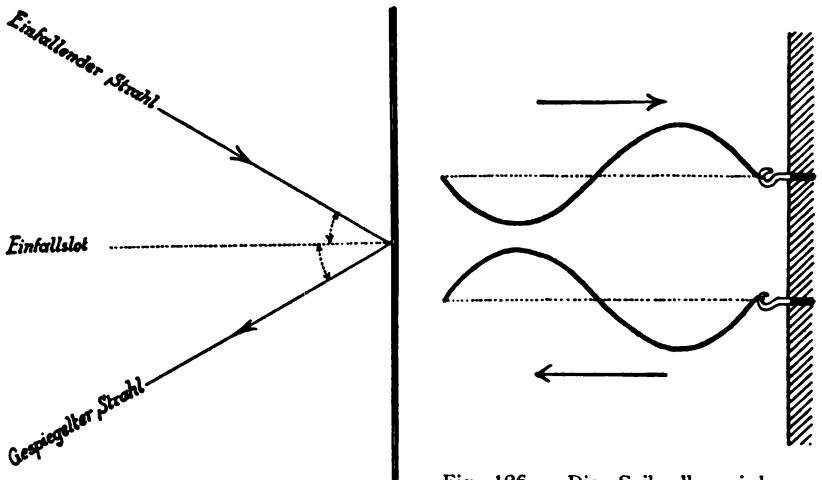
Fig. 126. Die Seilwelle wird vom Wandhaken, um eine halbe Periode verschoben, zurückgeworfen.
