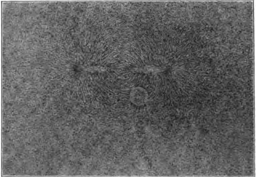
Fig. 24. Magnetstab und Eisenstäbe.
