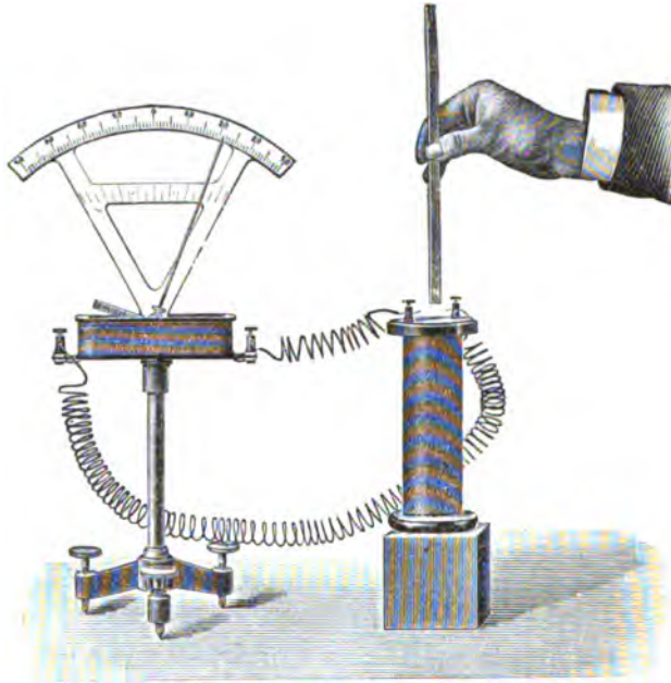
Fig. 45. Magnetinduktion. 1)
