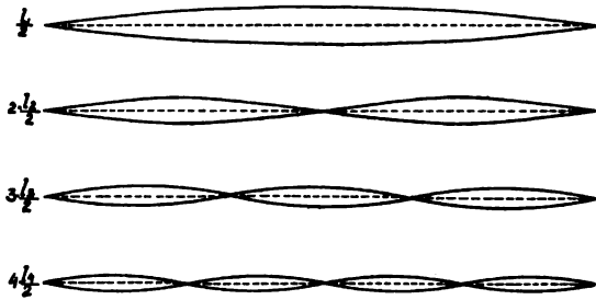
Fig. 129. Stehende Wellen verschiedener Länge auf einem Seil.
