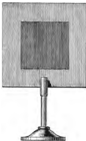
Fig. 65. Franklinsche Tafel.
