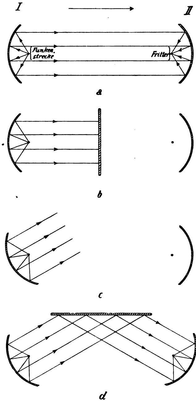
Fig. 340. Spiegelung elektrischer Wellen.
