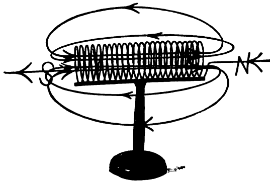
Fig. 38. Modell der Kraftlinien einer Spule.
