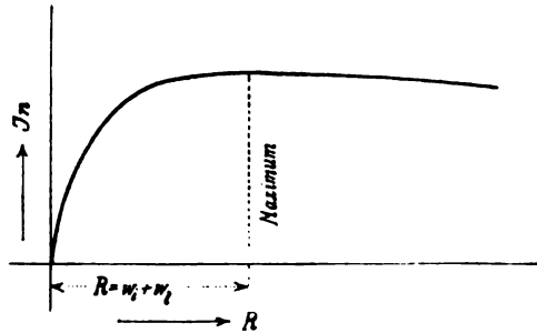
Fig. 147. Widerstand und Amperewindungen.
