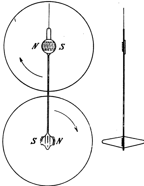
Fig. 268. Kabelgalvanometer.
