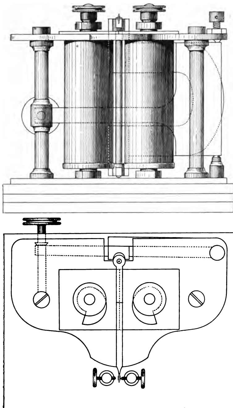
Fig. 186. Relais mit drehbaren Kernen.
