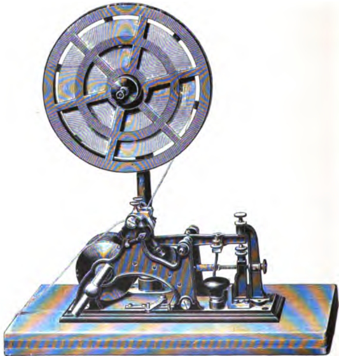
Fig. 140. Übungsapparat.
