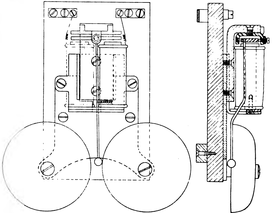
Fig. 316. Wechselstromwecker.
