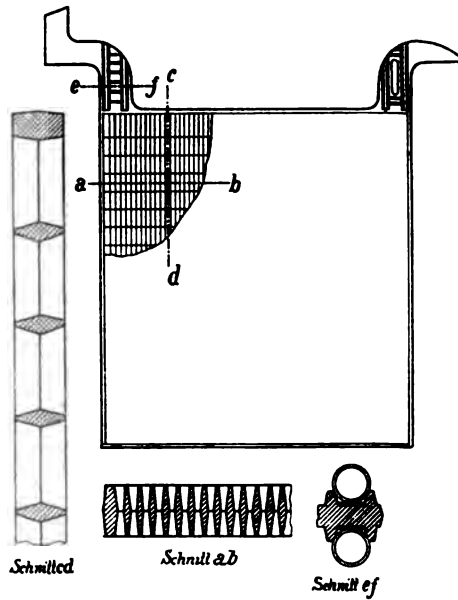
Fig. 109. Negative Hager Plate. (Platte \frac{1}{4} , Schnitte cd und ab annähernd \frac{1}{1} , ef \frac{1}{2} .)
