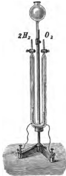
Fig. 79. Hofmannscher Apparat.
