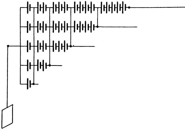
Fig. 198. Batterie in Leiterschaltung.
