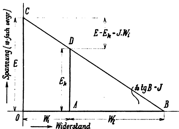
Fig. 82. Ohmsches Gesetz auf galvanische Elemente angewandt.
