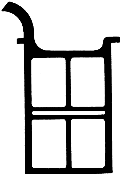
Fig. 106. Bösesches Gitter mit Schlitz.
