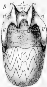
Fig. 433. Glyptoceras sphaericum Mart. Subcarbon. Rätigen b. Düsseldorf. Schale gegen die Septalfäche gesehen. el = Aussen-, sl = Seitenlobus; isl = innerer Seitenlobus; il = Innenlobus; ms = Mittelsattel; es = Aussensattel; is = Innensattel; u = Septalumschlag; si = Siphon.
