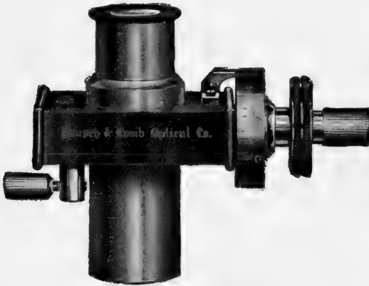
FIG. 71.—Filar Micrometer.
