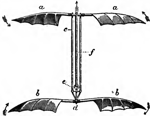
FIG. 38.—Hélicoptère or Screw-Model, by Pénaud.
