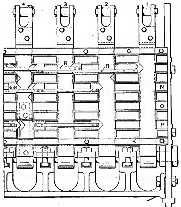
FIG. 7.—Interlocking Frame.
