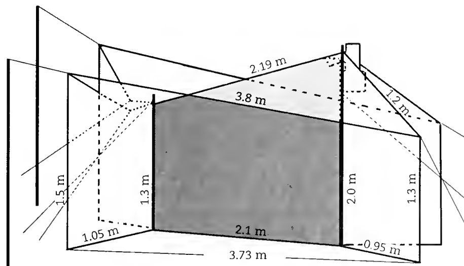
6. Schema of the redesigned Malaise trap. 6. Schema van de nieuw ontworpen Malaiseval.
