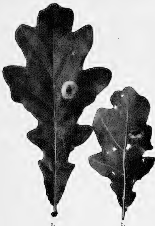
Fig. 1. Ekblad med blotch-mine af Lithocolletis sp.; a. från öfre, b. från undersidan; i midten ses den med ekkrement klädda kokongen. \frac{1}{1} . Förf. foto.
