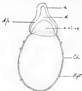
Fig. II. Ovariallägg af Ephemereida ignita Pod., subim., visande den längre, toppmösslika formen af epithema ( Afs ). Öfvervägande konturbild. Motsvarande beteckningar som i figg. 5 och 7 å Taf. I. Förstor. \times 150 .
