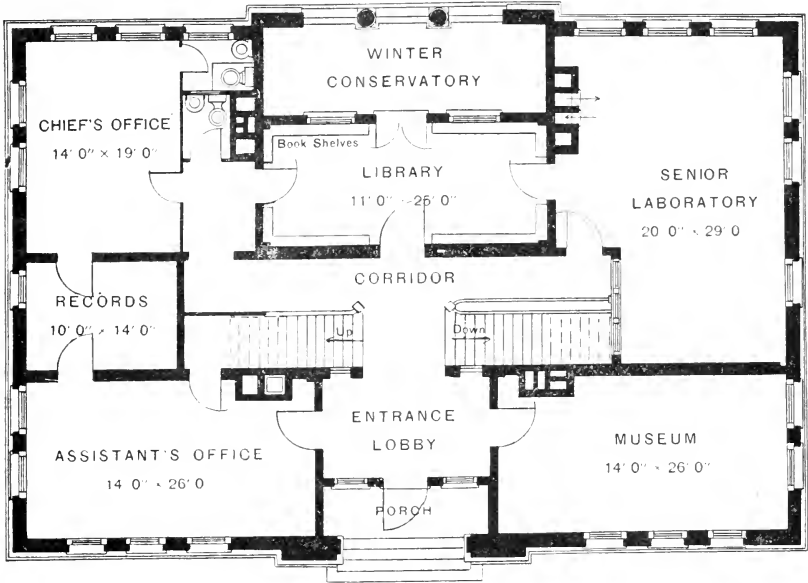
FIG. 3.—First-floor plan.
