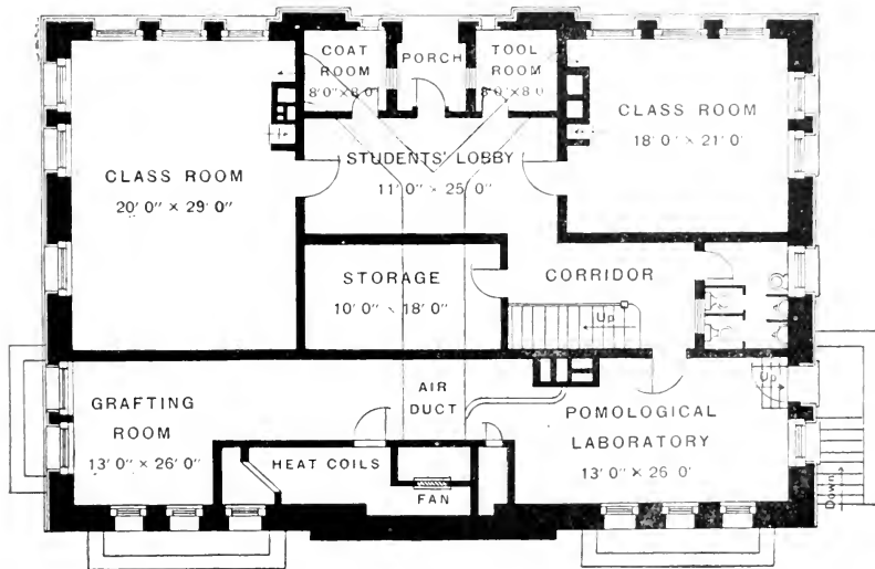
FIG. 2.—Basement plan.
