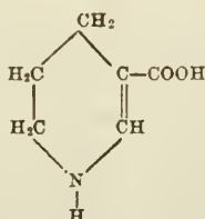
Isoguvacin C_6H_9NO_2 .
