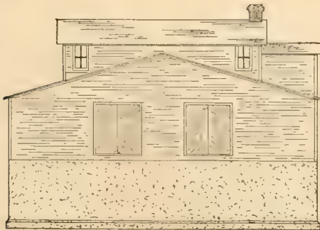
END ELEVATION
