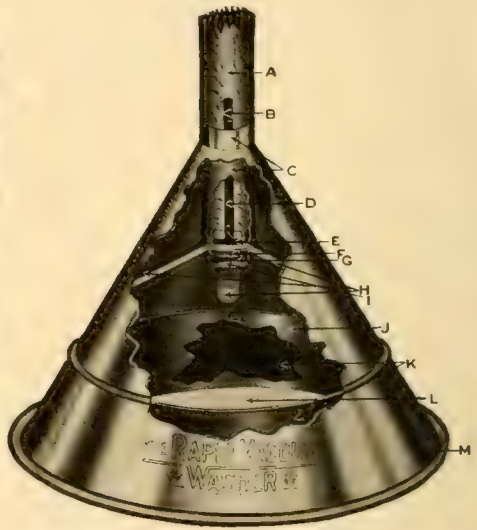
Fig. 2.—Hand Washer
