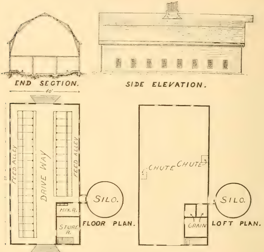
Fig. 1.—Dairy Barn.
