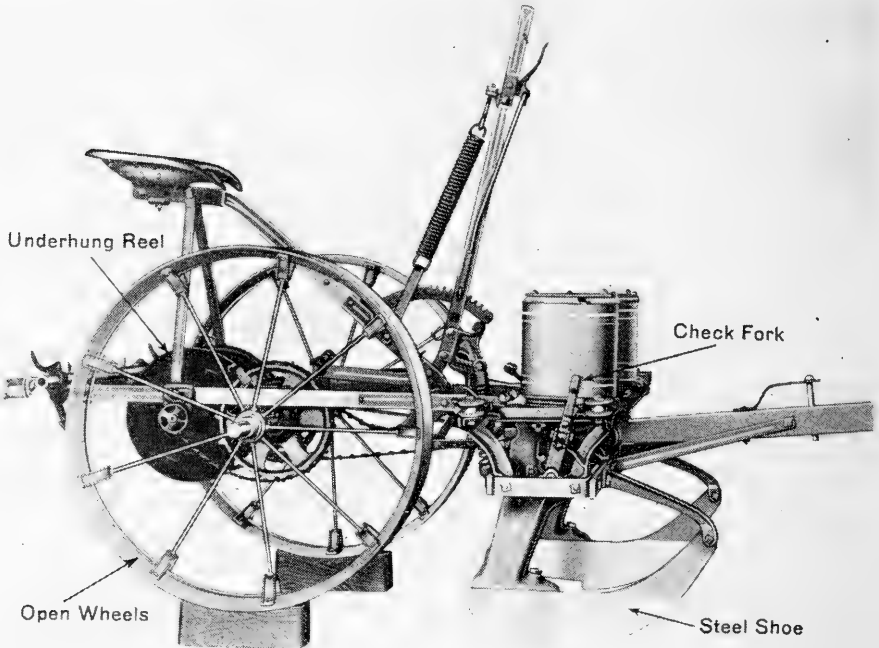
FIG. 320. Corn planter.
