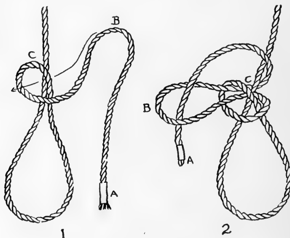
FIG. 383. Manger knot.
