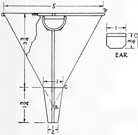
FIG. 286. Funnel.
