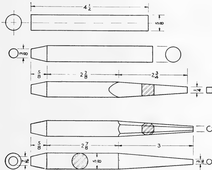
FIG. 222. Punches.
