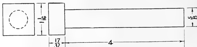
FIG. 188. Machine bolt.
