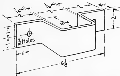
FIG. 228. A lighter stake-iron.
