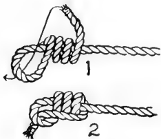
FIG. 373. Stevedore knot.
