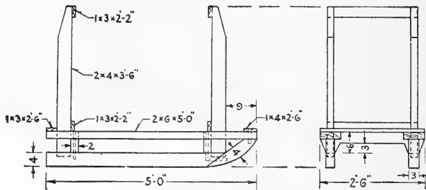
FIG. 135. Farm sled.
