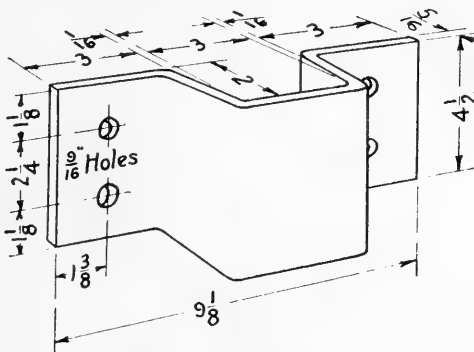
FIG. 227. Wagon-box stake-iron.
