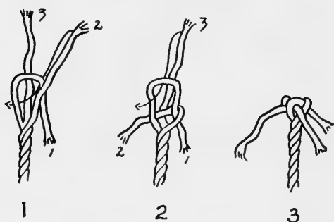
FIG. 364. Crown knot.
