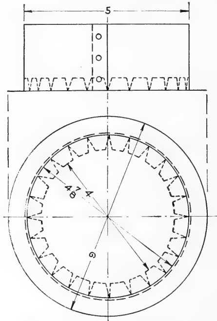
FIG. 294. Stovepipe collar.
