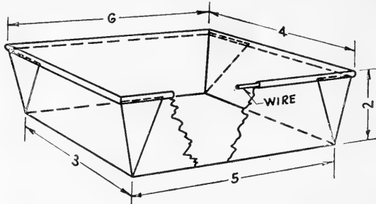
FIG. 275. Drip pan.
