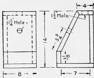
FIG. 123. Egg tester.
