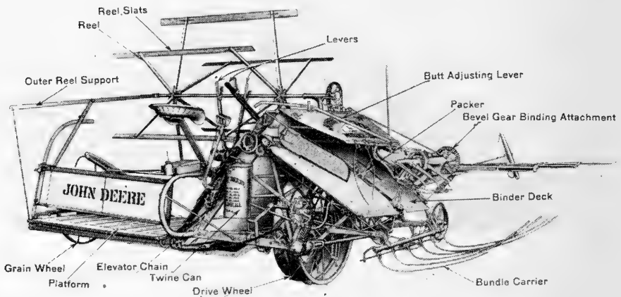
FIG. 324. Grain binder.
