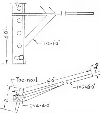
FIG. 129. Garden marker.
