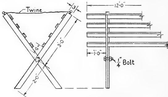
FIG. 125. Tomato trellis.
