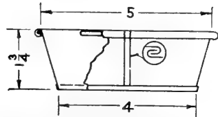
FIG. 287. Flaring pan.
