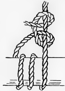
FIG. 390. Rolling hitch.
