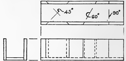
FIG. 80. Miter box.
