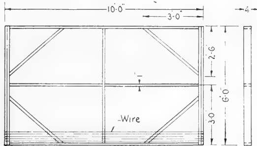
FIG. 121. Corn drier.
