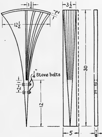
FIG. 9. Flower trellis.
