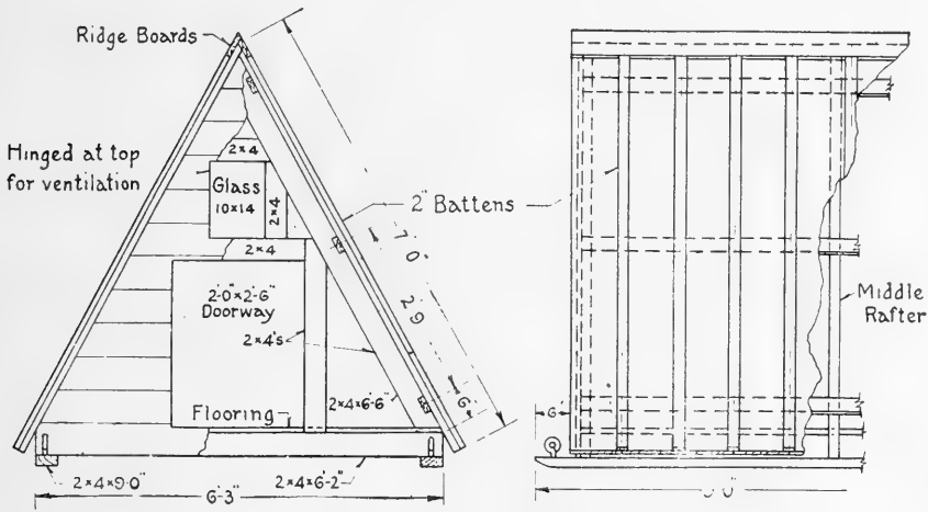
FIG. 130. Hog cot.
