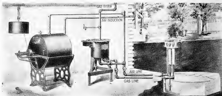
FIG. 339-a. Gasoline gas generator.
