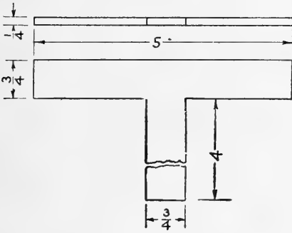
FIG. 205. "T"-weld.
