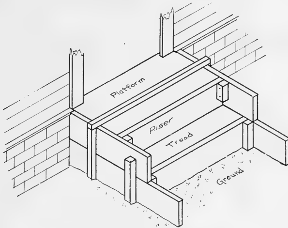
FIG. 149-a. Doorstep form.
