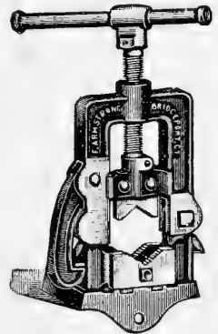
FIG. 344. Pipe vise.
