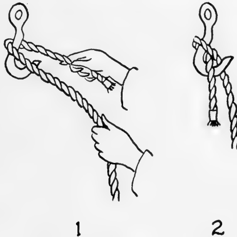
FIG. 393. Blackwall hitch.
