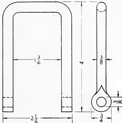
FIG. 187. Punched screw clevis.
