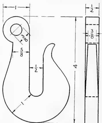
FIG. 189. Log hook.
