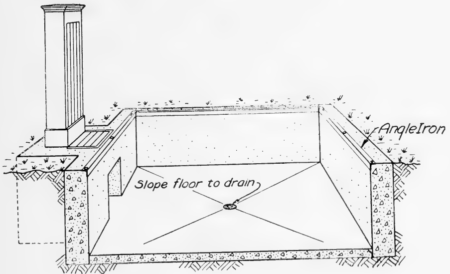
FIG. 163. Scale pit.
