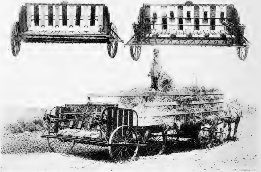
FIG. 322. Straw spreader.
