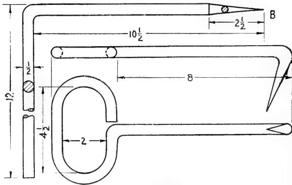
FIG. 178. Hay hook.
