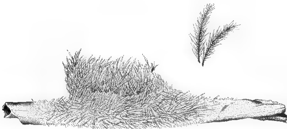
Fig. 27 bis. Cocon d' Euchromia folletii (Guérin-Méneville).
