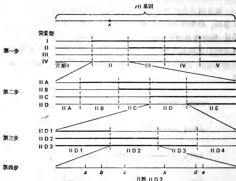
图 8-23 通过在 rII 基因内的各种部位上进行点突变型和缺失突变型的杂交实验，测知点突变发生在什么位置上。第一步，突变型 x 能跟突变型 II、III、IV 杂交而形成正常的重组体，跟 I 就不能。这意味着 I 的缺失包含 x 。因此突变 x 理应存在于染色体片断 II 上。第二步，使突变型 x 跟其他末端包括 II 区的缺失突变型杂交。如果这时只跟突变型 IID 形成正常重组体，那末突变体 x 应存在于染色体片断 IID 上。第三步，用同样方法测出突变型 x 存在于 IID2 部位。尽管已知其他点突变型 ( a, b, \dots ) 也发生在这个小小的范围内。
