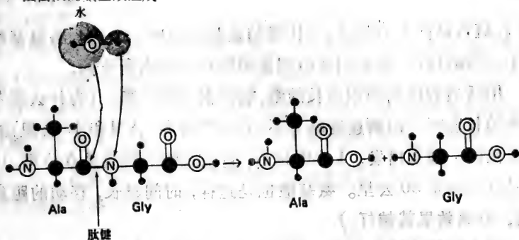
图 5-5 构成蛋白质的氨基酸之间的肽键，能由水解切断。也就是加入水的组分 \text{H}^+ 和 \text{OH}^- 使肽键切断。肽键的水解反应完全是肽键生成反应的逆反应(图 5-2)。蛋白质水解，要使它能在酸里煮沸或者跟蛋白酶作用。
