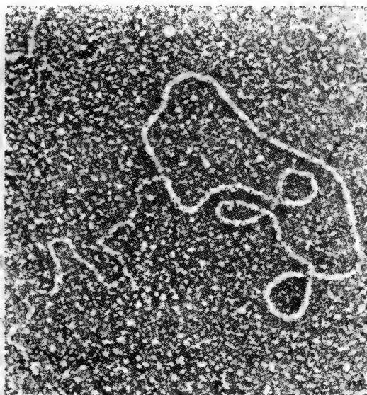
图 8-15 复制中的 \phi X 174 噬菌体的 DNA。在双链的滚环上拖有一条单链的尾部。随着裸露的滚环部分被合成新的互补的 DNA，单链的延长尾部剥落并切成适当的长度。当外面被蛋白质包裹后就成为子代噬菌体粒子。(感谢戴维·德雷斯勒)
