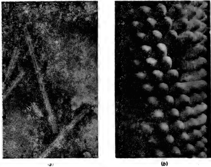
图 9-16 这种棒状的病毒是烟草花叶病的病原。(a)烟草花叶病毒的电镜照片。象纵向断片那样，棒状病毒的内芯孔道是相通的。(感谢加里福尼亚大学病毒研究所)(b)烟草花叶病毒的模型。相同的蛋白质亚单位排列呈螺旋状，它的内侧盘绕着 RNA。(感谢 D. L. D. Caspar 和 A. Klug)
