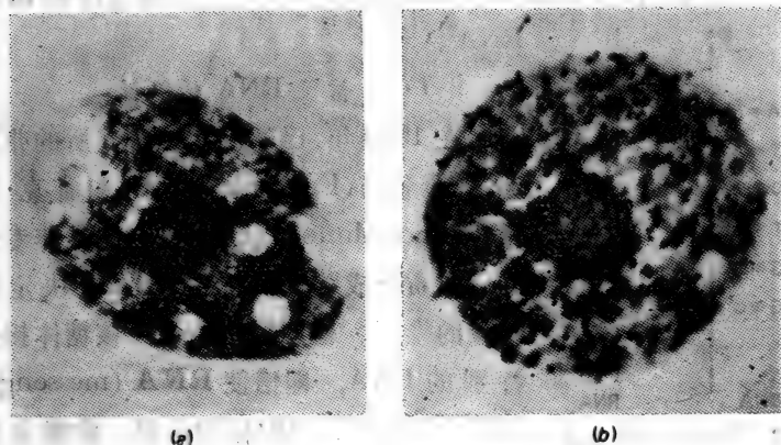
图9-2 本实验证实RNA在细胞核里合成,再转移到细胞质里。(a)使细胞跟RNA的一种成分的放射性标记的胞苷接触15分钟后的放射自显影图。(b)使细胞跟放射性标记的胞苷接触12分钟后再跟无放射性的胞苷接触88分钟的放射自显影图。(a)在15分钟时间内,大部分的RNA合成发生在细胞核里。(b)在跟无放射性的胞苷接触的88分钟内,大部分RNA转移到细胞质里。(据D. M. Prescott, Prog. Nucleic Acid Res. , III: 35(1964), 并向作者致谢)
