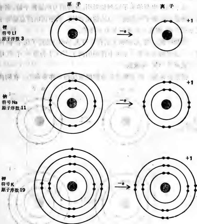
图2-7 锂、钠、钾是最外电子层上有一个电子的元素,失掉这个电子,它们的原子就有稀有气体那样的稳定电子结构。这时它们带一个正电荷。失去电子或者得到电子而带有电荷的原子,叫做离子。
