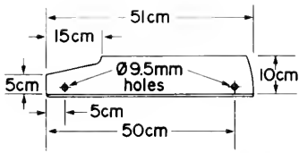
L. WING - SIDE ELEVATION
