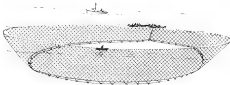
Menhaden purse seine
