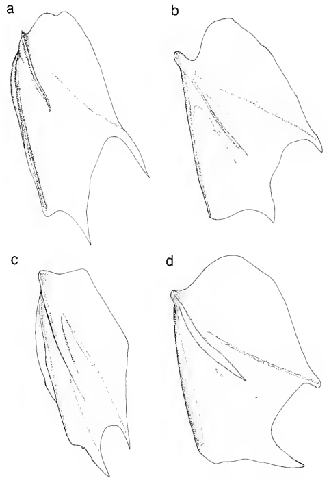
Fig. 5. Opercular bones of some Bathylagus species: a) antarcticus ; b) gracilis ; c) tenuis ; d) pacificus
