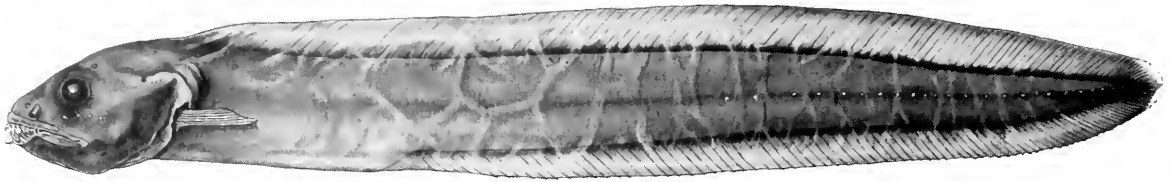
Fig. 11. Lycodapus antarcticus MNHN 1984-761, 184 mm SL, Kerguelen Plateau
