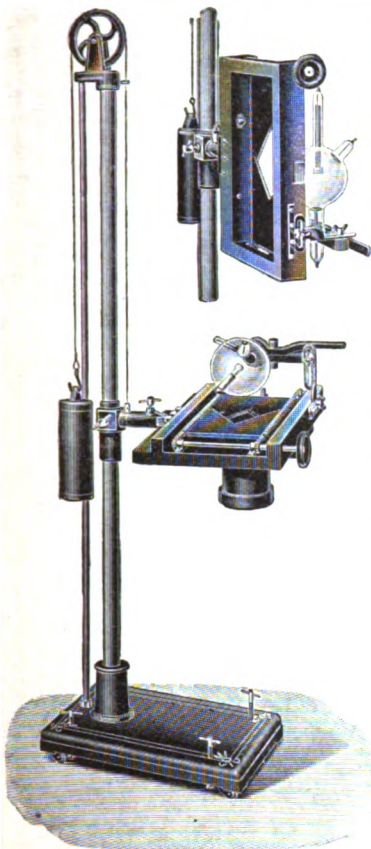
Blendenstativ.
