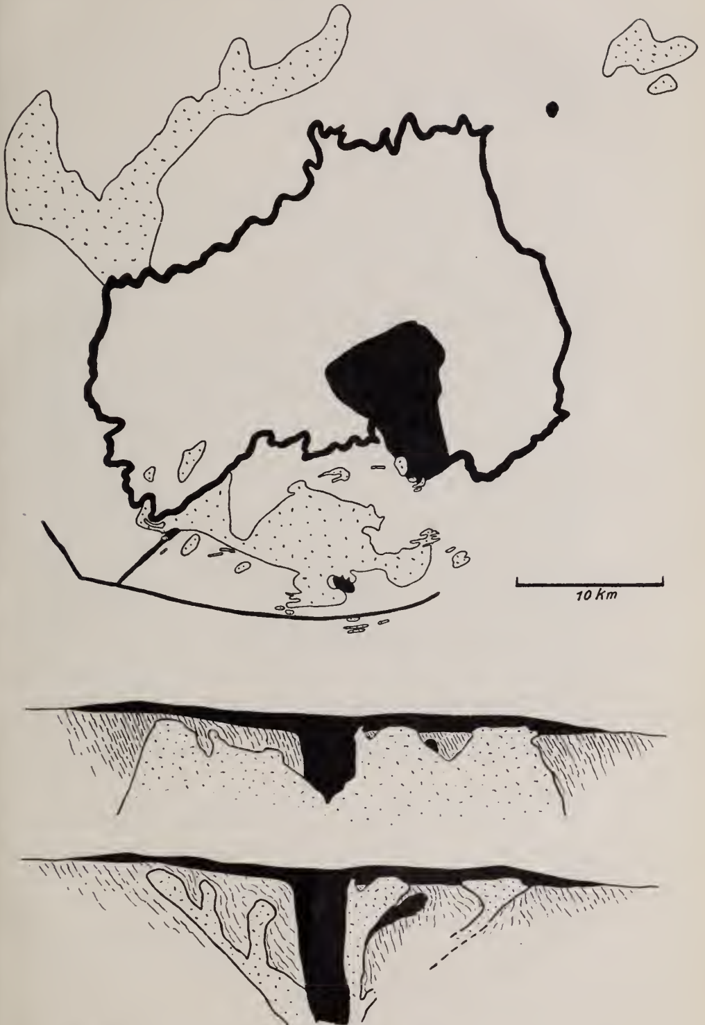
Figur 19. Karte und Profile des Erongogebirges im Hererolande
