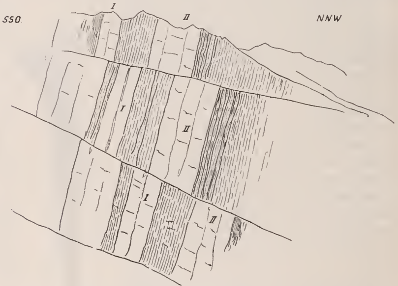
Fig. 13. Flache, diskordante Verschiebungsklüfte in steilstehenden Schichten. Bhf. Eisenbrod in Böhmen.
