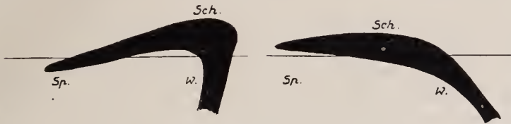
Fig. 17. Brockenmassiv (links) und Bayrische Massive (rechts) in Beziehung zu späteren Hebungen und zum Aufschlußniveau.
