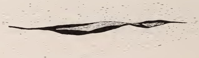
Fig. 22. Granit (schwarz) schält eine Gneisscholle aus ihrer Einbettung von (gestrecktem) Diorit. Röhrnbach im Passauer Wald (E. Cloos. 1922).
