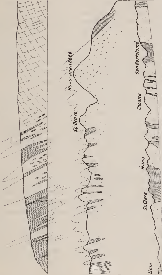
Fig. 24. Acht Profile durch konkordante Massive in gefaltetem Gebirge. — 1—3. Syenitmassiv von Nimptsch in Schlessien (nach H. Cloos, 1922). — 4 und 5. Syenitmassiv der Serra de Monchique in Portugal (nach E. Kaiser, 1914). — 6. Kontakt des mittelböhmisches Granitmassivs mit dem Algonkium am rechten Sazawauer (nach M. Kettner). — 7 und 8. Höheres und tieferes Profil durch die südamerikanische Cordillere, punktiert Granodiorit (nach G. Steinmann, 1910).
