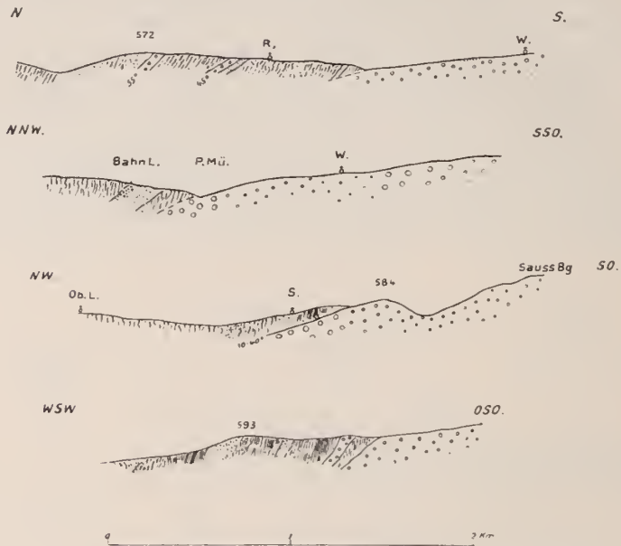
Fig. 11. Vier Profile durch das nördliche Hauenberger Massiv (nach E. Cloos).
