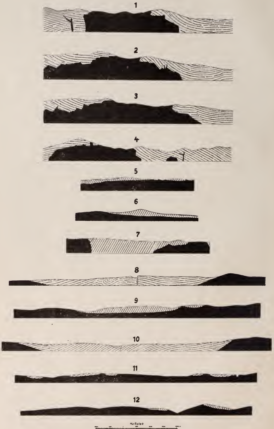
Figur 1. Zwölf Querschnitte durch Batholithen
