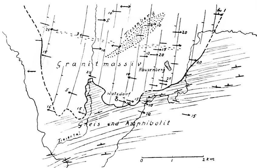
Fig. 9. Strukturkärtchen des südl. Hauzenberger Granitmassivs. Punktiert: feinkörniger Granit. Weiß: mittel- und grobkörniger Granit. Südlich davon die Gneisunterlage. Pfeile bezeichnen das Streichen und Fallen der linearen Streckung. Senkrecht darauf streichen und fallen die Q-Klüfte (nach der Kartierung des Verfassers).
