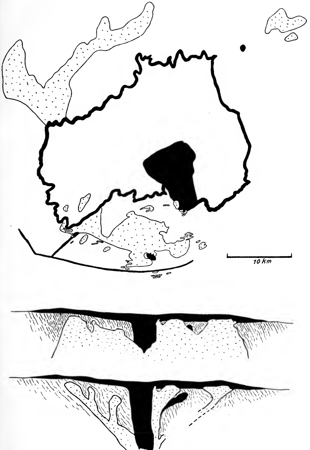
Figur 19. Karte und Profile des Eronggebirges im Hererolande
