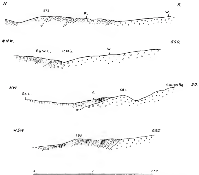
Fig. 11. Vier Profile durch das nördliche Hauzenberger Massiv (nach E. Cloos).
