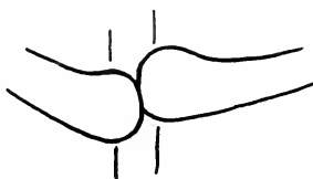
FIG. 592. Ptilophyllum pecten . (Manchester Museum, Williamson Coll. 3726.)
