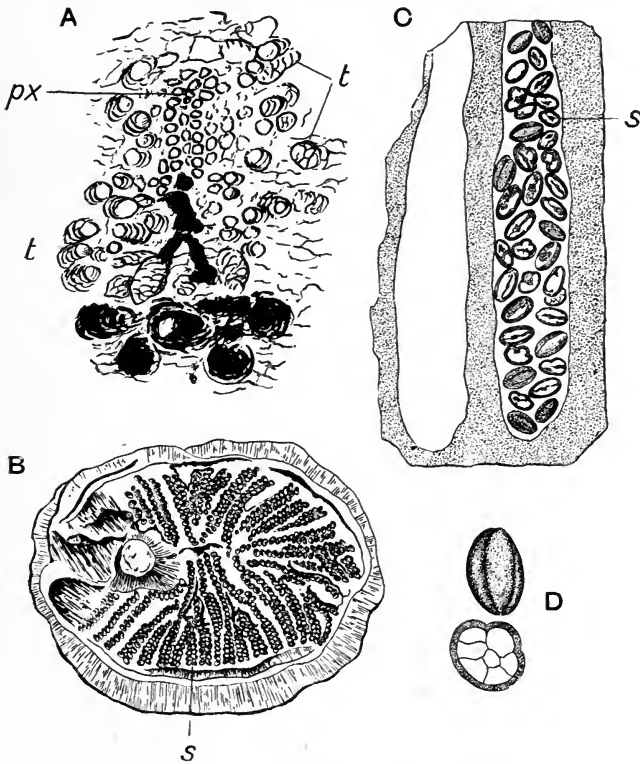
FIG. 432. A. Dolerophyllum Goeperti , section of vein. B. Dolerophyllum Berthieri ; s, microspores. C. Dolerophyllum fertile . D. Dolerophyllum fertile , microspores. (After Renault.)
