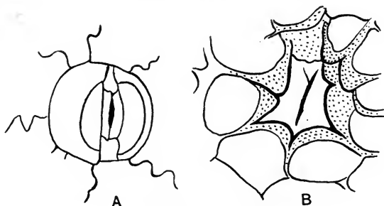
FIG. 611. A, Pterophyllum Nilssoni ; B, Nilssonia mediana . (After Thomas and Bancroft.)
