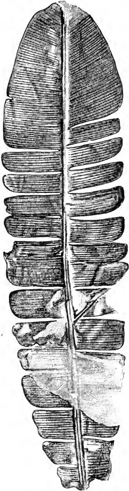
FIG. 615. Pterophyllum ( Anomozamites ) Nilssoni . (British Museum, 39,306; nat. size.)
