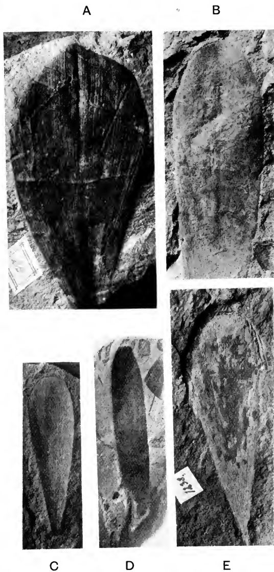
FIG. 469. A—C, E, Cordaites aequalis ; D, Cordaites Clerci . (After Zalessky; \frac{5}{8} nat. size.)
