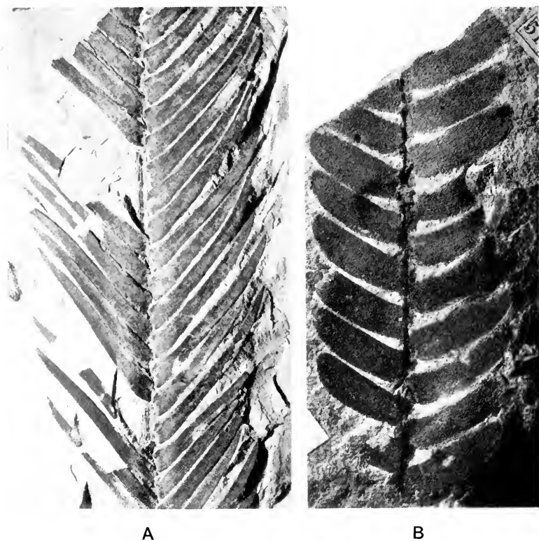
FIG. 603. A, Otozamites Goepertianus . B, Otozamites obtusus (= O. Bechei ); type-specimen. (A, British Museum, V. 2360; B, Oxford Museum.)
