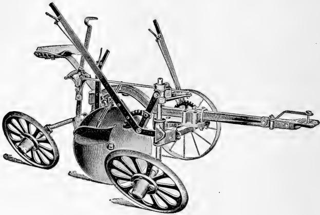
FIG. 78. Disk sulky plow.
