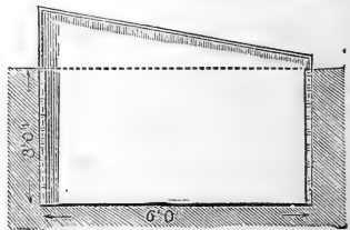
Fig. 46.—SUNKEN PIT.
