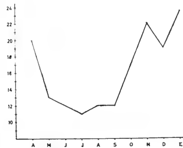
FIG. 7. LAGUNA LO MENDEZ, TEMPERATURA SUPERFICIAL DEL AGUA.
