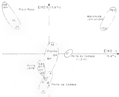
Figura 11. Análise fatorial de correspondências sobre os dados de recobrimento: projeção dos relevés no plano fatorial I-II (vide código dos relevés no parágrafo “metodo logia”).
