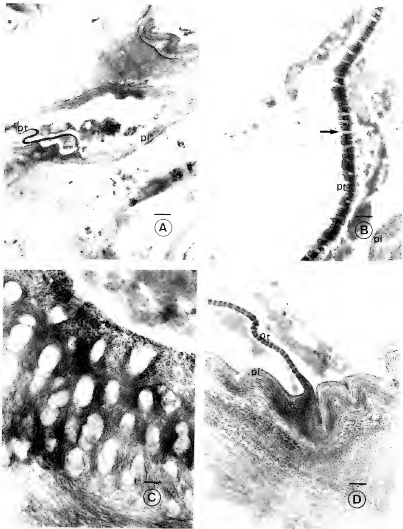
Fig. 3. Fotomicrografía de elementos cribados en Lessonia nigrescens . A: Elementos cribados del tejido medular del estipe. Se observa una gruesa pared lateral (lpl) y la pared transversal (pt) X 9400. B: Pared transversal (pt) presenta poros (flecha) X 15500. Escala = 0.5 \mu m. C: Corte oblicuo de la pared transversal. Se observan poros X 88000. Escala = 0.09 \mu m. D: Pared lateral (lpl) formada por microfibras orientadas en forma paralela X 27200. Escala = 0.29 \mu m.
