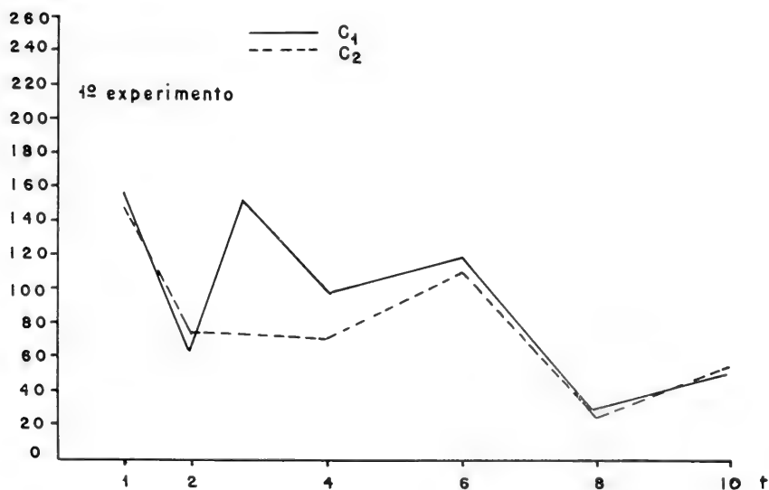
Fig. 6. Teor médio de clorofila-a (mg/m 3 ) de Tetraselmis chuii nos diversos meios.
