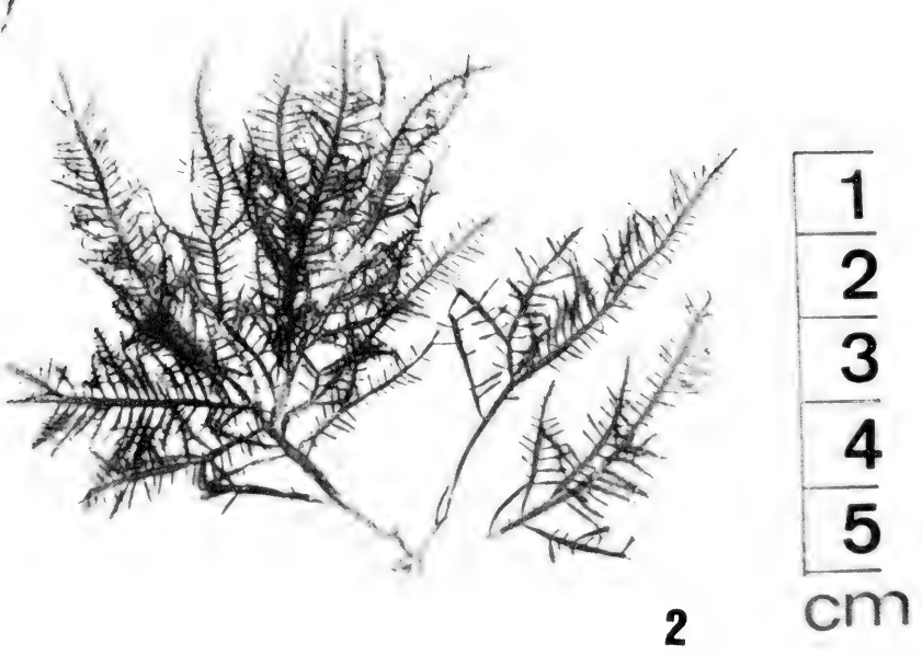
Fig. 2. Gelidium coarctatum .
