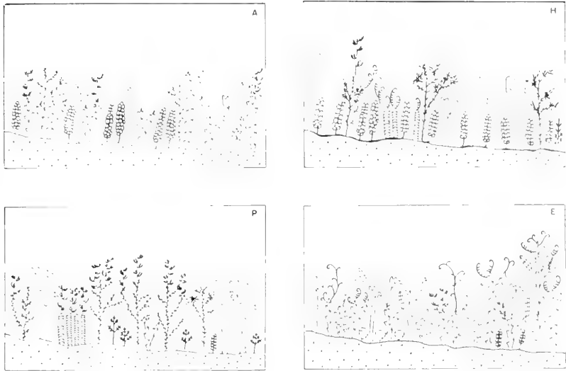
Figura 6.- Relevê fitosociológico da estação 14 (Praia Rasa). Representação esquemática das populações com espécies do minantes, nas 4 estações do ano (A - outono, H - inverno, P - primavera e E - verão)
