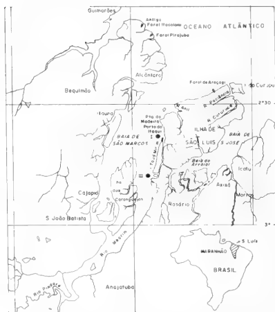
Fig. 1.- Localização das estações do microfítocoplâncton. (Est. I e Est. III), na Baía de São Marcos, São Luís, Maranhão - Brasil.
