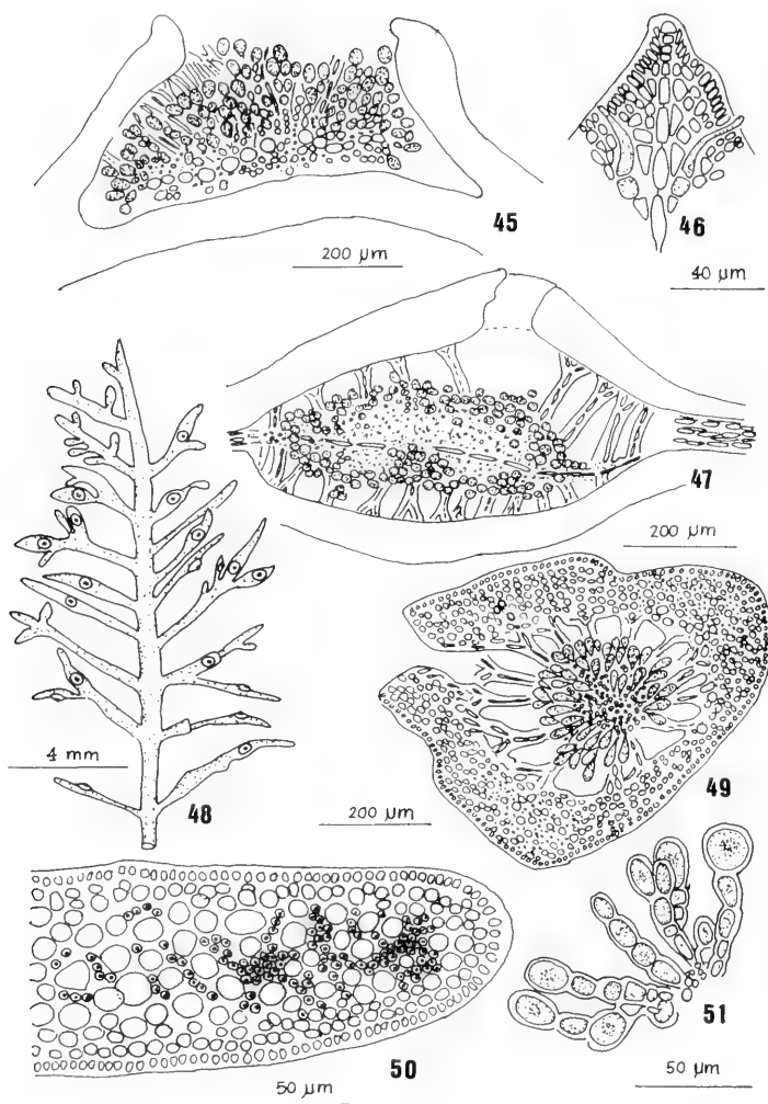
Figs. 45-51. Pterocladia capillacea (Gmelin) Bornet et Thuret. 45. Corte longitudinal de um cistocarpo, mostrando carposporos formados em série; desenho esquemático. 46. Corte longitudinal de um ápice fértil, mostrando a organização do talo e os carposônios. 47. Desenho esquemático de um cistocarpo em corte longitudinal. 48. Ramo com cistocarpos. 49. Corte transversal de um cistocarpo. 50. Corte transversal de um ramo; margem do corte. 51. Detalhe do carposporófito. Figs. 45-48 e 50 - Guarapari, ES (SPF 9079). Figuras 49 e 51 - Praia dos Fornos, Cabo Frio, RJ (SPF 2157).
