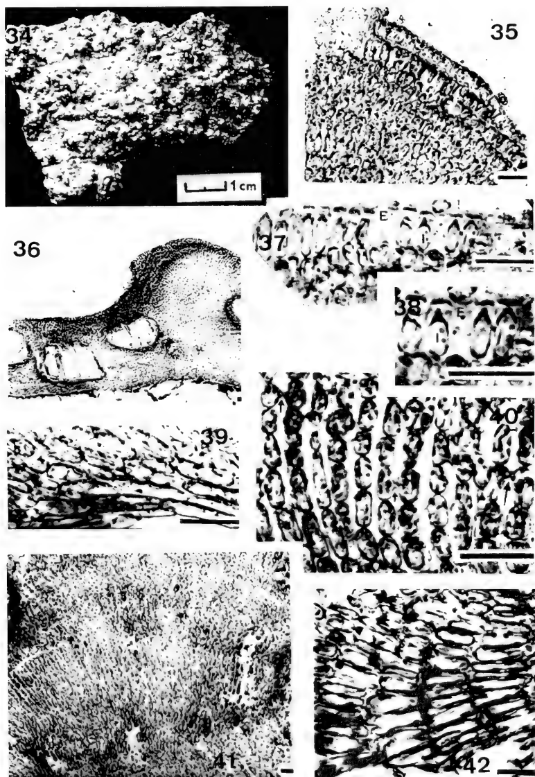
Fig. 34. Lithothamnion granuliferum Fosl.; Argentina, Tierra del Fuego, Coll. Mendoza N° 18705, 25-2-1987. Fig. 35. Porción lateral de una excrescencia. Fig. 36. Corte longitudinal radial del talo basal y excrescencia mostrando la disposición de los conceptáculos asexuales. Fig. 37 y 38. I) células iniciales peritállicas; E) epitalo. Fig. 39. Hipotalo de estructura simple. Fig. 40. Células de una excrescencia mostrando las fusiones. Fig. 41. Porción basal de una excrescencia. Fig. 42. Falso hipotalo coaxial. Escala de micrones: 20, \mu m.
