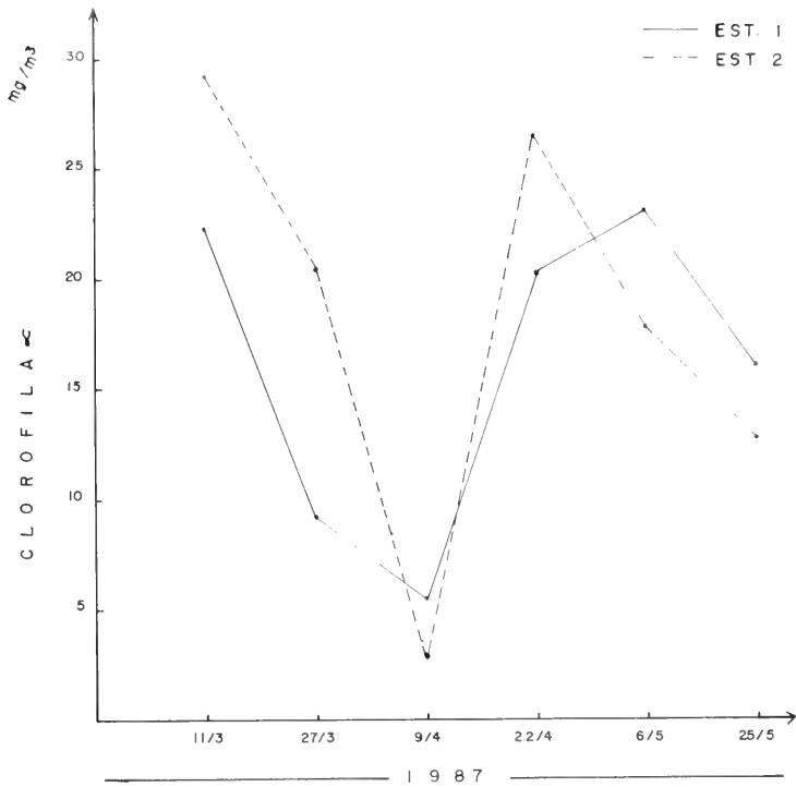
Fig. 3. Variação do conteúdo de clorofila α do viveiro 3.
