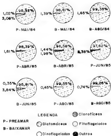
Fig. 3. Abundância relativa dos principais grupos, de microfiteoplâncton, estação III, na baía de São Marcos (São Luis-MA) em campanhas realizadas durante os anos de 1984 e 1985
