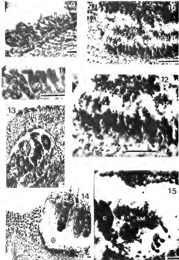
Fig. 9. Lithothamnion heterocladum Fosl. Carposporofito maduro; A) células auxiliares; B) célula de fusión; C) filamento del gonimoblasto; D) resto de las ramas carposporogonales. Figs. 10 y 13. Espermatangios maduros; S) disposición de los espermatangios en forma dendroide; SM) masa de espermacios. Fig. 11. Formación de carposporogonios iniciales. Fig. 12. Conceptáculo carposporofítico maduro. Fig. 14. Conceptáculo tetraspórico maduro; T) tetrasporangios; →poro de salida. Fig. 15. Conceptáculos hermafroditas. Escala de micrones: 20 \mu m.
