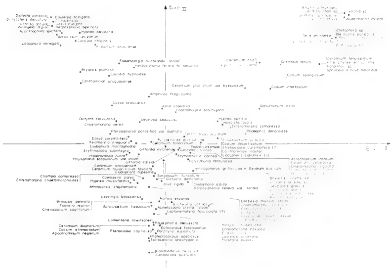
Figura 12. Análise fatorial das correspondências sobre dados de recobrimento. Projeção das espécies no plano fatorial I-II.
