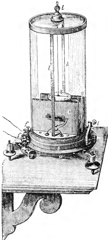
FIG. 37. A MULTIPLIER.
