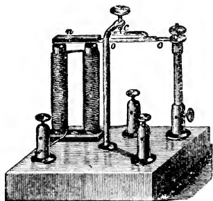
FIG. 12. WAGNER'S HAMMER.
