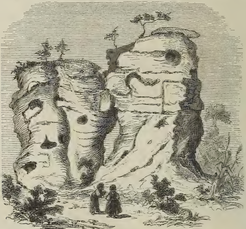
Fig. 114. Felsenruinen an den Tysaer Wänden.
