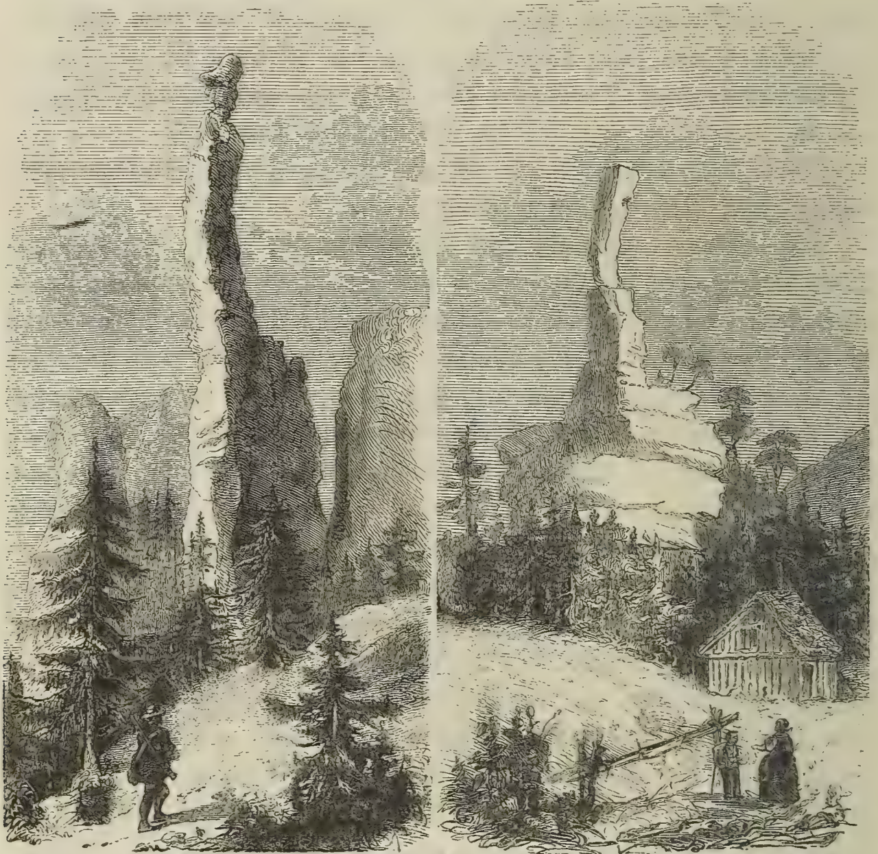
Fig. 111. Felsenfäule am Pfaffenstein. Fig. 112. Die Kazentirche im Thale von Dittersbach.
