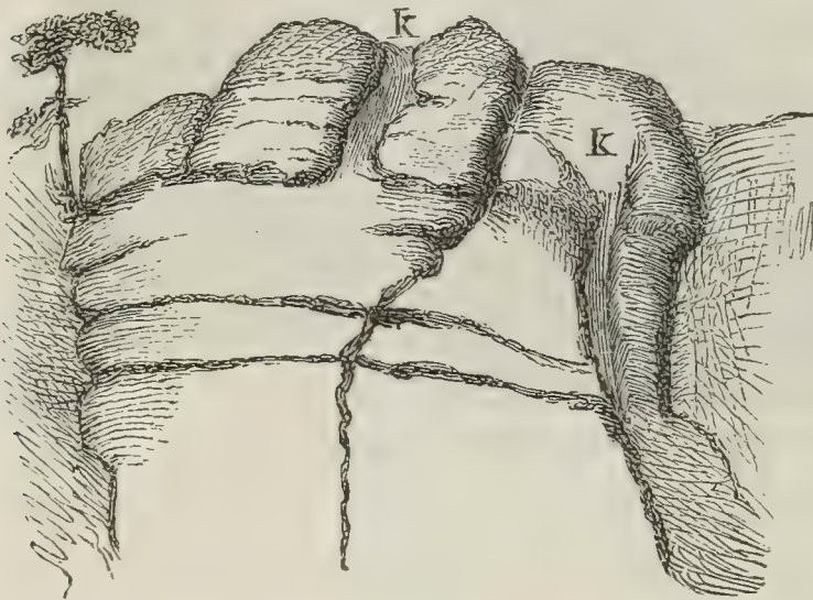
Fig. 70. Felsmasse mit Kanälen k k an den Seitenwänden; am obern Ende des Wurzelweges nach den Winterbergen.
