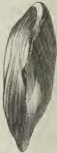
Fig. 29. 30. Lima multicosata . Geinitz. Königstein.
