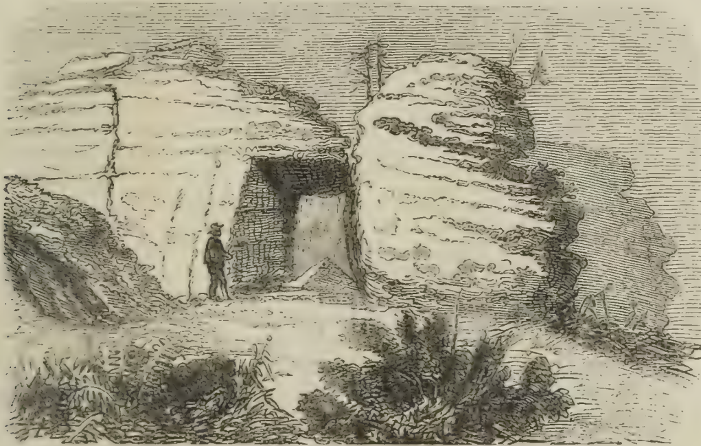
Fig. 118. Wildpretstammer in den Nickelisdorfer Wänden.
