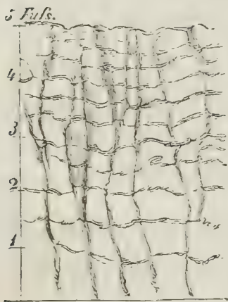
Fig. 55. Zerklüftung des Sandsteins in Loosdorf.
