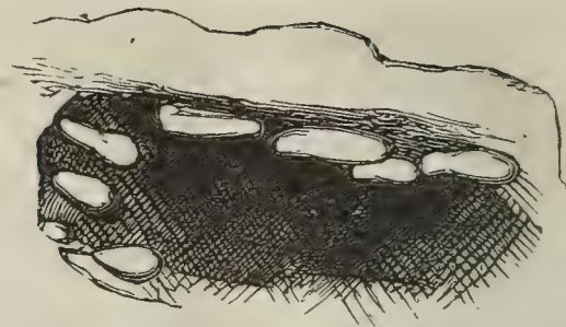
Fig. 10. Sandsteinfragment, worin eine Höhlung mit Kohlenpulver. Bohrlochausfüllungen zusammengedrückt.
