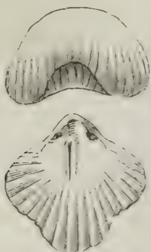
Fig. 7. Terebratula plicatilis . Sowerby. Königstein.
