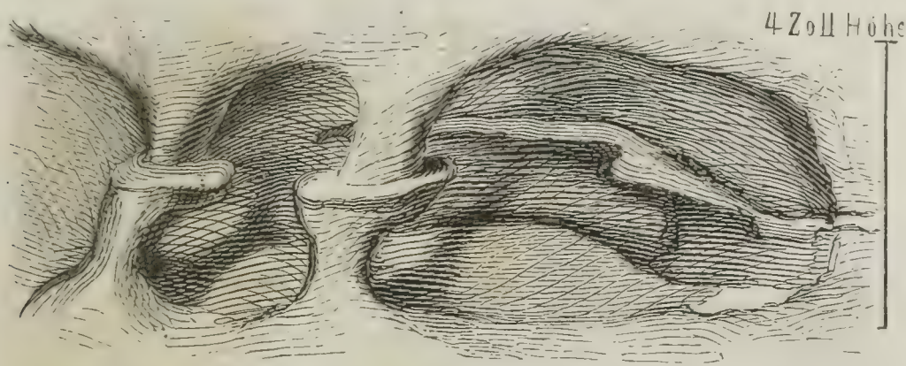
Fig. 103. Höhlenbildung zwischen dem Teufels- und Schlüsselgrunde.
