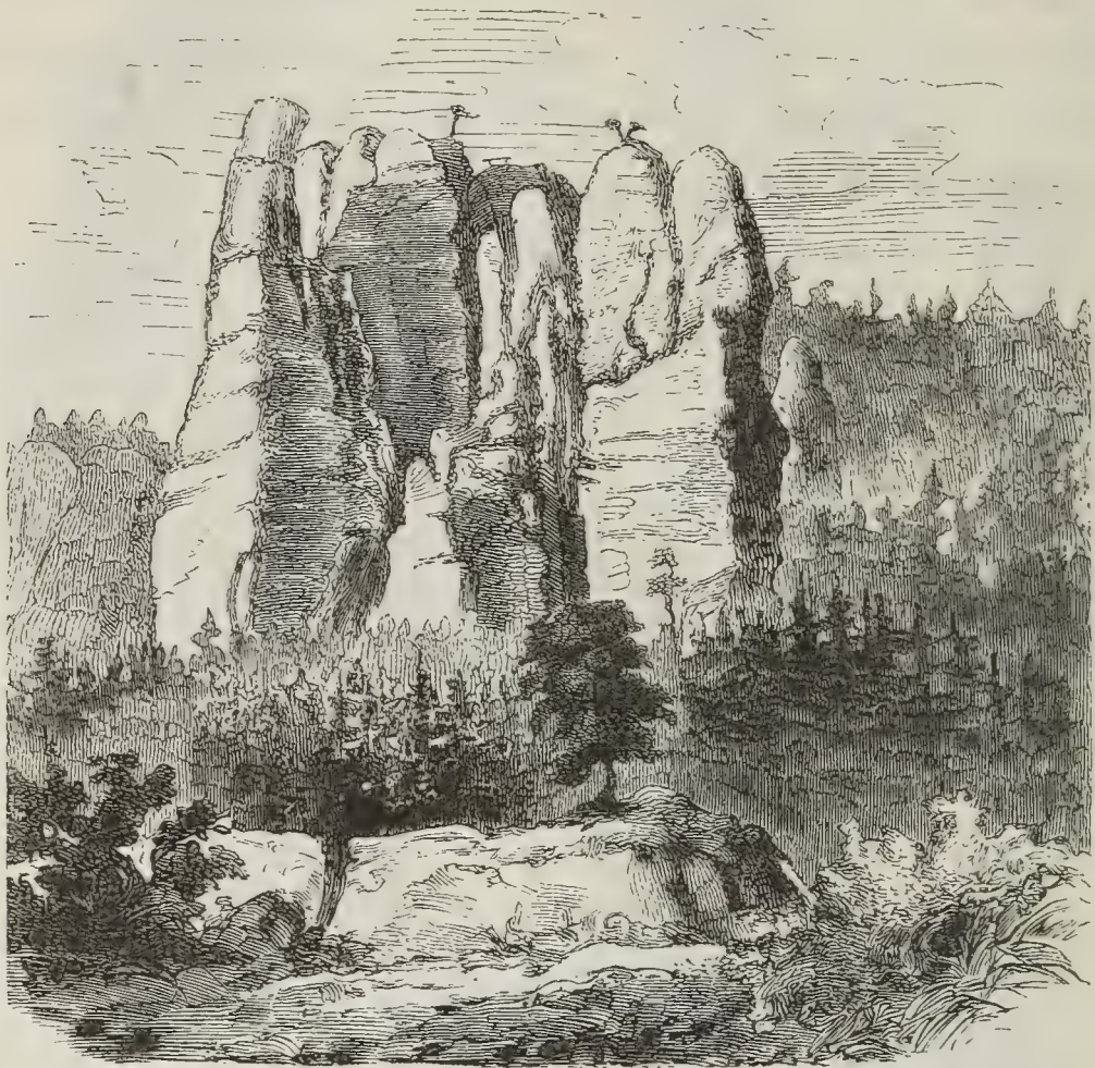
Fig. 42. Der Ferdinandsstein nördlich der Bastei, nach Bürger.
