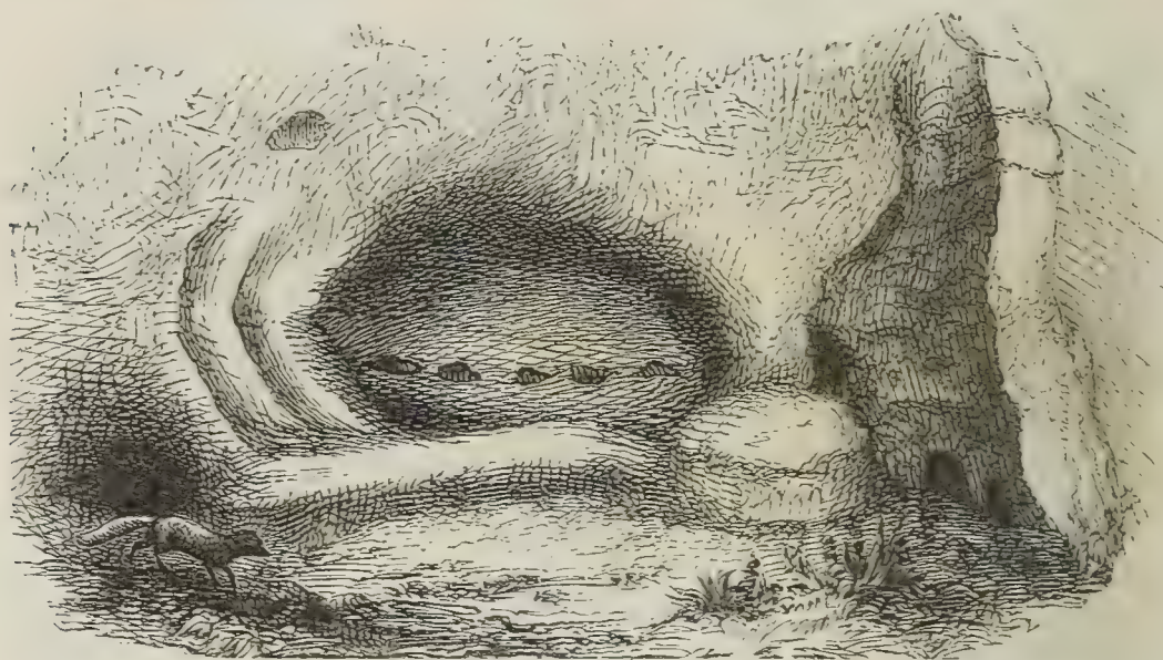
Fig. 105. Nische und Ruhebank am Quirl.
