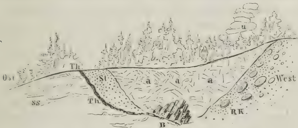
Fig. 52. Durchschnitt des Basaltausbruchs am Gorischstein: S. S. Sandstein, zum Theil säulenförmig. Th. Thoneisenstein. St. Steinmark. a. a. a. Aufgelöster Basalt. B. Fester Basalt. R. K. Reibungskonglomerat von Steinmark mit Ballen von Sandstein. w. Weg. u. Ungeförte Felsmasse.
