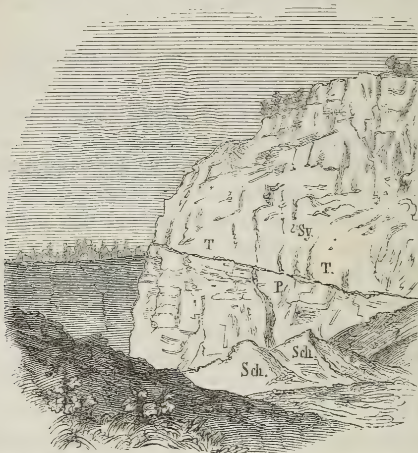
Fig. 56. Steinbruch bei Weinböhl, frei nach Caru: Sy. Syenit. T. Thon- und Mergelschicht. P. Plänerkalkstein. Sch. Schutt.
