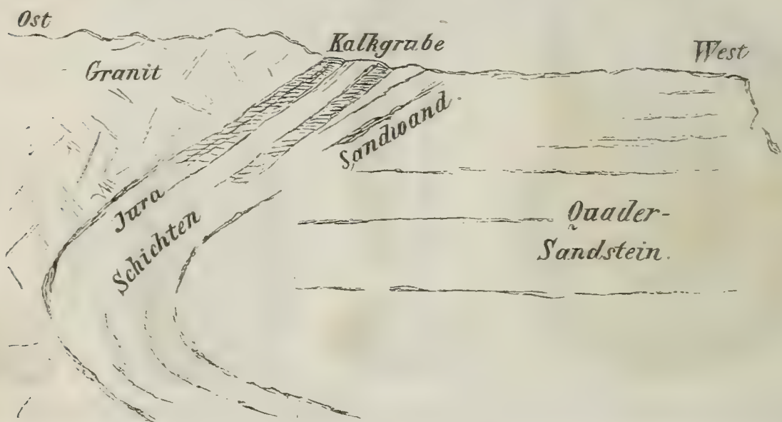
Fig. 62. Ideales Profil der Grenzverhältnisse bei Hohnstein, nach Cotta.
