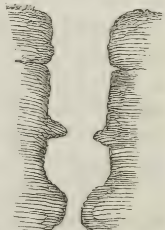
Fig. 74. Spalte gleichmäßig ausgewaschen.
