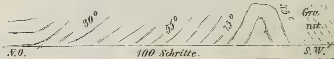
Fig. 65. Schichtung des Pläners bei Niederwartha, ideal nach Naumann.
