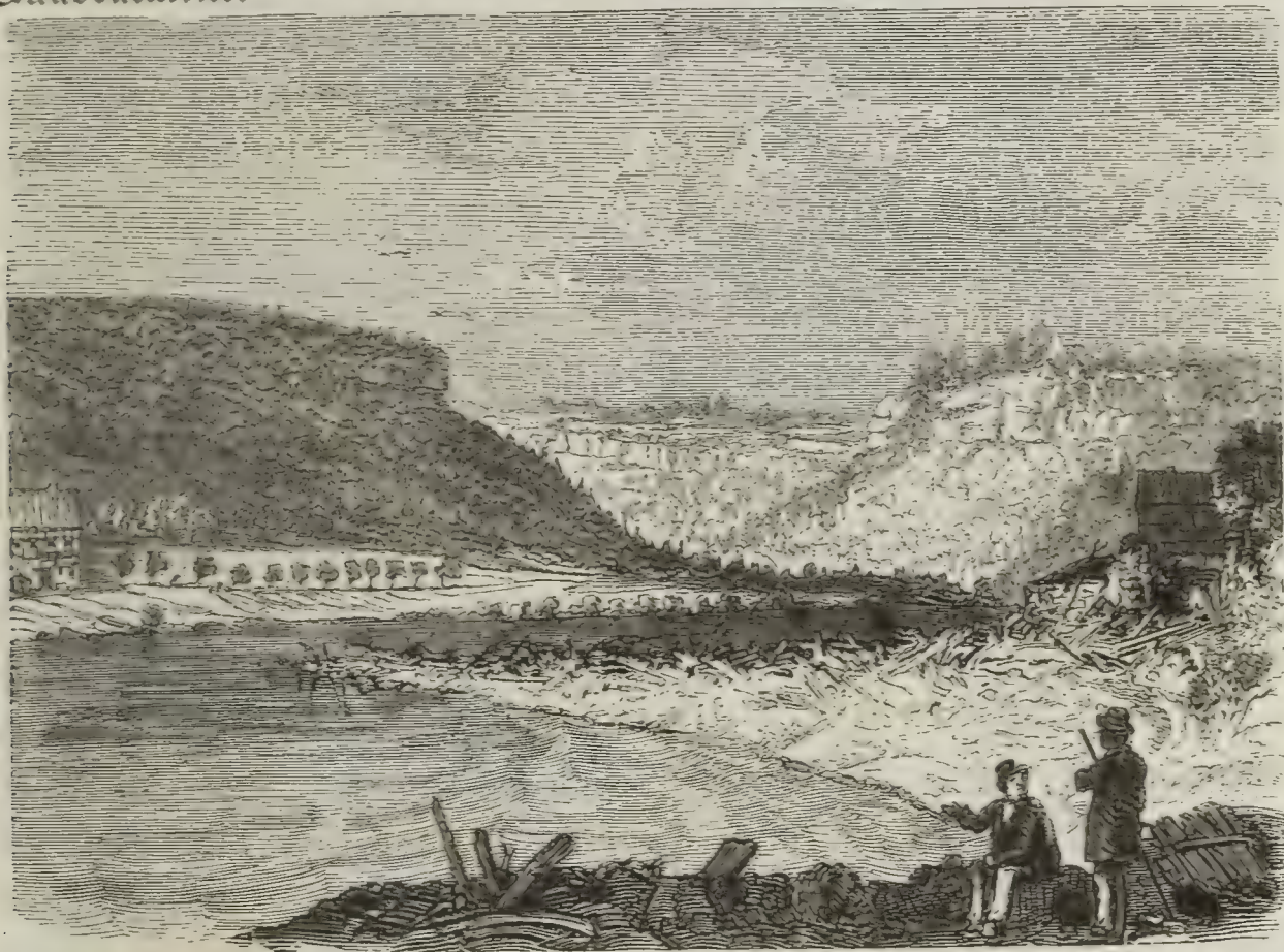
Fig. 97. Schuttmasse am Ausflusse des Ottewalder Baches in die Elbe bei Wehlen, nach dem Wolkenbruche vom 1. Sept. 1822.
