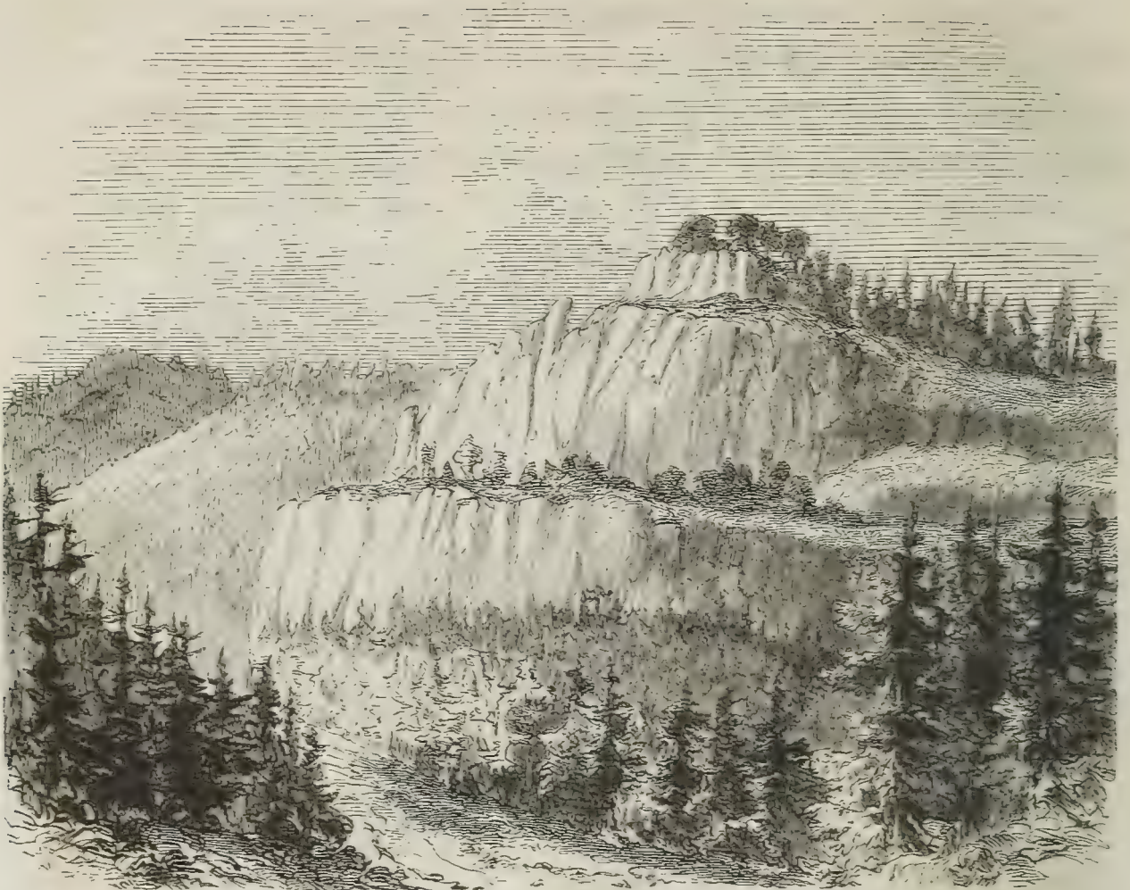
Fig. 78. Felsterrassen des Teichsteins, aus dem großen Fischand gesehen.
