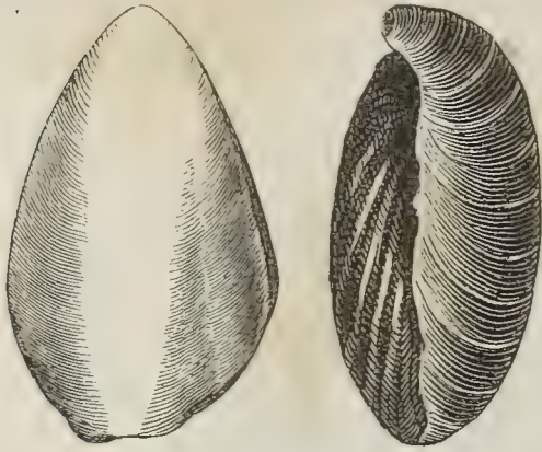
Fig. 18. Terebratula nerviensis . d'Archiac. Grünsand. Tunnel.
