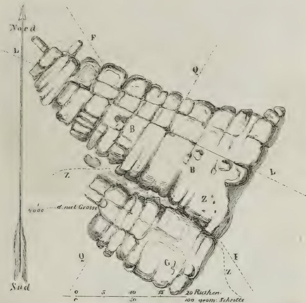
Fig. 43. Grundriß der Felsplatte des Gorischsteins: Z Zugang. G Gipfel. B vorstehende Blöcke. L Längenabsonderung, auf den Königstein treffend. Q Querabsonderung. F Fallrichtung der Schichten. \frac{1}{4000} d. nat. Grösse.
