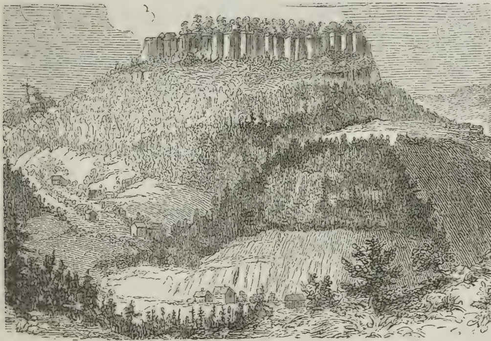
Fig. 47. Königstein, Südostseite, von Einsiedel bei Pfaffendorf gesehen.
