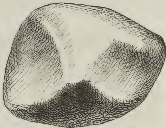
Fig. 85. Geschiebe, vierseitig abgeschliffen.
