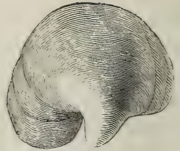
Fig. 28. Exogyra columba . Sowerby.
