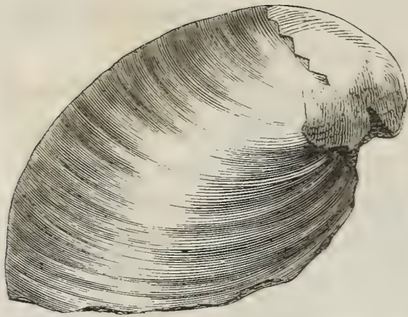
Fig. 27. Id. Steinfarn mit der Schale. Postelberg. Böhmen.
