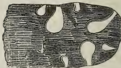
Fig. 11. Treibholzfragment, verkohlt, mit Bohrlochern von Pholas Scelerodites. Geinitz. Raundorf.
