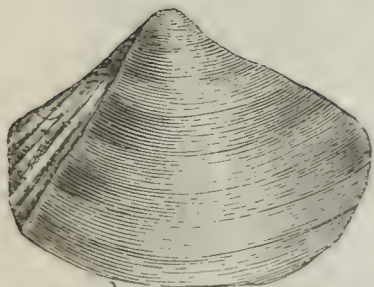
Fig. 6. Protocardia Hillana . Sowerby. Tyssa. Königstein.
