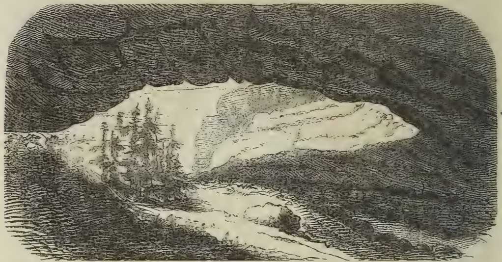
Fig. 108. Die große Hicfelshöhle in einer Seitenschlucht des großen Zschand.
