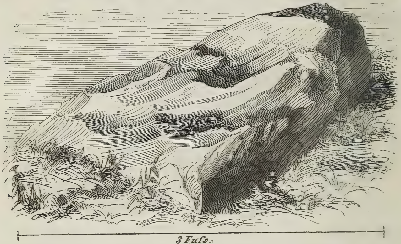
Fig. 87. Erratischer Block westlich der Meridiansäule bei Rähmig.
