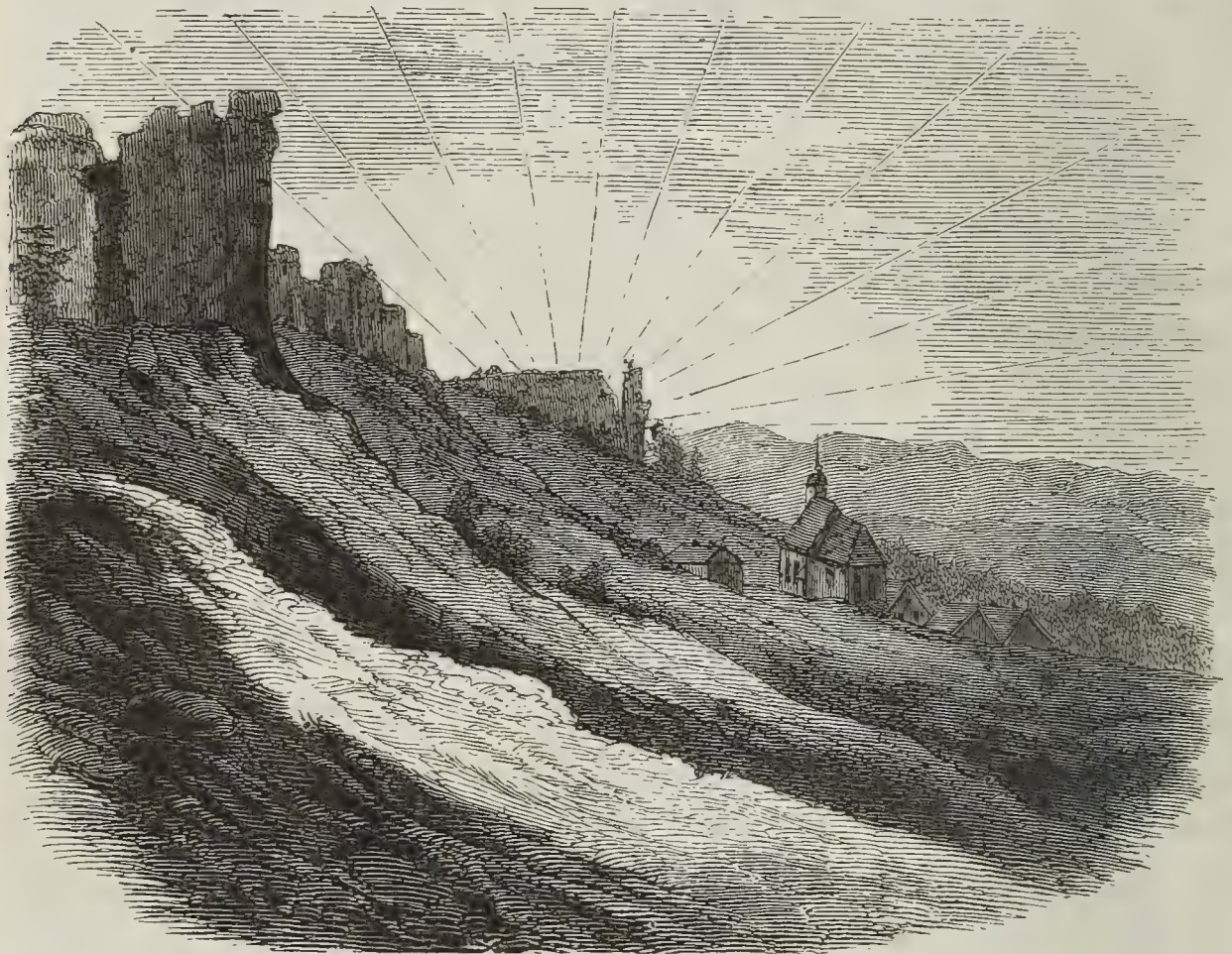
Fig. 36. Abfall von den Tyssaer Wänden nach Süden.
