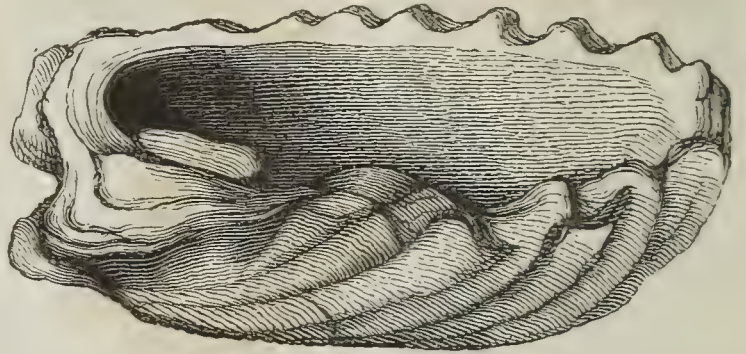
Fig. 19. Ostrea diluviana . Linné. Untere Schale. Unterer Pläner. Plauen.
