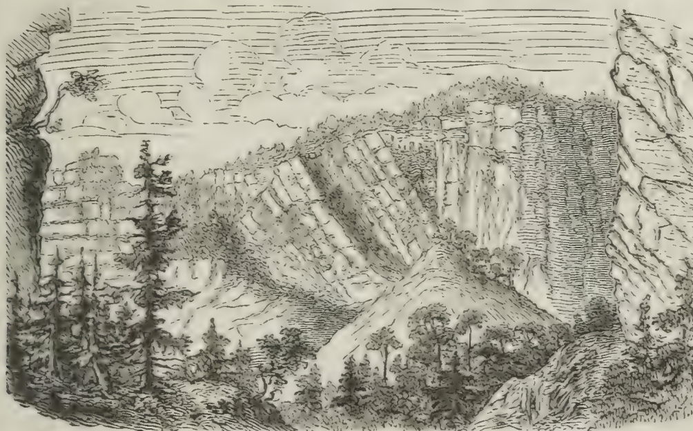
Fig. 49. Südwestseite des Naundorfer — nördlichen — Bärensteins, gesehen vom Thürmsdorfer Bärenstein, schräge Zerklüftung.
