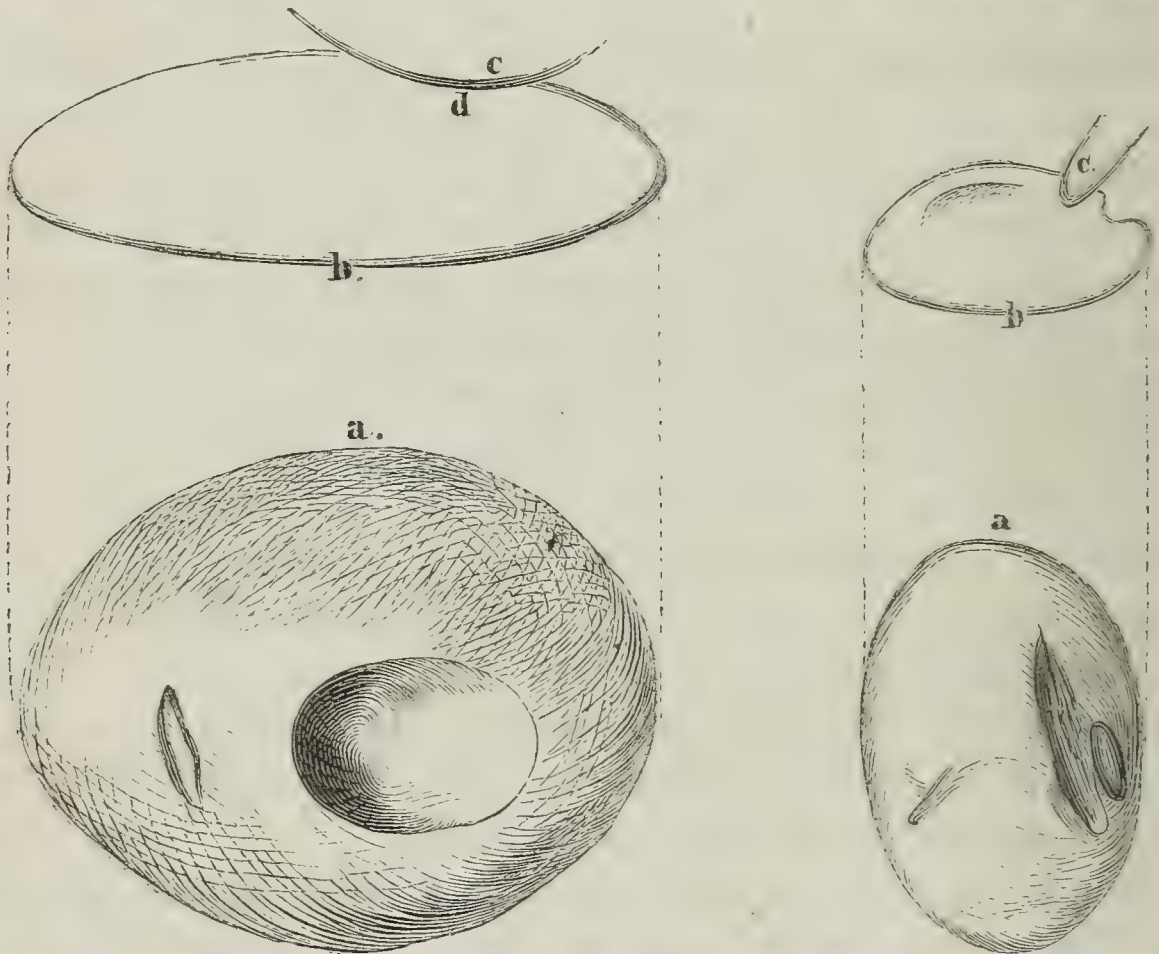
Fig. 81. Erratische Geschiebe mit flacher Aushöhlung. Fig. 82. Erratische Geschiebe mit tiefer Rinne.
