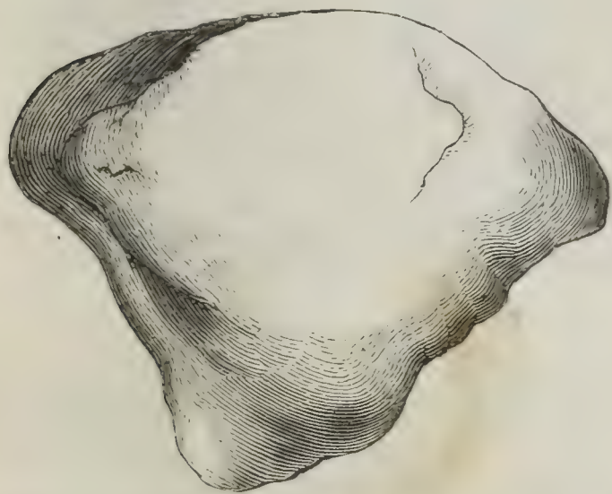
Fig. 25. Exogyra columba . Sowerby. Steinfern im Gestein, mit der Höhlung für den Wirbel. Königstein und überall.
