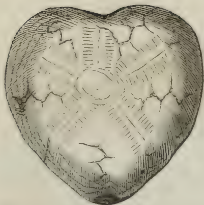
Fig. 5. Spatangus cor anguinum . Lamarck. (Seeigel.)
