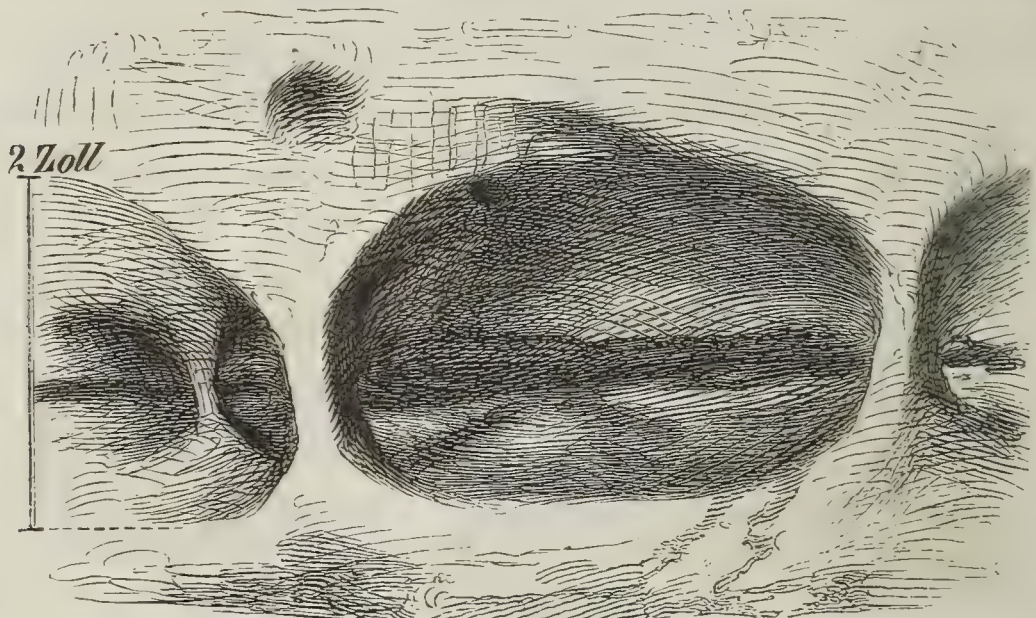
Fig. 102. Bildung der kleinsten Höhlen.
