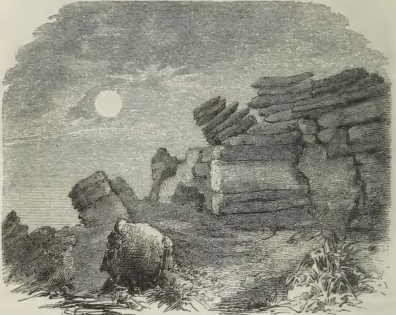
Fig. 76. Klippen an den Nickelsdorfer Wänden.
