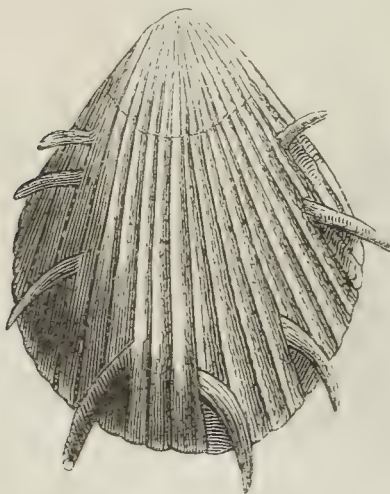
Fig. 23. Spondylus spinosus . Sowerby. Plänerkalk. Strehlen.
