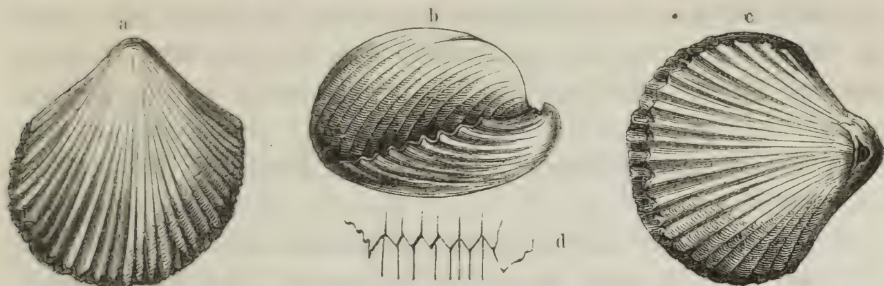
Fig. 57. Juraversteinerungen von Hohnstein und Beschnig. Terebratula lacunosa . Colonia.
