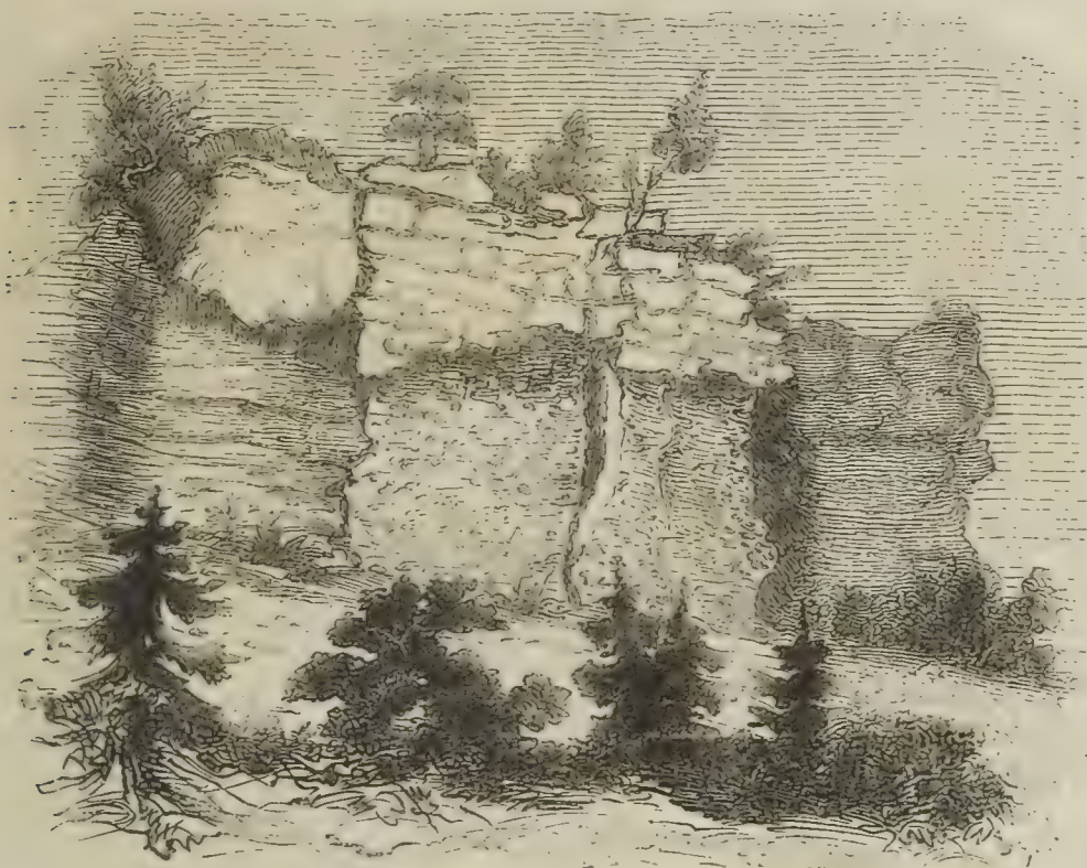
Fig. 109. Wand mit Verwitterung bei Rosenthal.
