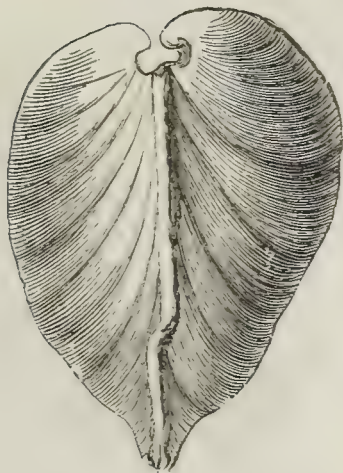
Fig. 31. 32. Inoceramus striatus . Mantell. Königstein und überall.
