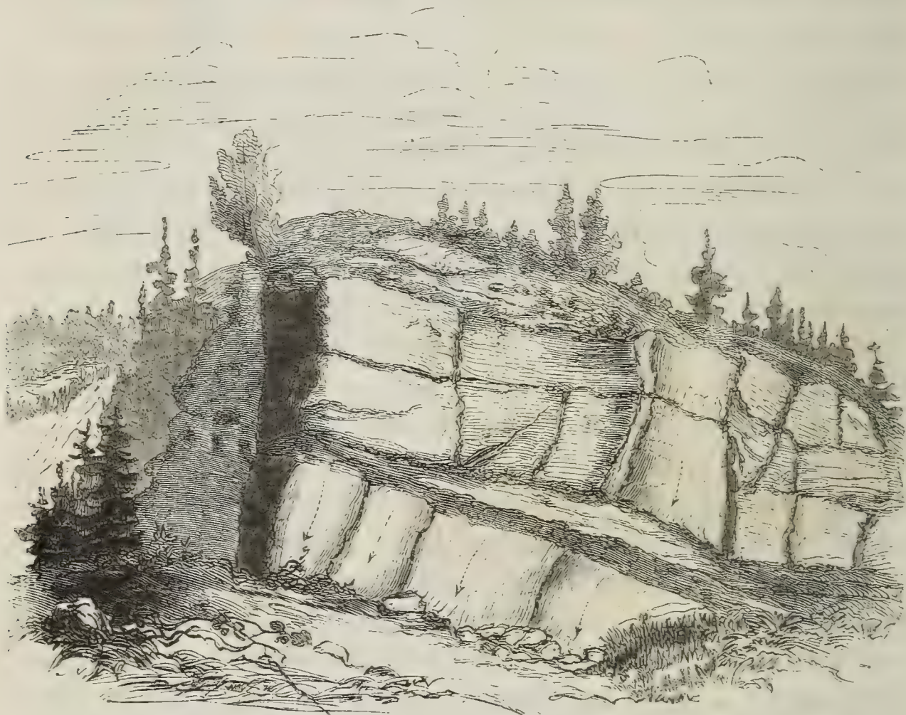
Fig. 63. Felswand am Kirnitzschberge. — Senkrecht abblätternder Sandstein.
