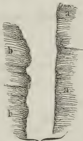
Fig. 73. Spalte einseitig ausgewaschen.
