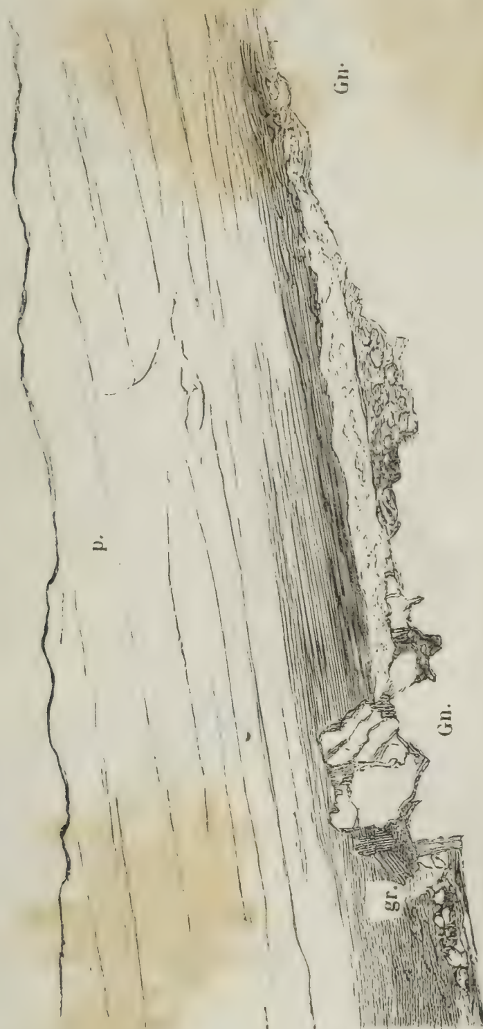
Fig. 17. Einziger Meeresgrund am Westende des Tunnels bei Dherau. Gn. Gneis. gr. Grünsand mit einer Geröllschicht aus Gneis und Granit. p. Unterer Pläner — frei nach Geinitz.
