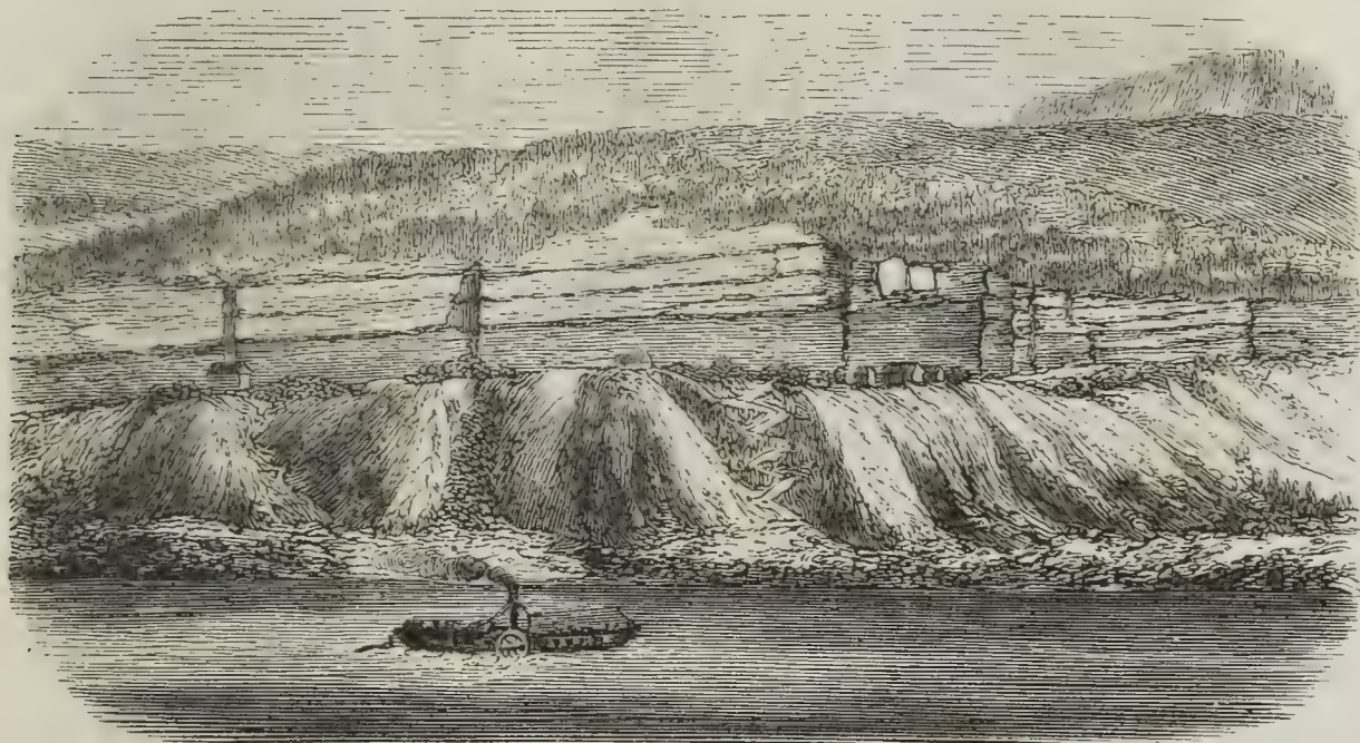
Fig. 33. Die Schulhahn-Steinbrüche von Südwest. (Flachgeneigte Bänke.)
