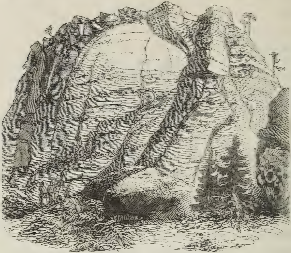
Fig. 39. In Richter's Schlüchten, sphäroidische Absonderung.
