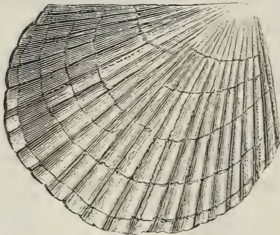
Fig. 29. 30. Lima multicosata . Geinitz. Königstein.
