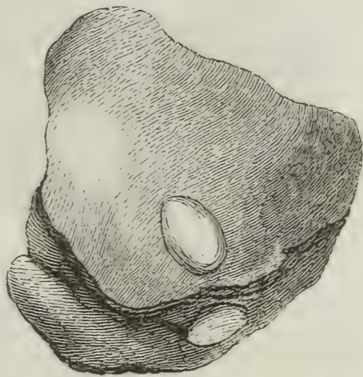
Fig. 26. Id. Steinfern mit der flachen Klappe oben, und den Reliefs der Muskeleindrücke. Königstein und überall.
