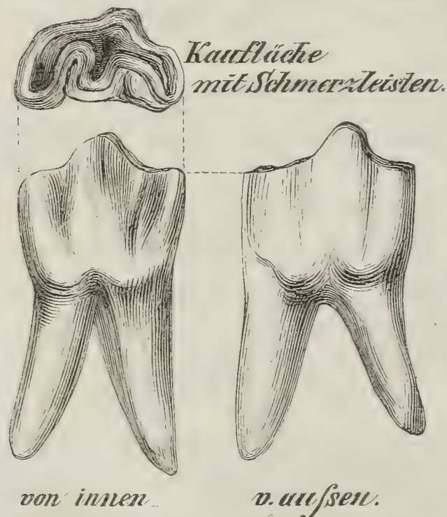
Fig. 89. Backenzähne aus dem Unterkiefer des Rhinoceros tichorhinus .
