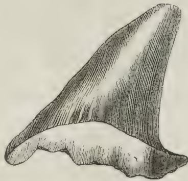
Fig. 21. Oxyrhina mantellii . Agassiz. (Haifischzahn.) Plänerkalk. Strehlen.
