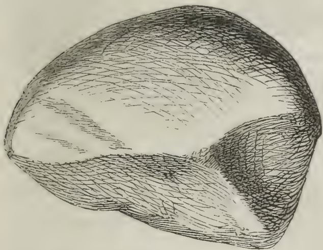
Fig. 84. Geschiebe, dreiseitig abgeschliffen.
