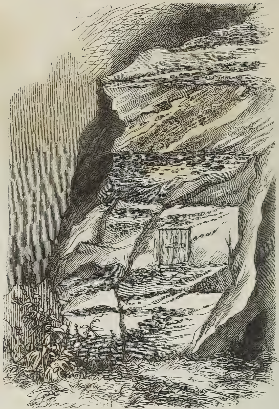
Fig. 16 Bei Herniskretschken (Schräge Schichten in den wagrechten Bänken.)
