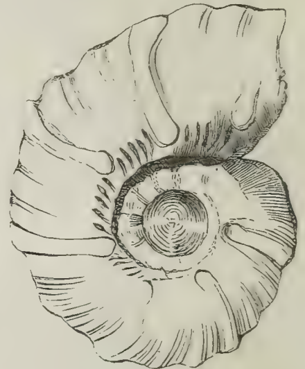
Fig. 22. Ammonites peramplus . Sowerby. Plänerkalk. Strehlen.
