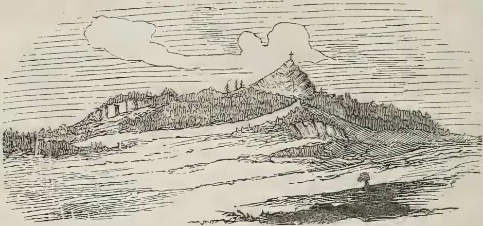
Fig. 50. Der Schönwalder Spizberg von Norden gesehen.
