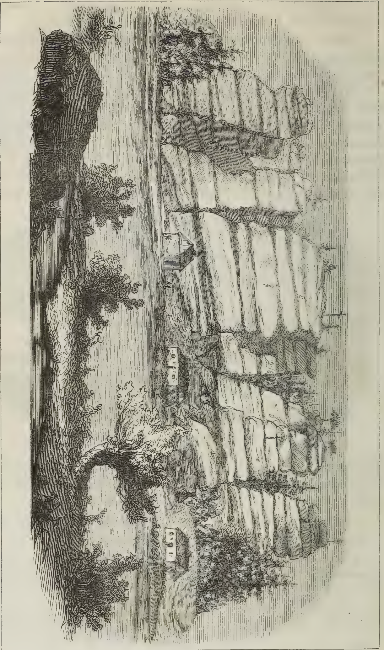
Fig. 34. Der Strenberg im Silaer Grunde. (Blachgenigte Bänke.)
